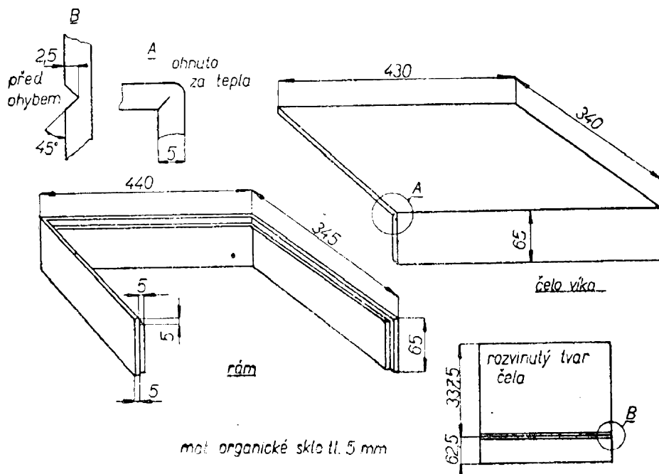
Obr. 31. Křít gramofonového šasi – druhý způsob řešení
