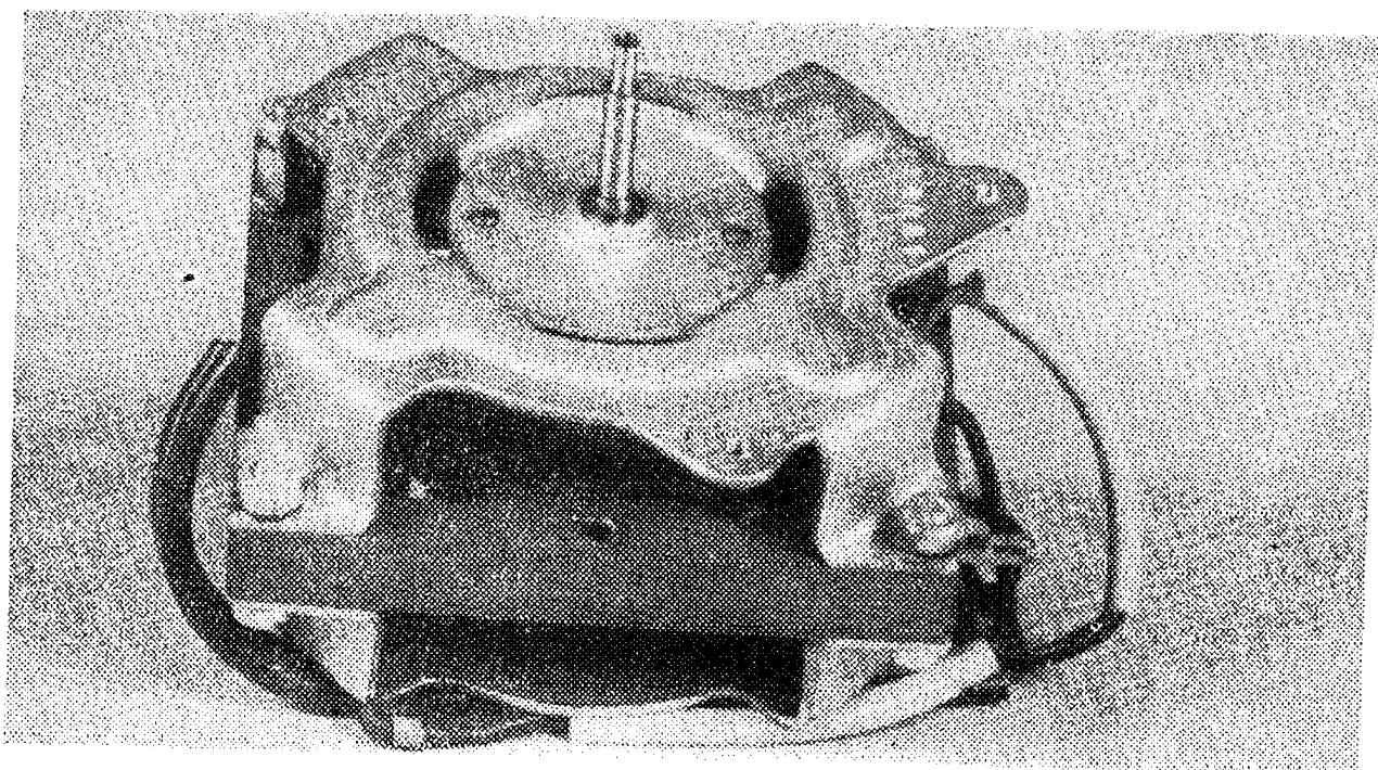
• Motorek MT6
