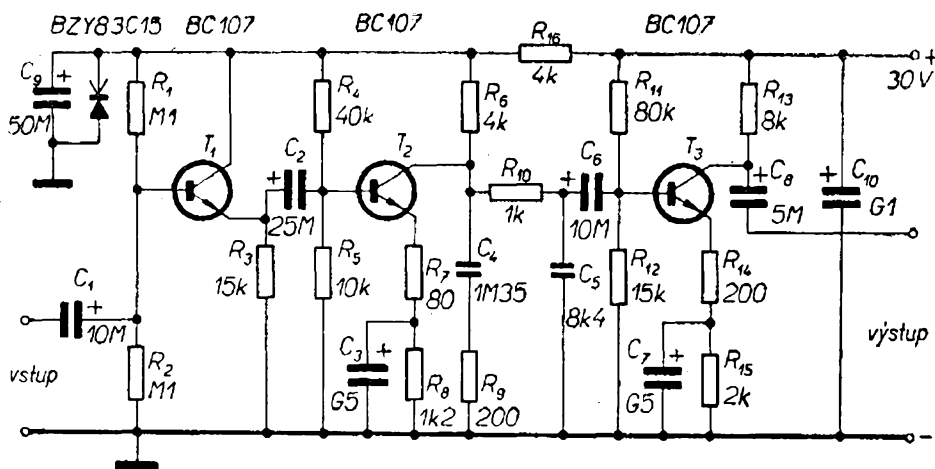
Obr. 36. Třístupňový korekční předzesilovač pro jeden kanál
