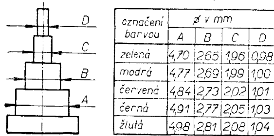
Obr. 12. Odstupňování rozměrů kladek pro asynchronní motorek
