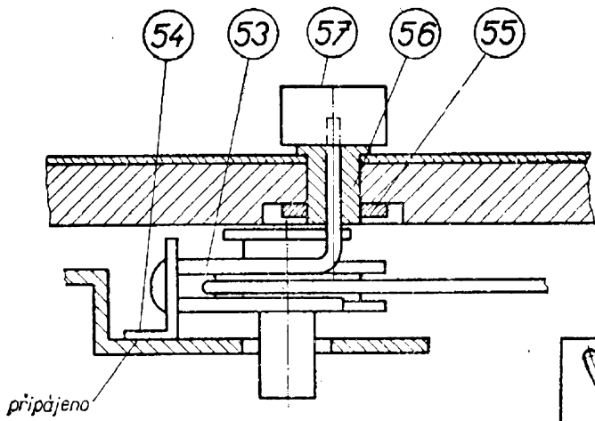
Sestava a detaily pohonného mechanismu a nosného panelu
