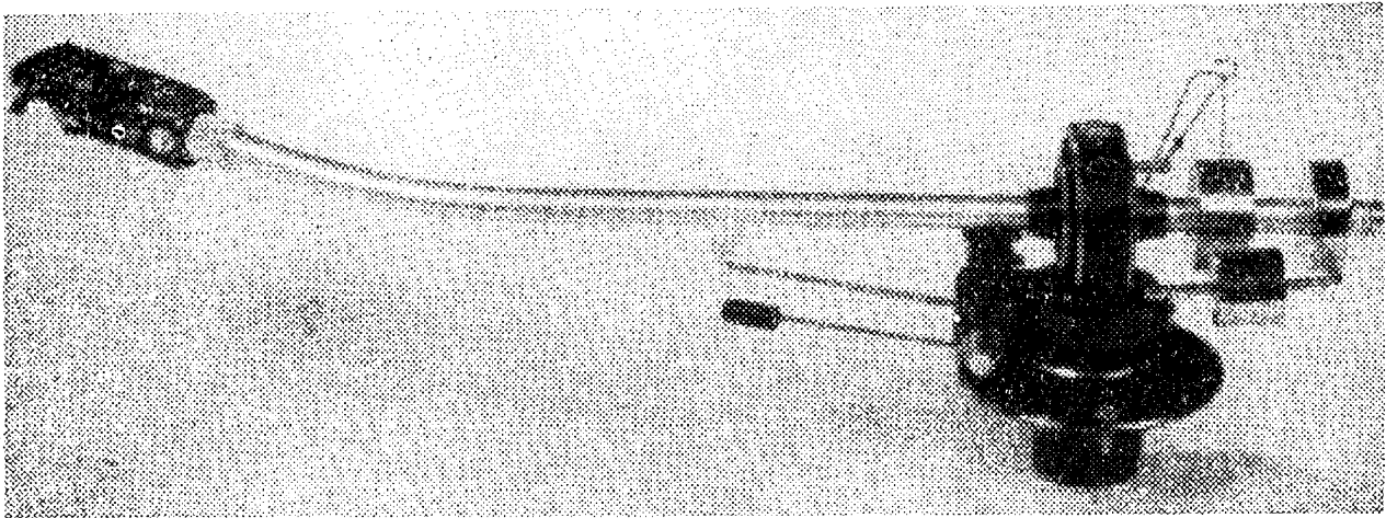
Obr. 13. Velmi kvalitní čs. přenoska P1101 Tesla Litovel, která získala první stupeň jakosti a je vybrána k registraci nejlepších čs. výrobků s právem používat označení „Vybráno pro CID“
