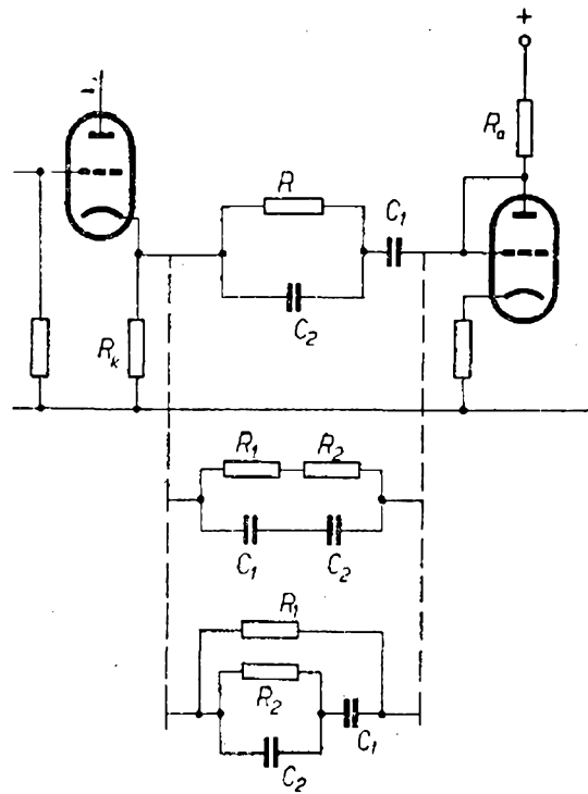
Obr. 35. Korekce v obvodu zpětné vazby
