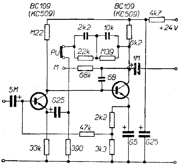
Obr. 42. Předzesilovač pro mikrofon a rychlostní vložku (pro jeden kanál)
