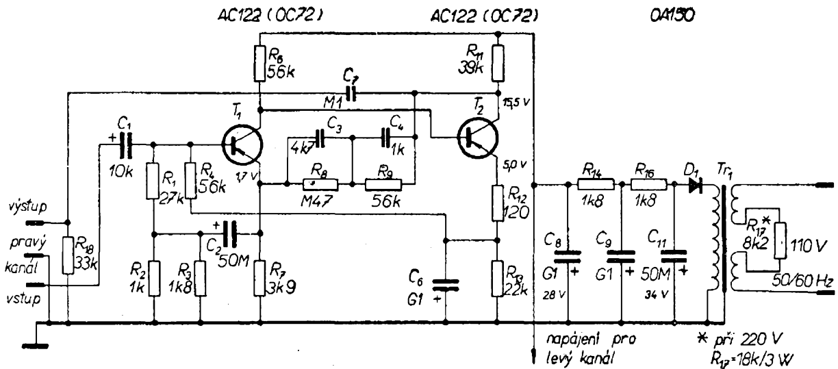
Obr. 38. Předzesilovač pro jeden kanál se dvěma tranzistory
