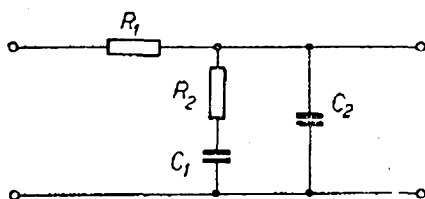
Obr. 34. Pasivní čtyřpól
