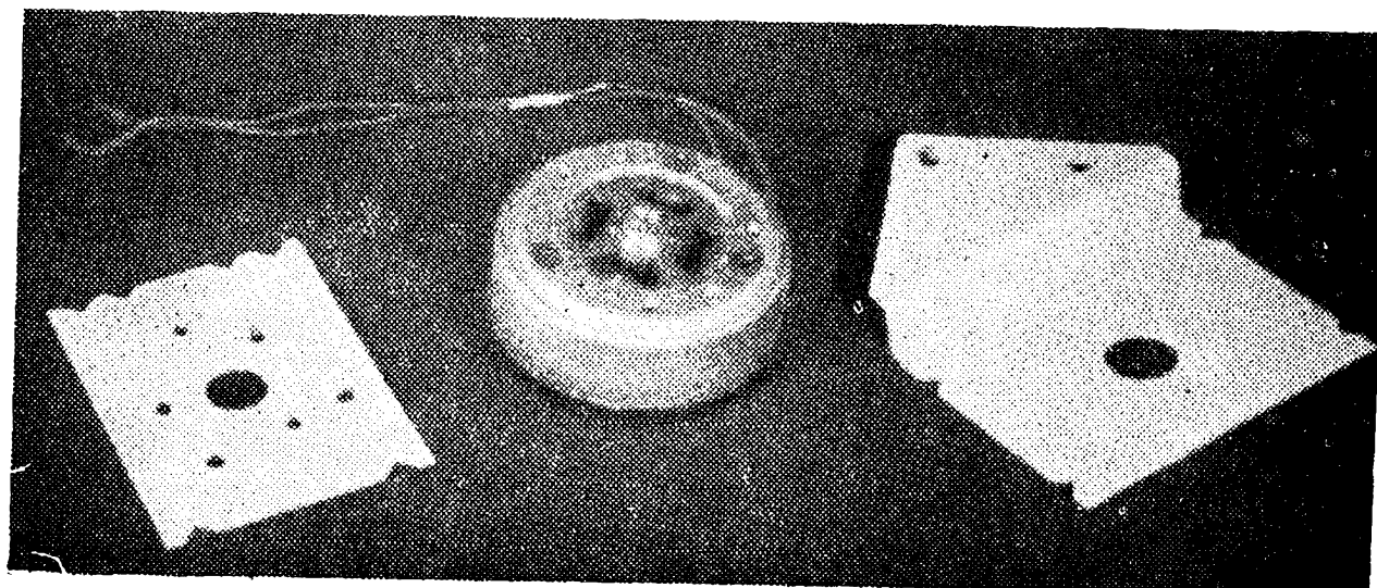
Motorek SMz 375/R a držák motoru
