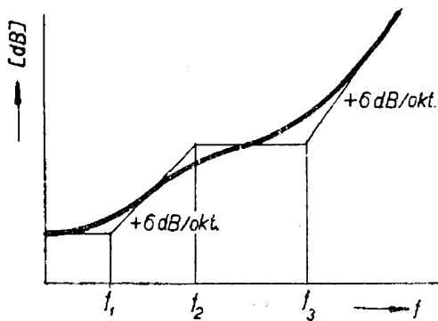
Obr. 33a. Průběh záznamové charakteristiky RIAA
