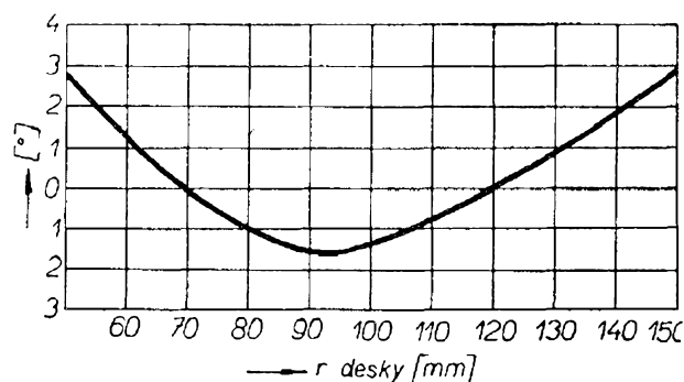
Obr. 24. Typický průběh chyby snímacího úhlu v závislosti na poloměru desky
