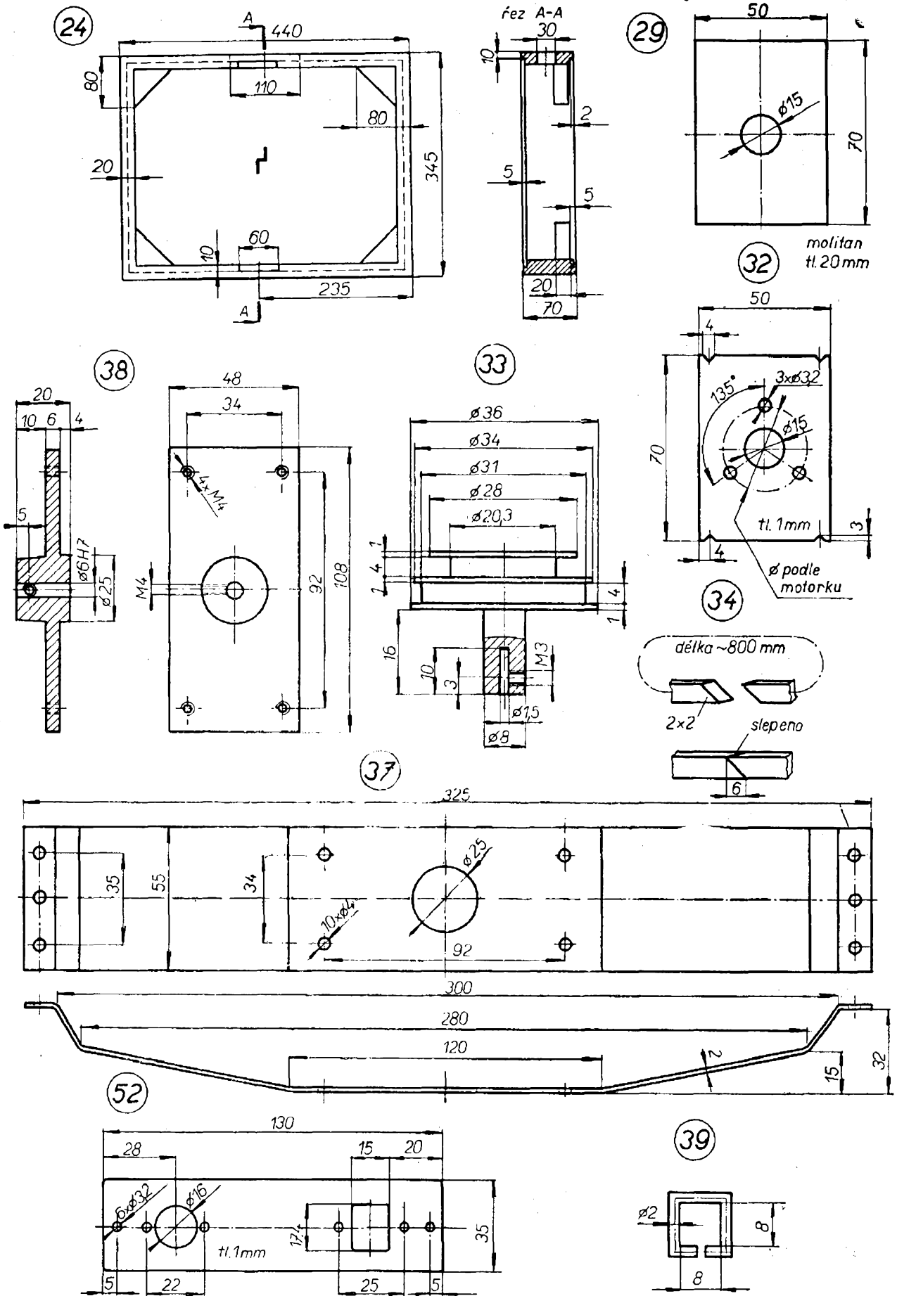
Detaily pohonného mechanismu a nosného panelu (det. 37 viz foto, str. 49)
