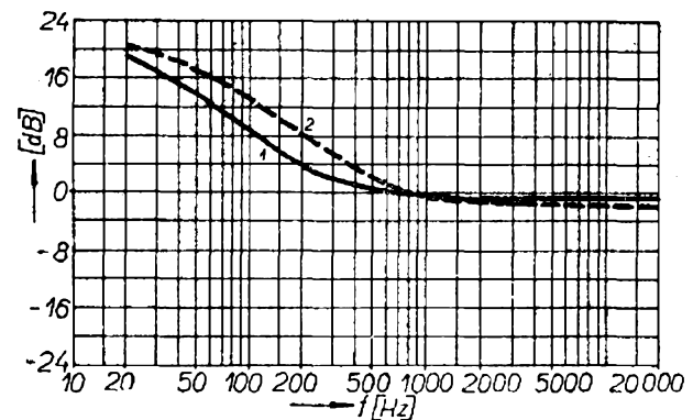
Obr. 40. Korekční kmitočtové průběhy 1, 2
