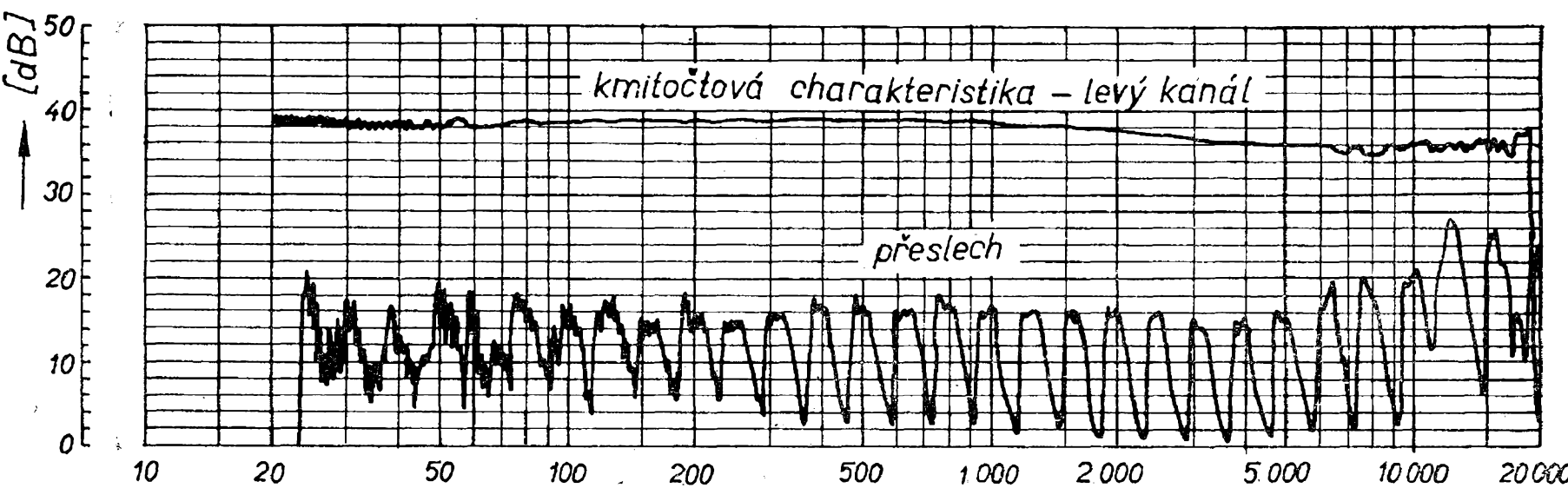
Obr. 26. Kmitočtová charakteristika přenoskové vložky Shure VI5-II v raménku P1101
