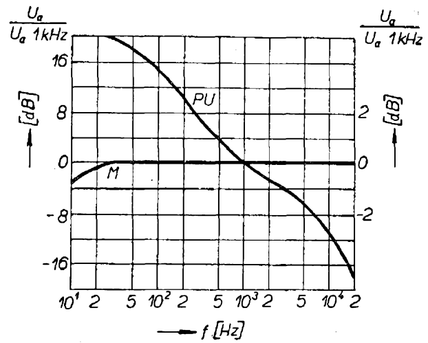
Obr. 43. Kmitočtové charakteristiky předzesilovače
