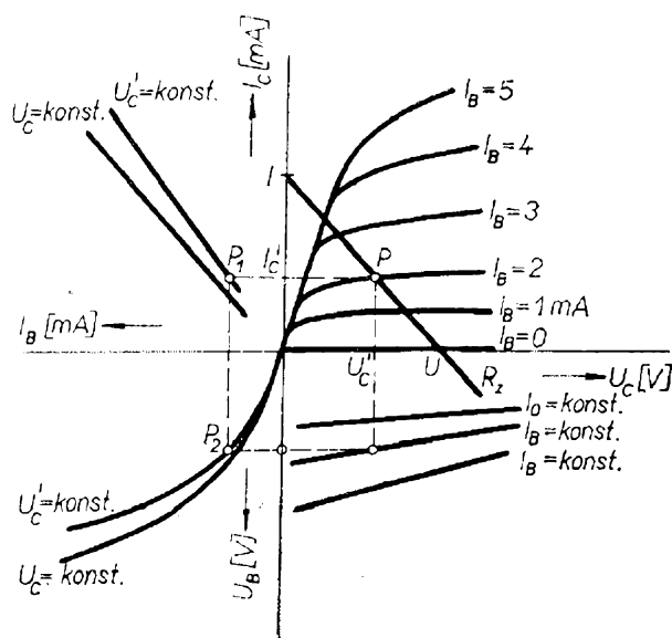
Obr. 29. Statické charakteristiky tranzistoru
