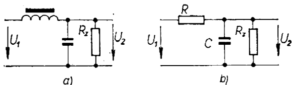
Obr. 56. Vyhlašovací filtry
