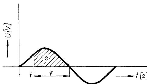
Obr. 40. Spínání tyristoru
