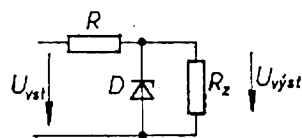
Obr. 58. Stabilizátor se Zenerovou diodou
