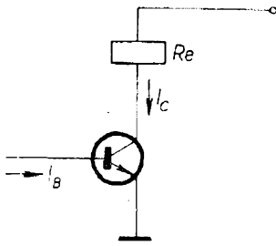
Obr. 34. Tranzistor jako spínač
