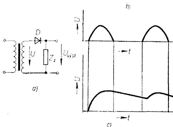
Obr. 51. Jednocestný usměrňovač
