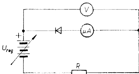
Obr. 23. Měření závěrné charakteristiky
