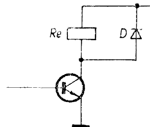
Obr. 36. Indukční zátěž
