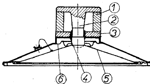
Obr. 16. Konstrukce reproduktoru
