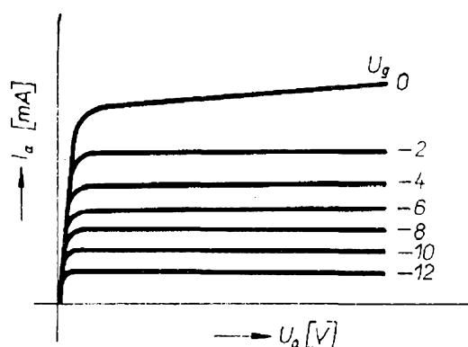
Obr. 19. Průběhy anodových charakteristik
