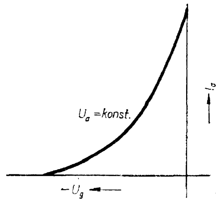
Obr. 18. Převodní charakteristika
