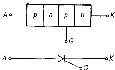
Obr. 38. Tyristor
