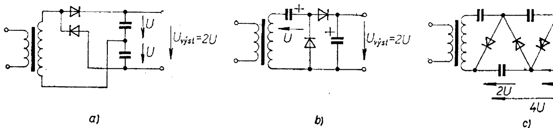
Obr. 55. Zdvojovače a násobiče napětí
