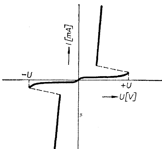
Obr. 49. Charakteristika diaku
