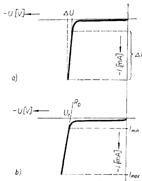
Obr. 24. Charakteristika Zenerovy diody
