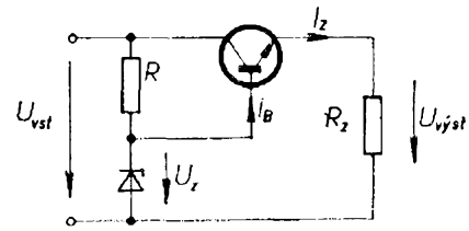
Obr. 62. Stabilizátor s jedním tranzistorem
