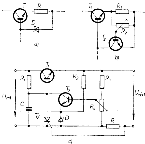
Obr. 65. Elektronická pojistka
