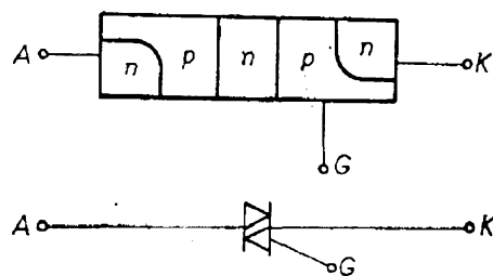
Obr. 46. Triak
