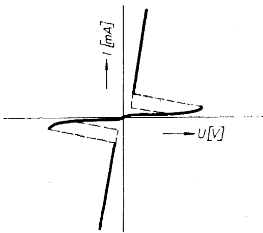
Obr. 47. Charakteristika triaku
