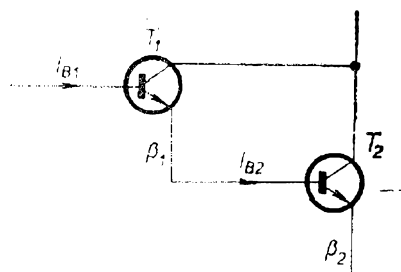
Obr. 32. Darlingtonovo zapojení tranzistorů
