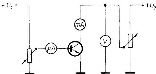
Obr. 35. Měření tranzistorů
