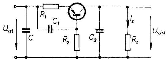
Obr. 57. Elektronický filtr
