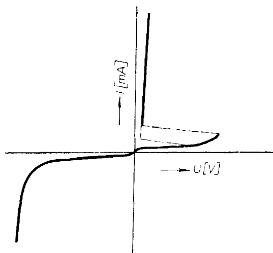
Obr. 39. Charakteristika tyristoru
