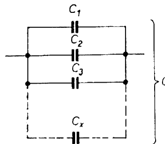
Obr. 8. Řazení kondenzátorů paralelně
