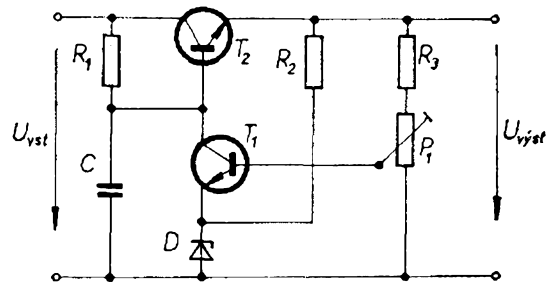
Obr. 63. Stabilizátor s regulačním tranzistorem
