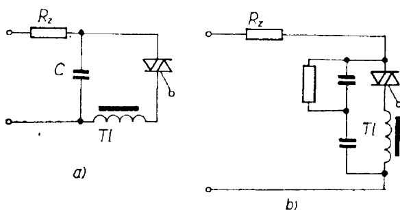
Obr. 50. Odrušení pro tyristorové a triakové obvody
