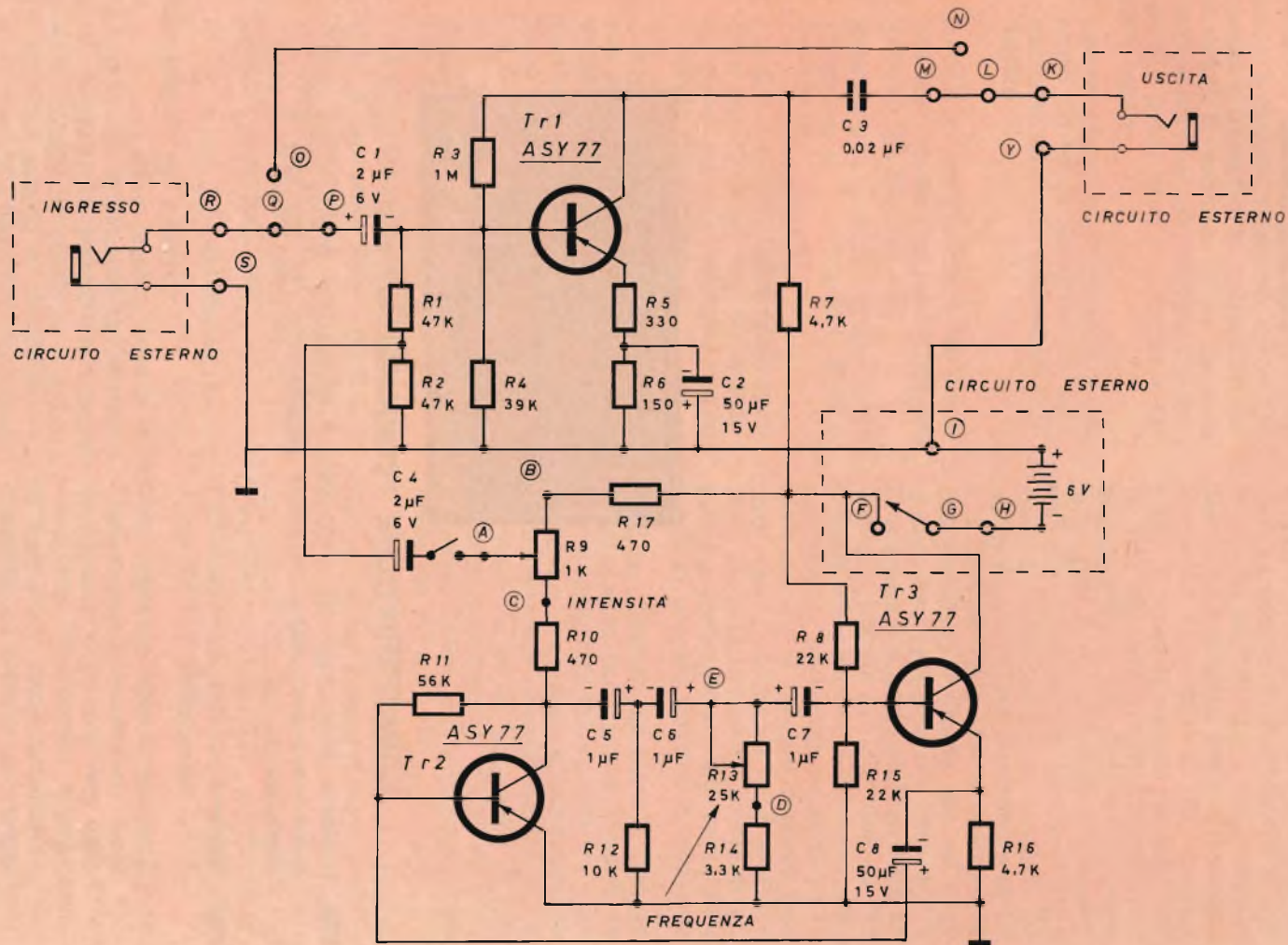
Fig. 1 - Schema di principio del circuito elettrico.
