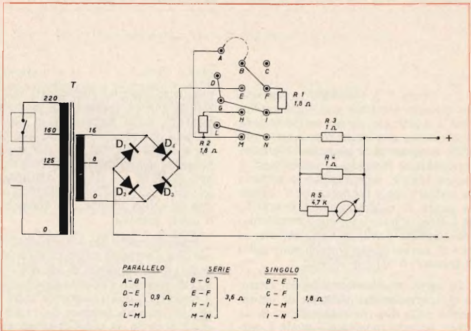
Fig. 1 - Schema elettrico del carica batterie.
