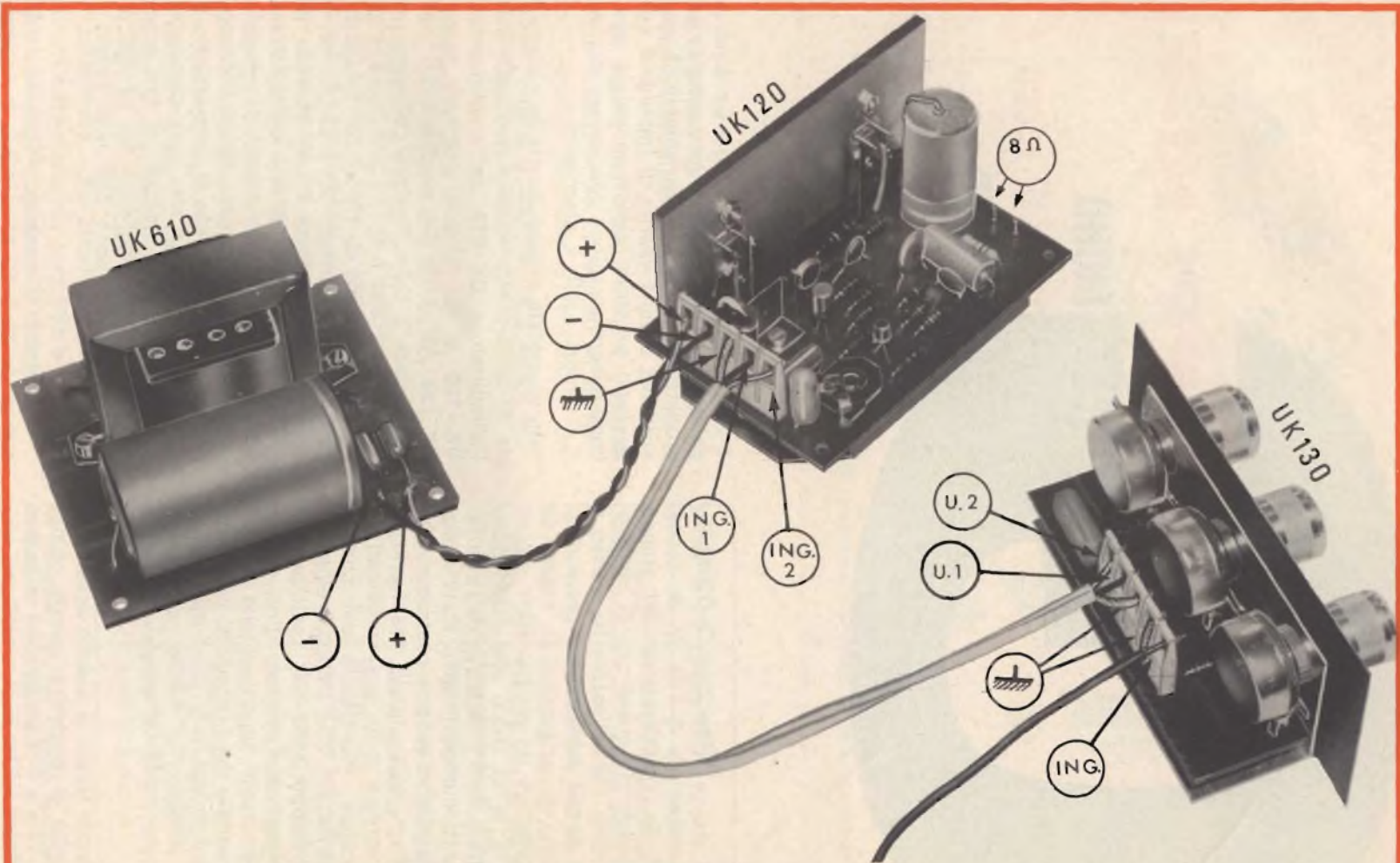
Fig. 1 - Aspetto d'insieme del gruppo HI-FI mono da 12 W di picco. Esso è composto dall'alimentatore UK 610 dall'amplificatore UK 120 e dal gruppo comandi mono UK 130. La figura mette in evidenza le connessioni fra i vari nuclei.
