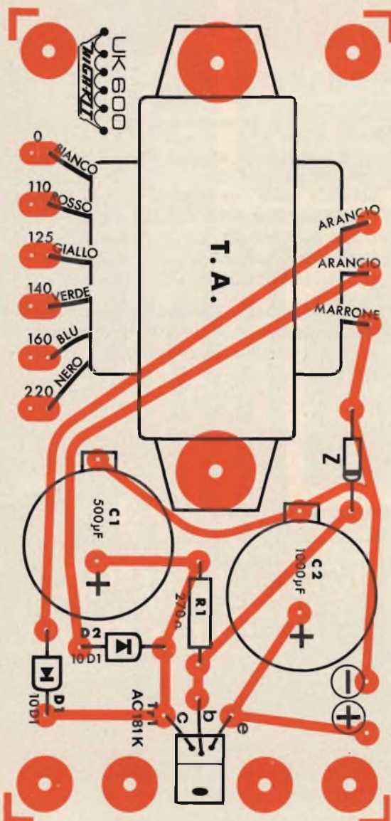
Fig. 2 - Disposizione dei componenti sulla piastra a circuito stampato.
