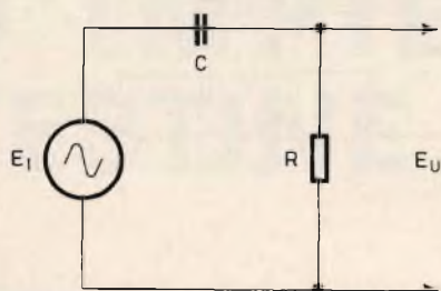
Fig. 2 - Circuito equivalente di una testina ceramica, rappresentata dalla capacità C. E_1 rappresenta la tensione di ingresso fornita dalla testina, che funge da generatore di tensione alternata, R rappresenta la resistenza di carico, ed E_0 la tensione di uscita disponibile ai capi del carico stesso.
