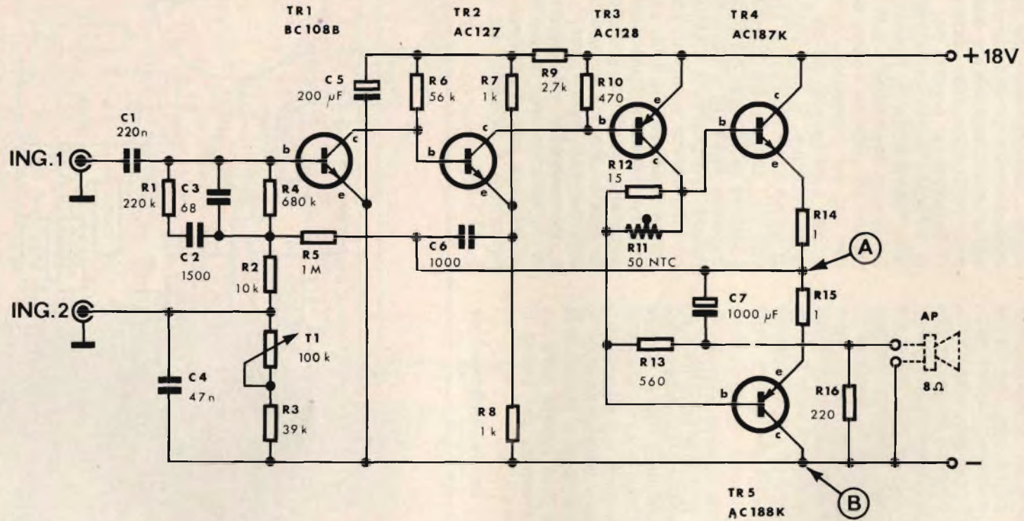
Fig. 1 - Schema elettrico dell'amplificatore UK 115.
