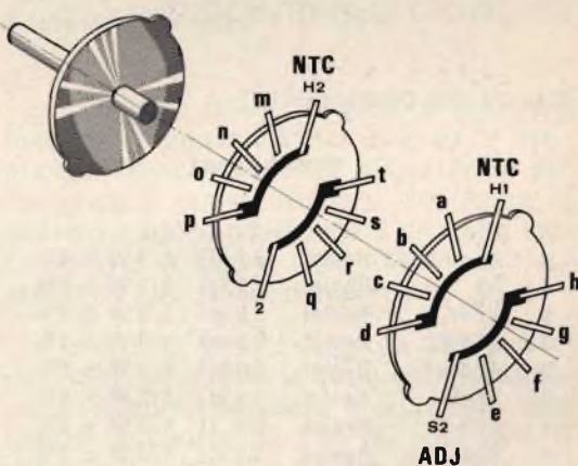
Fig. 4 - Vista in sezione del commutatore rotativo S1.
