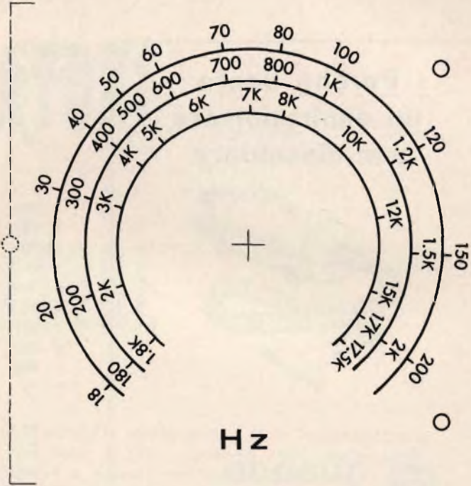
Fig. 7 - Tracciatura della scala di sintonia (scala 1 : 1).
