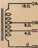
Fig. 6 - Uso di prese sul secondario del trasformatore per l'adattamento di impedenza.
