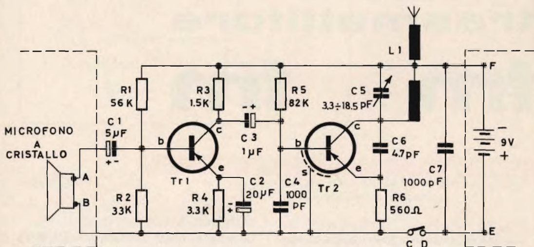
Fig. 1 - Schema di principio del circuito elettrico.
