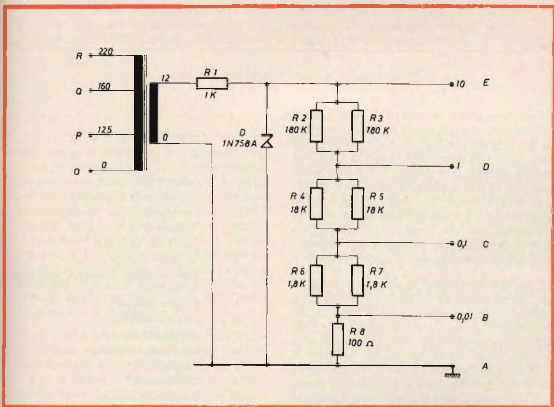
Fig. 1 - Schema elettrico.
