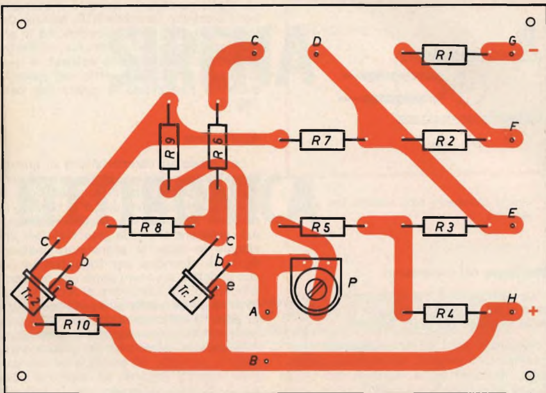
Fig. 2 - Montaggio dei componenti sul circuito stampato.
