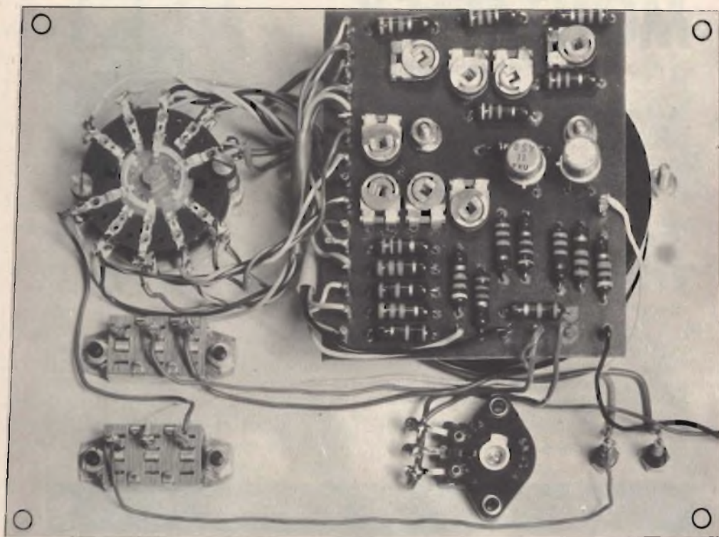
Vista posteriore del pannello comandi.
