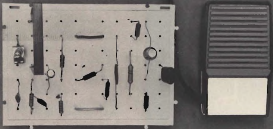
In figura: trasmettitore completo su di un S-DeC.
