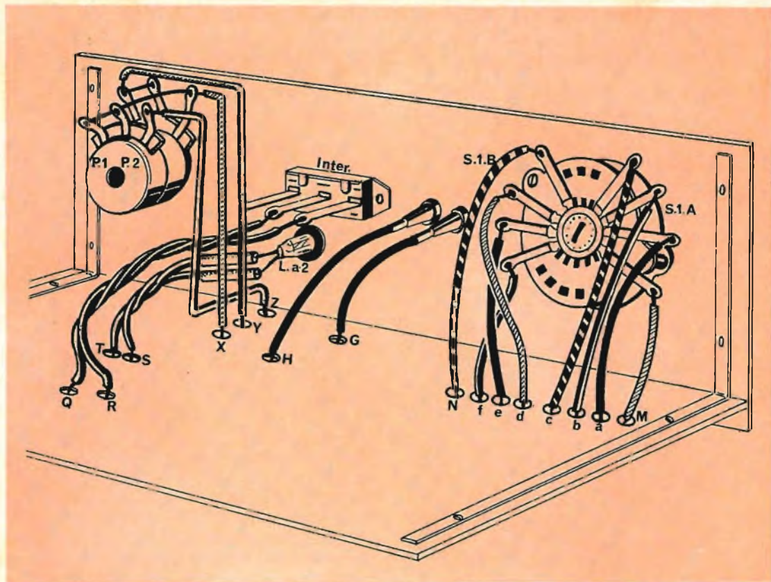
Fig. 6 - Schema di montaggio dei componenti sul pannello frontale.
