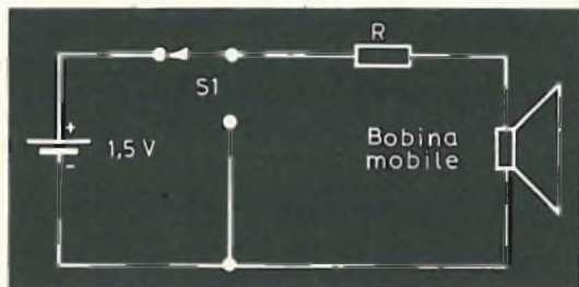
Fig. 2 - Circuito per determinare lo smorzamento.
