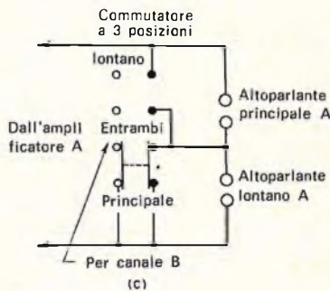
Fig. 4 - Vari circuiti di commutazione che possono essere usati per mettere in funzione un altoparlante a distanza.
