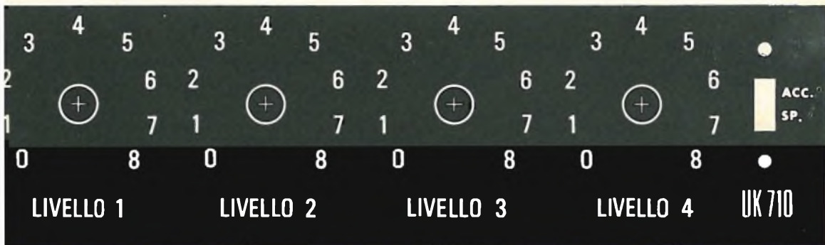
Fig. 6 - Dima di foratura al naturale del pannello frontale.
