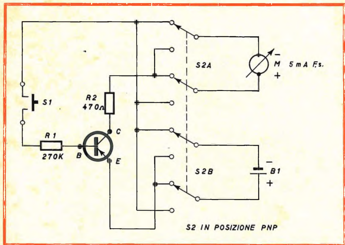
Fig. 1 - Schema elettrico del provatransistor.
