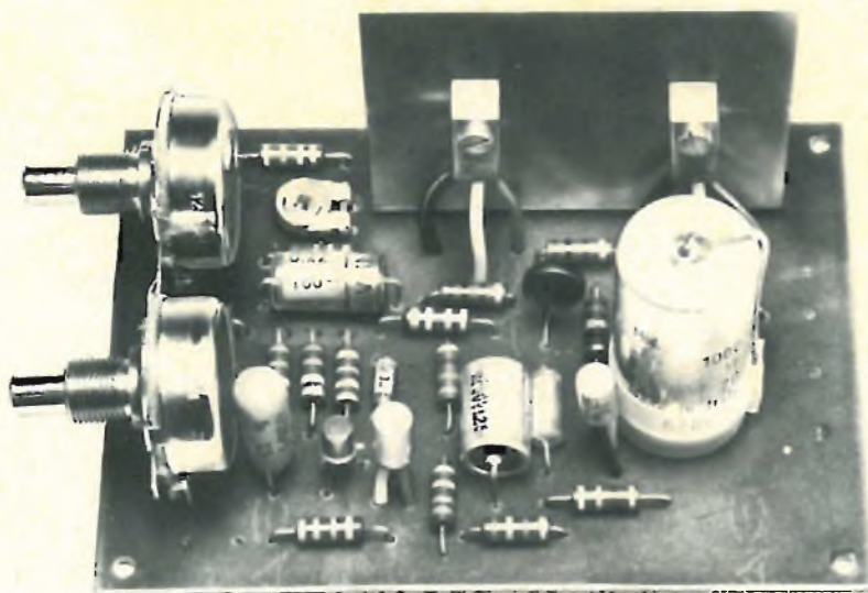
Vista dell'amplificatore a montaggio ultimato.
