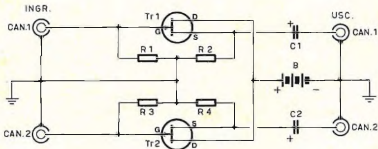
Fig. 4 - Circuito elettrico di uno stadio di ingresso per testina ceramica stereo, che — con un carico di 200.000 ohm per ciascun canale, fornisce un responso lineare da 20 Hertz a 15.000 Hertz, entro \pm 0,5 dB.
