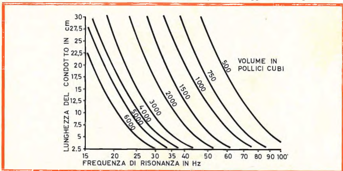
Fig. 6 - Nomogramma per calcolare la lunghezza del condotto, adottando per lo stesso un diametro di 5 centimetri.
