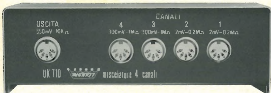
Fig. 5 - Aspetto della parte posteriore dell'UK 710.
