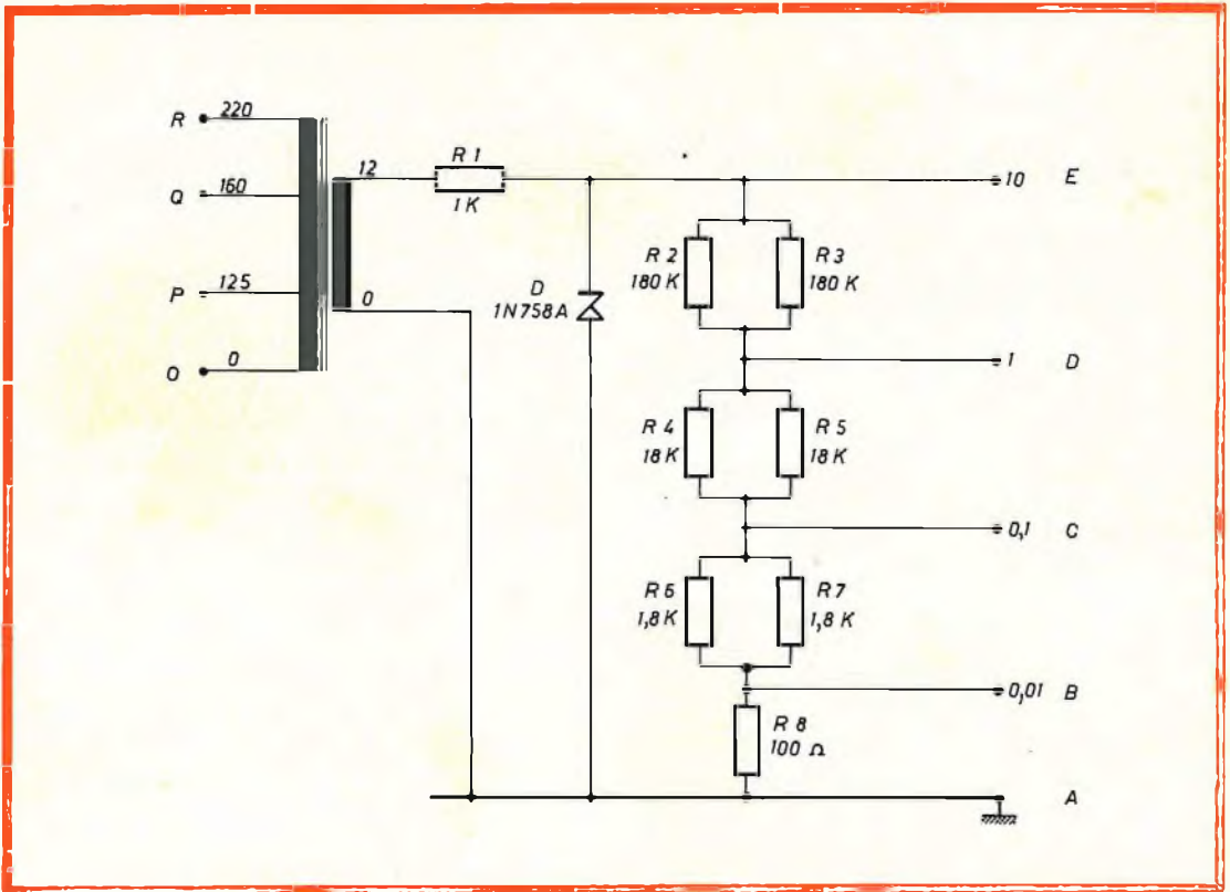
Fig. 1 - Schema elettrico.
