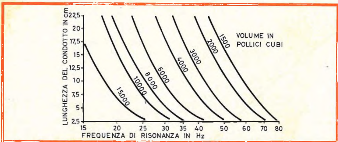
Fig. 7 - Nomogramma per calcolare la lunghezza del condotto adottando per lo stesso un diametro di 7,5 centimetri.
