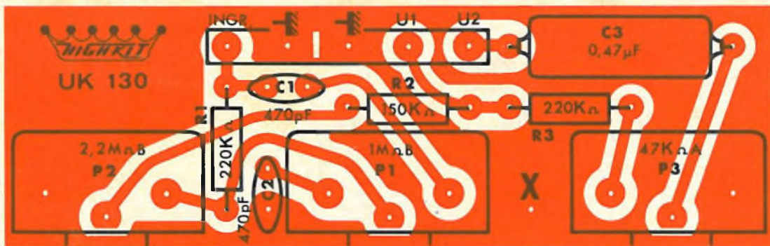
Fig. 2. - Serigrafia del circuito stampato
