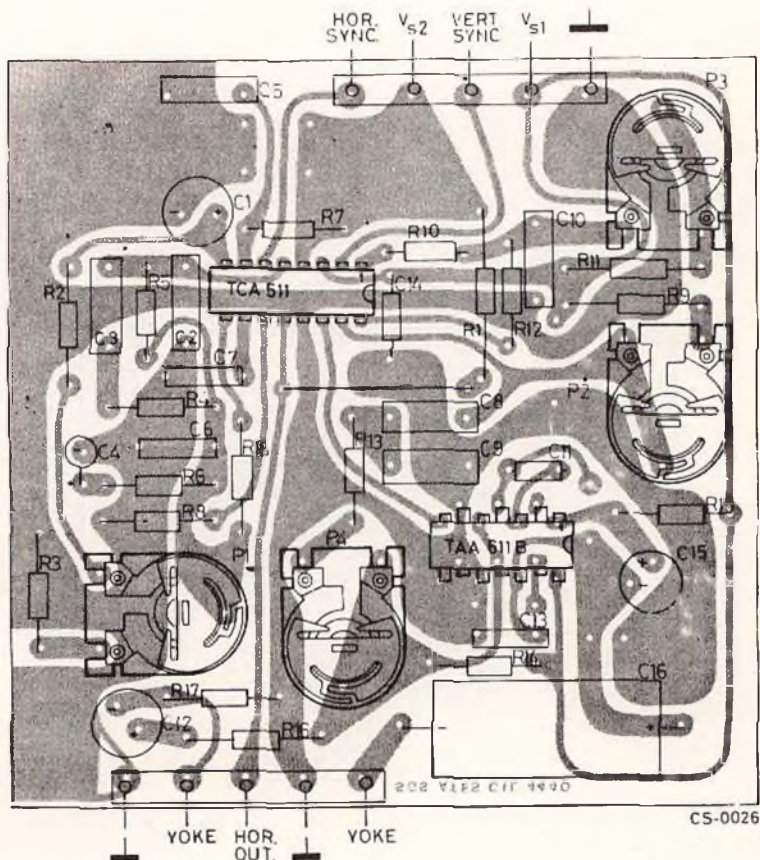
Fig. 6 - Circuito stampato e disposizione dei componenti relativi al circuito di fig. 5 (scala 1:1)
