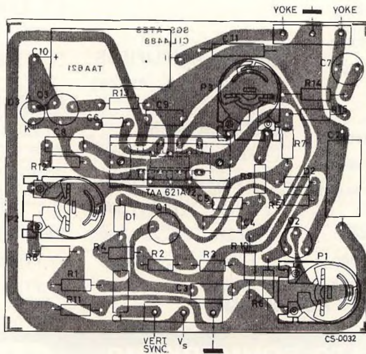
Fig. 30 - Circuito stampato e disposizione dei componenti relativi al circuito elettrico di fig. 29.
