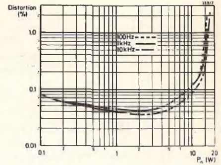
Fig. 18 - Distorsione in funzione della potenza di uscita nell'amplificatore da 15 W/4 \Omega .
