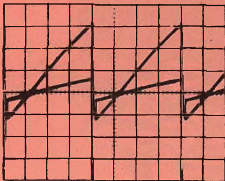
Fig. 27 - Corrente e tensione di giogo. Scala verticale: I_Y = 200 mA/div.; V_Y = 10 V/div.; Scala orizzontale: 5ms/div.
