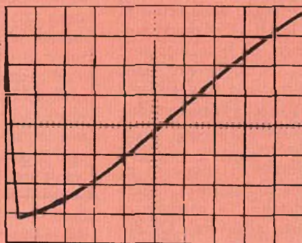
Fig. 2 - Corrente di giogo con P_s = 0 \Omega . Scala verticale: 100 mA/div.; Scala orizzontale: 2ms/div.
