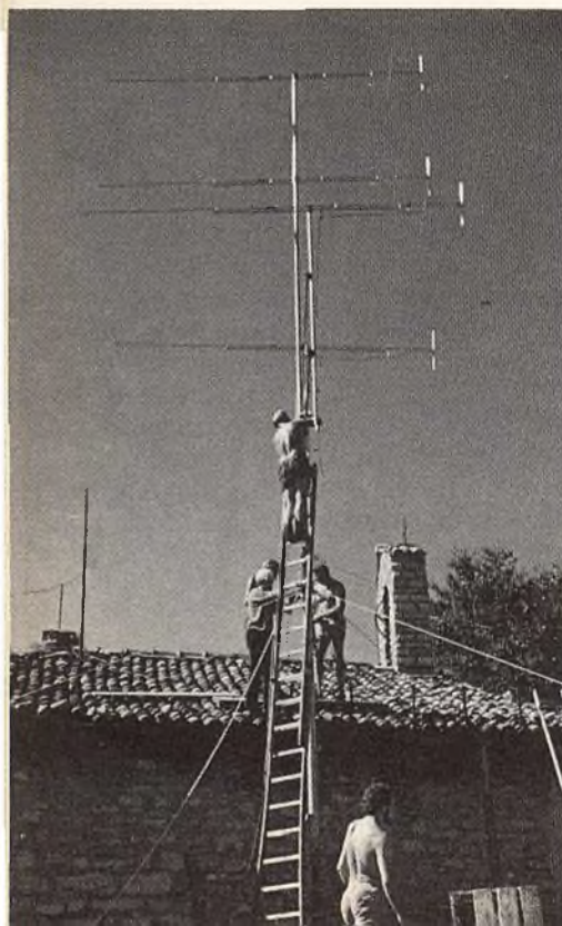
Figg. 3-4 - Fasi di montaggio dell'antenna HB9SV particolarmente delicate in cui necessitano stabilità d'appoggio base, controventatura a mezzo tiranti a scivolamento e molta fatica di braccia.
