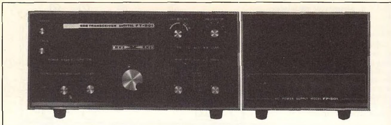
Fig. 6 - Ricetrasmittitore Sommerkamp FT-501 con alimentatore FP-501.
