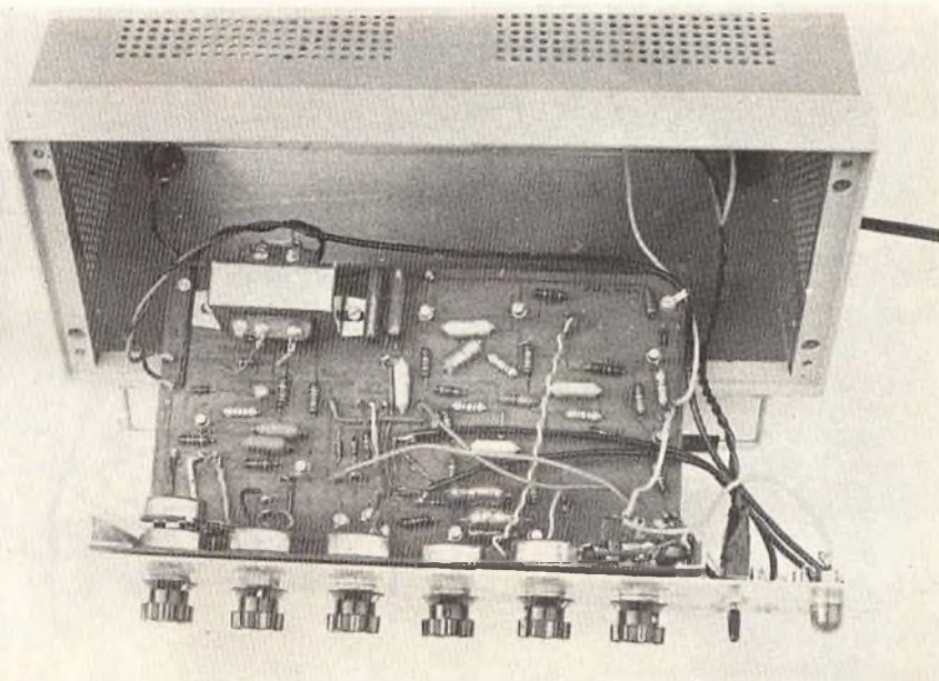
Foto 14 - Vista interna del primo prototipo realizzato, del generatore descritto in queste pagine: brutto, eppure funziona! d'altro canto non ci può essere una bella copia, se non c'è stata prima una brutta copia!
