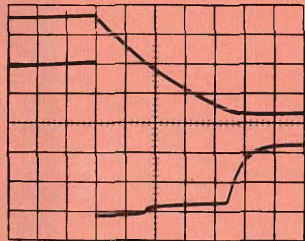
Fig. 8 - Corrente di giogo e tensione di uscita del TBA820 durante il tempo di ritraccia. Scala verticale: I_Y = 200 \text{ mA/div.} ; V_o = 2 \text{ V/div.} ; Scala orizzontale: 200 \mu\text{s/div.}
