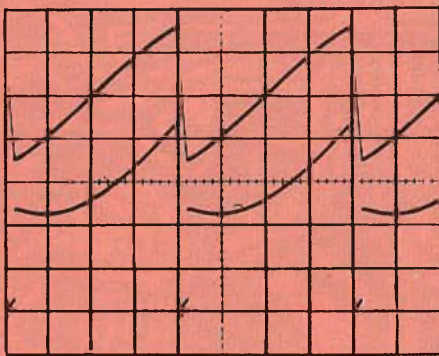
Fig. 11 - Corrente di giogo e tensione di uscita del TBA641B. Scala verticale: I_Y = 500 mA/div.; V_a = 2 V/div.; Scala orizzontale: 5 ns/div.
