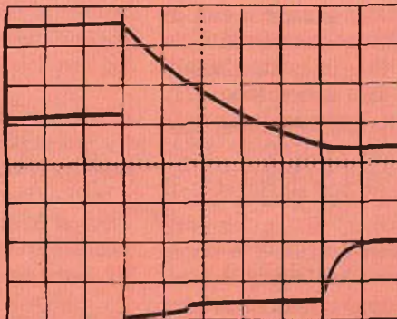
Fig. 4 - Corrente di giogo e tensione di uscita del TAA611B durante il tempo di ritraccia. Scala verticale: I_Y = 200 \text{ mA/div.} ; V_o = 2 \text{ V/div.} ; Scala orizzontale: 200 μs/div.
