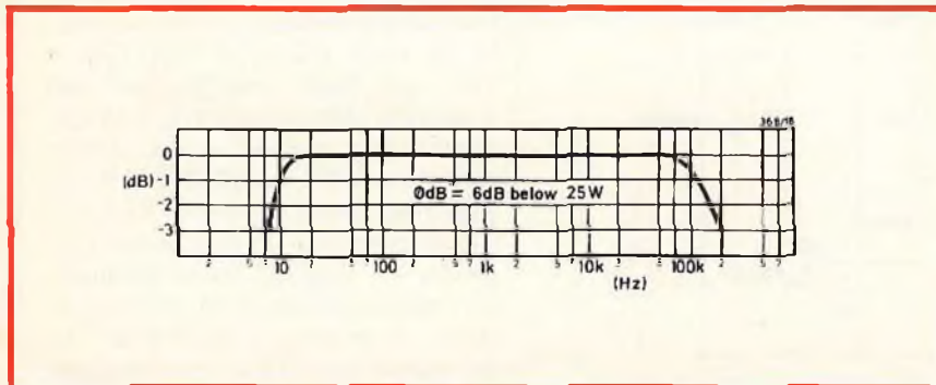
Fig. 32 - Risposta in frequenza dell'amplificatore da 25 W/8 Ω.
