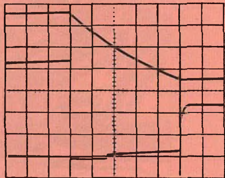
Fig. 16 - Corrente di giogo e tensione di uscita del TBA810S durante il tempo di ritraccia. Scala verticale: I_Y = 500 mA/div.; V_o = 2 V/div.; Scala orizzontale: 200 μs/div.
