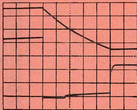
Fig. 12 - Corrente di giogo e tensione di uscita del TBA641B durante il tempo di ritraccia. Scala verticale: I_Y = 500 mA/div.; V_a = 2 V/div.; Scala orizzontale: 200 μs/div.
