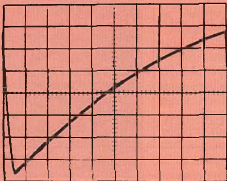
Fig. 1 - Corrente di giogo con P_s = 100 \text{ k}\Omega . Scala verticale: 100 mA/div.; Scala orizzontale: 2ms/div.
