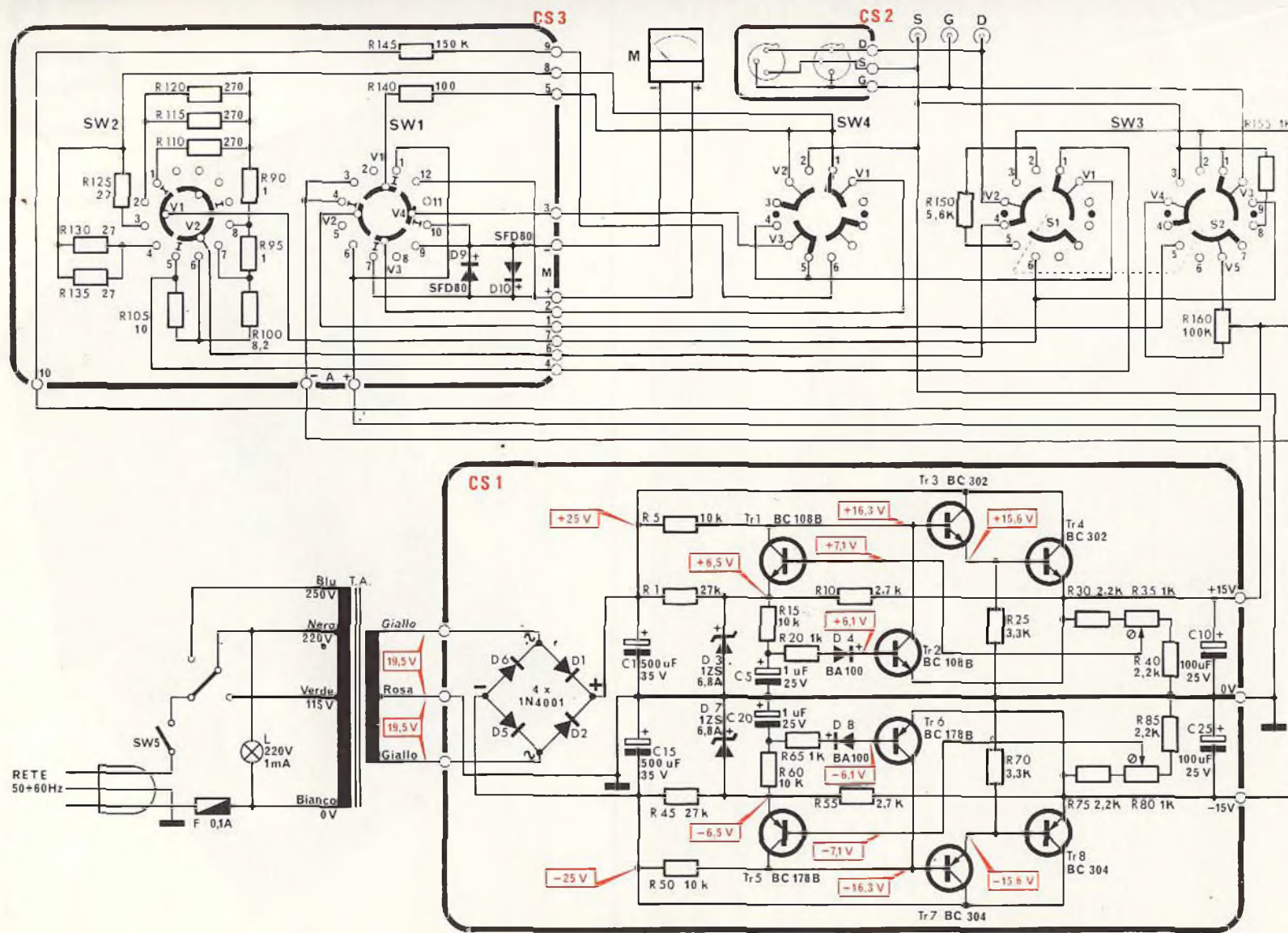
Fig. 3 - Schema elettrico.
