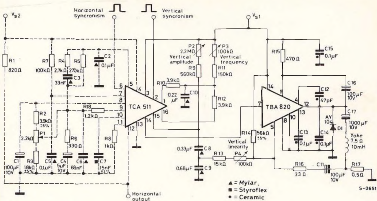
Fig. 9 - Schema del circuito di deflessione verticale per tubi catodici 12" 90° con impiego del TBA820.
