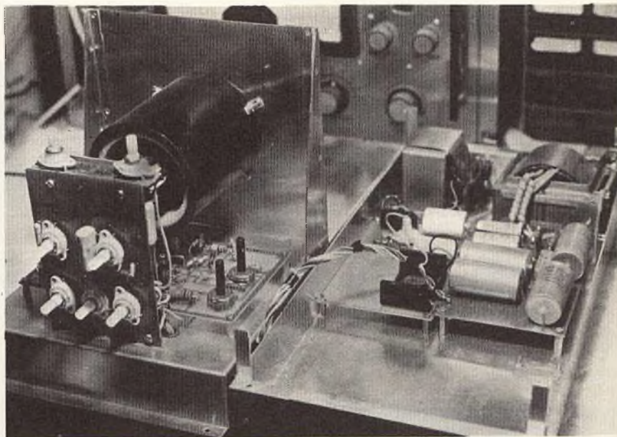
Foto 18 - Vista dei circuiti relativi al fototubo, che completano la parte trasmettente SSTV: verranno descritti nella seconda parte, pubblicata in uno dei prossimi numeri. Da notare la mancanza dell'alimentatore ad alta tensione per il fototubo (1800 V) da noi alimentato in modo del tutto originale, con notevole risparmio di componenti.
