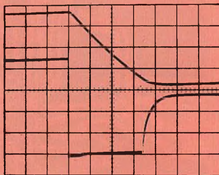
Fig. 20 - Corrente di giogo e tensione di uscita del TBA800 durante il tempo di ritraccia. Scala verticale: I_Y = 200 mA/div.; V_o = 5 V/div.; Scala orizzontale: 200 μs/div.
