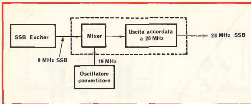
Fig. 6 - Lo stadio converter trasla l'uscita dell'eciter alla frequenza di trasmissione.
