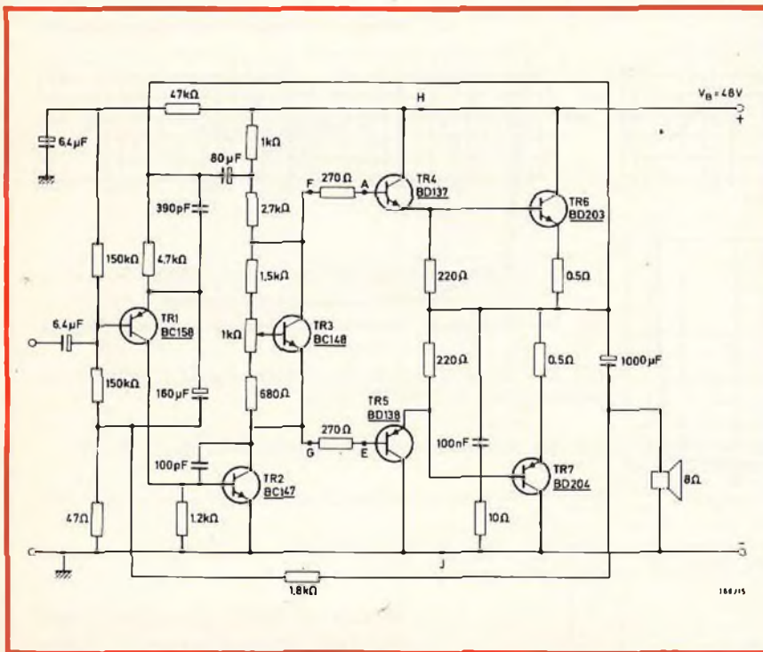
Fig. 31 - Schema elettrico dell'amplificatore da 25 W/8 Ω.
