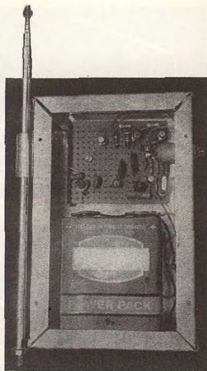
Fig. 16 - Aspetto del trasmettitore dopo la costruzione, visto dal retro, col coperchio asportato per chiarire la posizione della basetta di supporto e della batteria di alimentazione, nonché il metodo di fissaggio del pulsante e dell'antenna a stilo.
