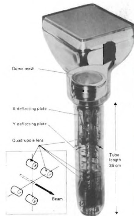
Fig. 5b - Struttura interna del CRT utilizzato dalla IWATSU.
