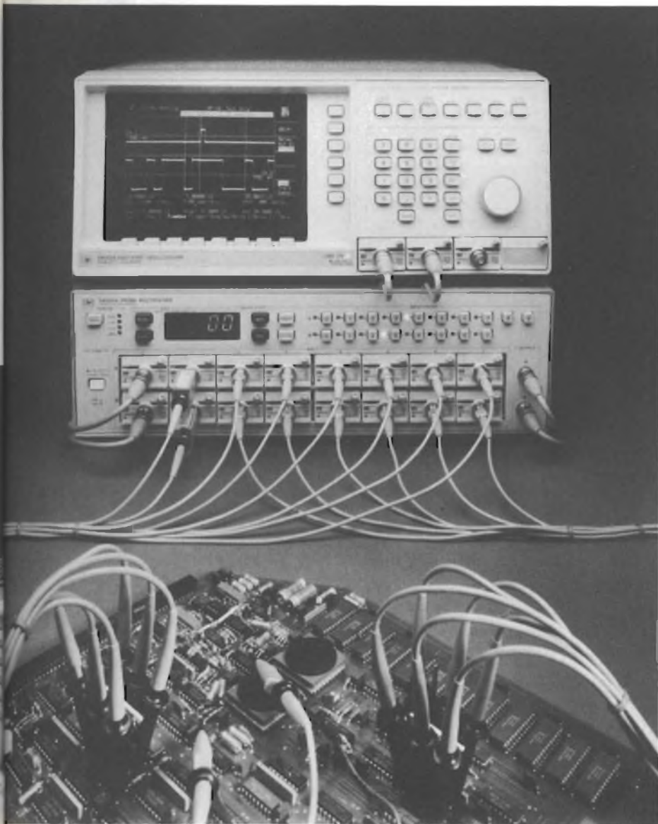
Fig. 3 - I fronti di salita e di discesa degli impulsi con durata dell'ordine del nanosecondo (circuiti logici veloci) possono essere visualizzati istantaneamente su carta sia ricorrendo ad un plotter che ad una stampante grafica; si eliminano così le costose e macchinose riprese fotografiche.
