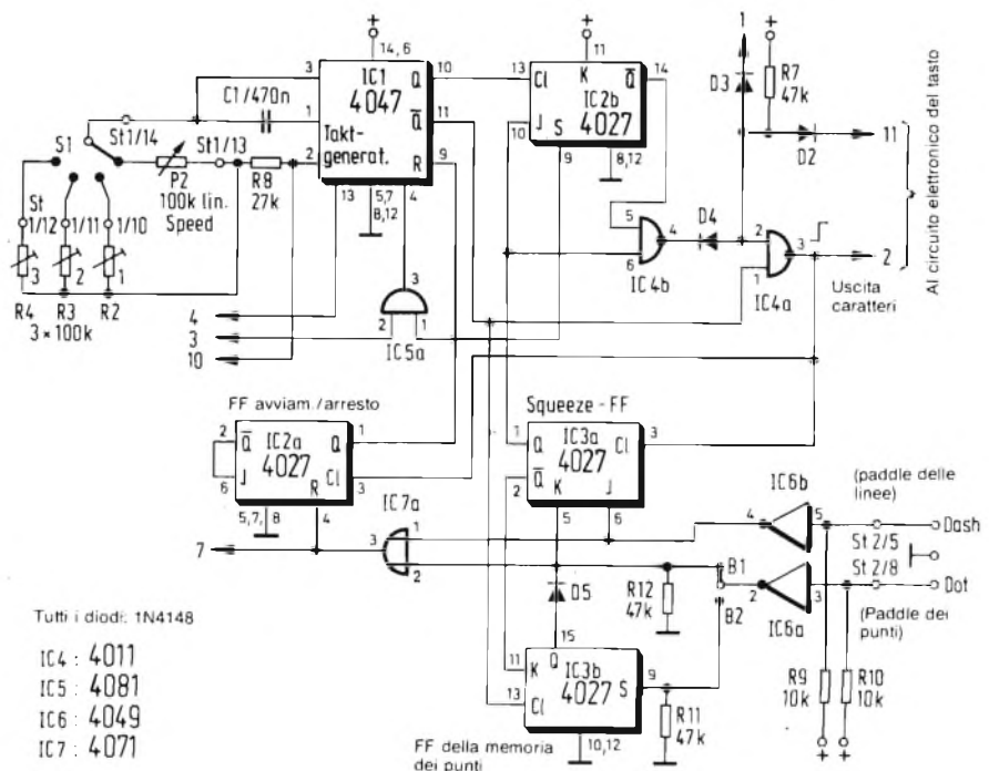
Fig. 5 - Schema del circuito elettronico "squeeze". Gli ingressi e le uscite vanno ai punti di connessione con identico contrassegno, sugli altri moduli circuitali.
