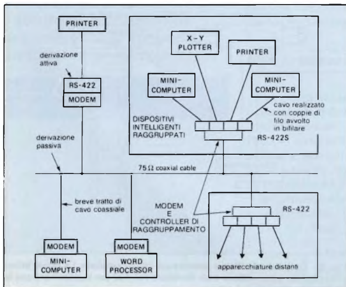
Fig. 3 - Una rete token-passing con struttura a bus (IEEE P802.4) può utilizzare molti modem e qualsiasi combinazione di prese attive e passive. Controller intelligenti smistano il traffico a utenti raggruppati tramite interfacce RS-422.
