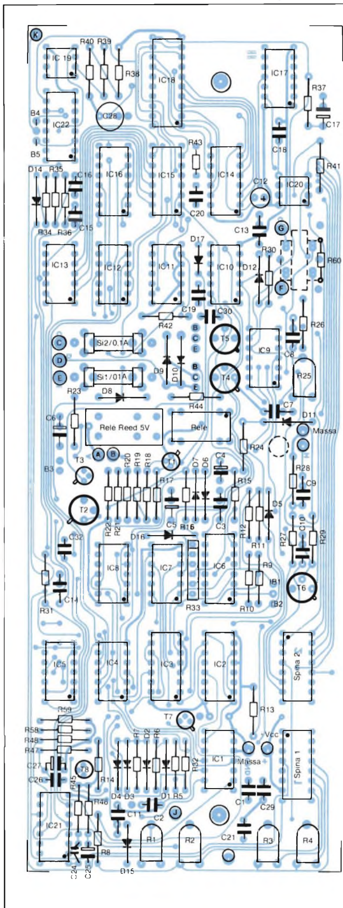
Fig. 12 - Disposizione dei componenti sul circuito stampato principale. Per i condensatori sono state previste diverse distanze tra i terminali.
