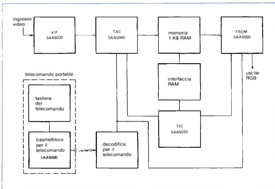
Fig. 3 - Schema a blocchi di decodificatore teletext della prima generazione realizzato con circuiti integrati LSI.
