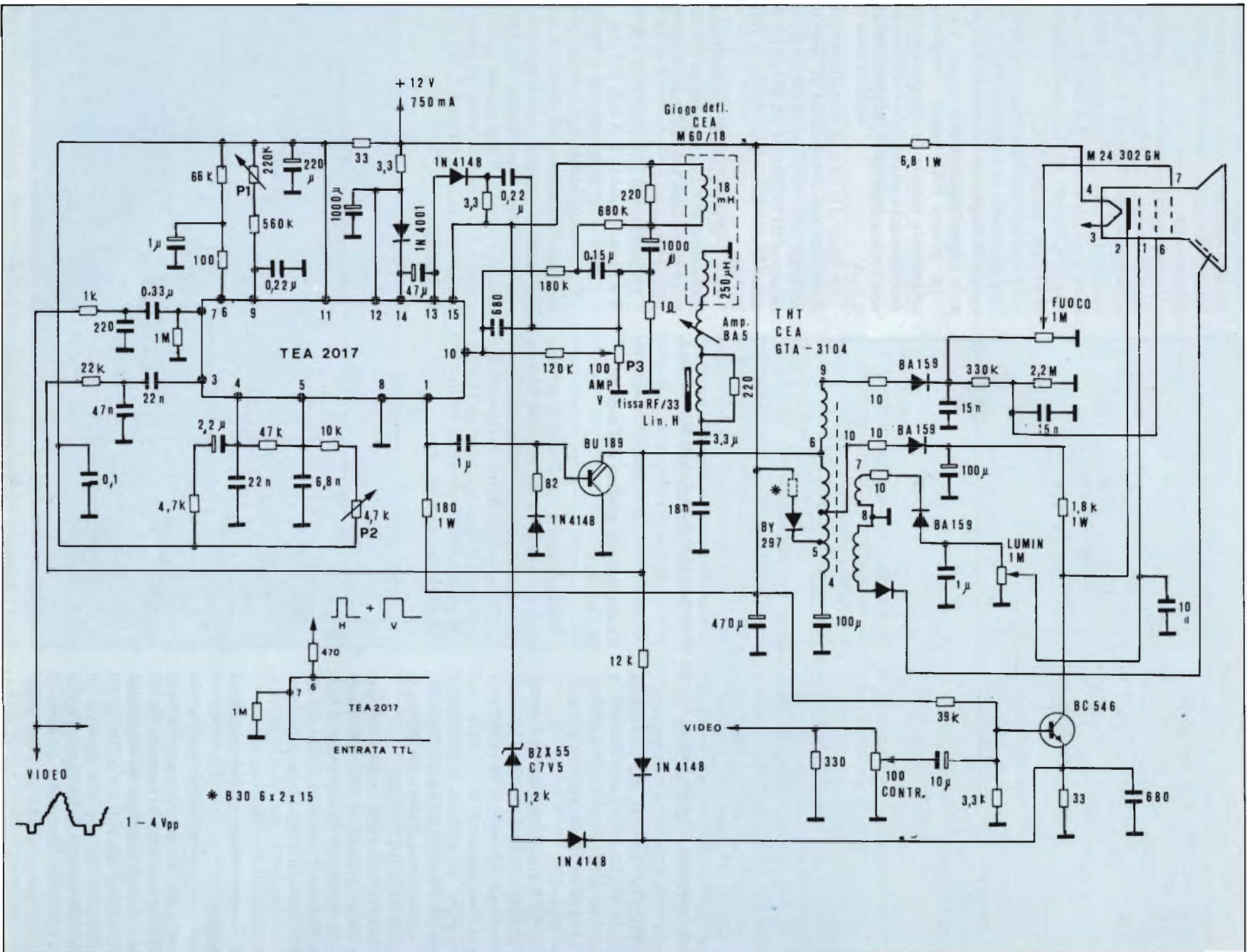
Fig. 8 - Schema elettrico completo del monitor bianco/nero con cinescopio da 90°, 8 pollici di diagonale. In basso è indicata la configurazione per ingresso di segnali TTL.
