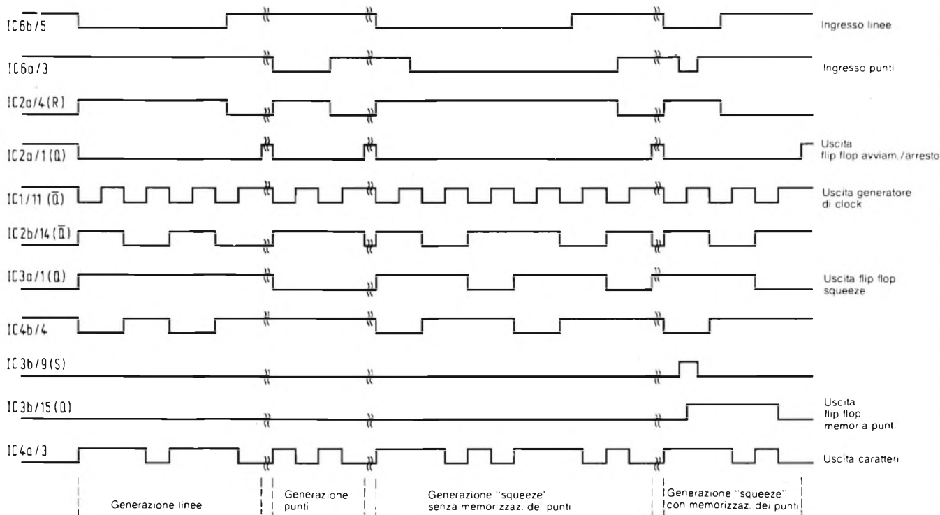
Fig. 6 - Diagramma dei livelli delle più importanti tensioni nel circuito.
