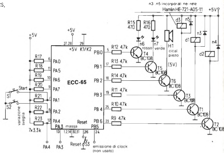
Fig. 4 - Il collegamento all'ECC-65 dei tasti, dei LED e del cicalino piezoelettrico. È consigliabile il montaggio di componenti CMOS sull'ECC-65 (65C04, 65C32, 65C16) per il minor consumo di corrente.
