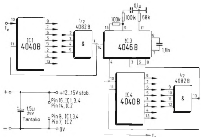
Fig. 2 - Schema del modulo PLL. I diversi rapporti di divisione vengono realizzati mediante ponticelli.
