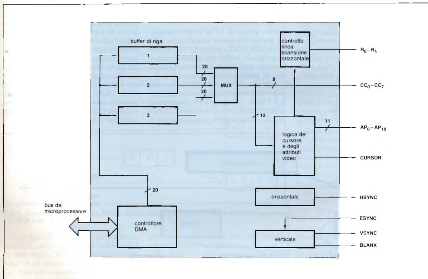
Fig. 2 - Schema a blocchi dello Am8052.
