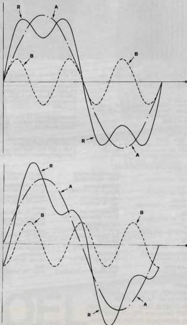
Fig. 6 - Effetto della distorsione di fase su un segnale formato da una fondamentale e dalla sua terza armonica.
