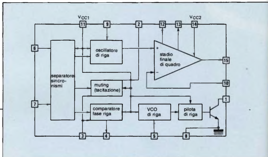
Fig. 1 - Schema a blocchi indicante le funzioni contenute nel c.i. TEA 2017.
