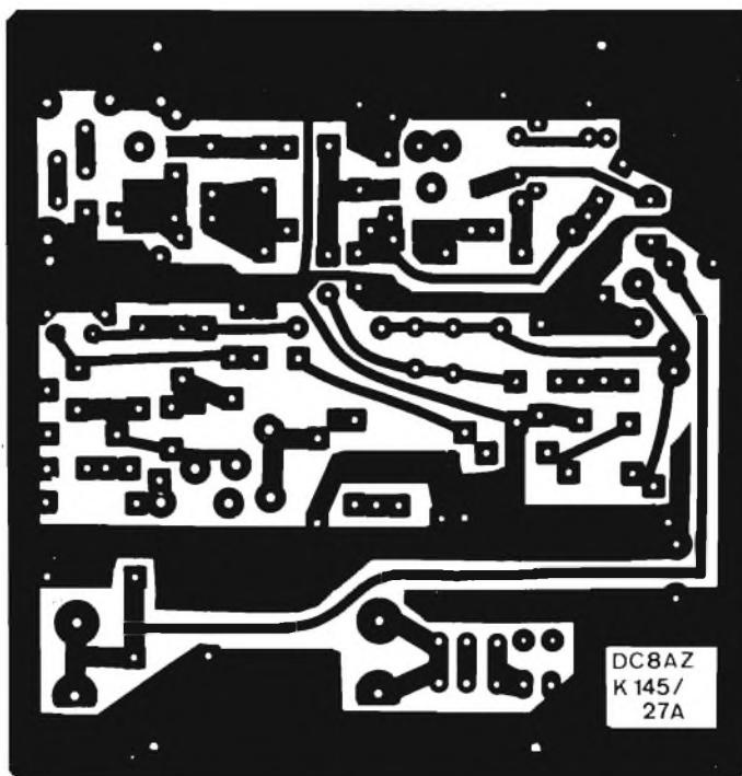
Fig. 2 - Piste di rame del circuito stampato.
