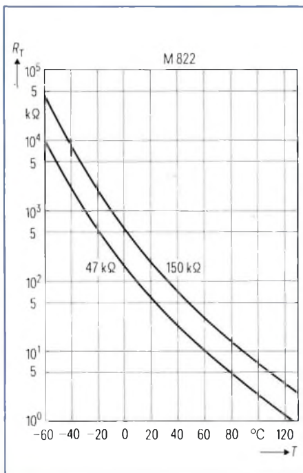
Fig. 6 - Andamento della resistenza R_T del termistore in funzione della sua temperatura T .
