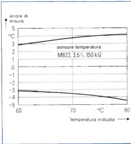
Fig. 7 - Errori massimi di valutazione della temperatura nel sensore M 822. Campo di misura: da 60° a 80 °C. Resistenza in serie al termistore con l'1% di tolleranza.
