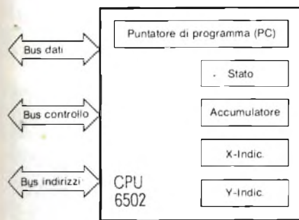
Fig. 2 - I registri interni del 6502.
