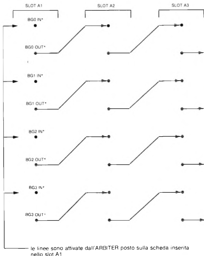
Fig. 6 - Struttura in daisy-chain delle linee di assegnazione del DTB.
