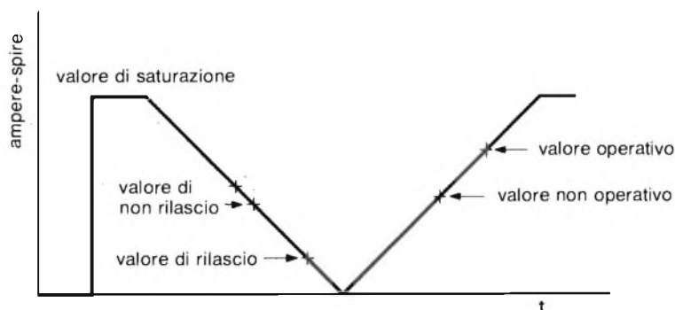
Fig. 3 - Diagramma che illustra la definizione di alcuni parametri fondamentali dei microinterruttori reed.
