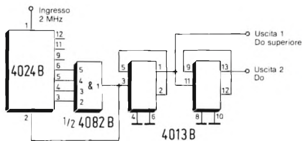
Fig. 7 - Schema del divisore per la nota "do", che permette di ottenere la frequenza del "do superiore".
