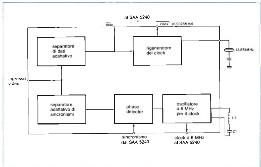
Fig. 5 - Schema a blocchi del processore video VIP2 SAA5230.
