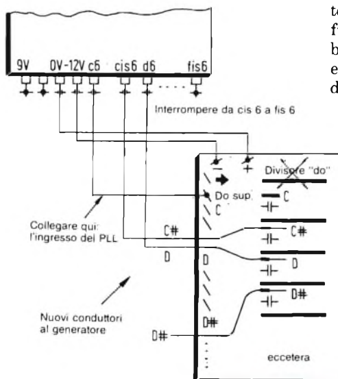
Fig. 16 - Modifiche al cablaggio, necessarie con i modelli più vecchi di organi Boehm. Il divisore "do" ed i 4013 della scheda base non sono necessari, e le note vengono direttamente prelevate dalle uscite degli stadi PLL.
