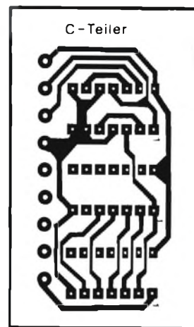
Fig. 8 - Circuito stampato del divisore "do". Anche questa scheda verrà inserita sulla scheda base di figura 9.
