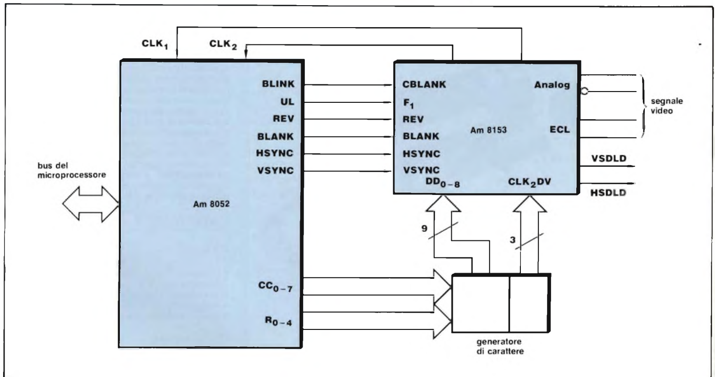
Fig. 1 - Controllore video per terminale CRT con spaziatura proporzionale.
