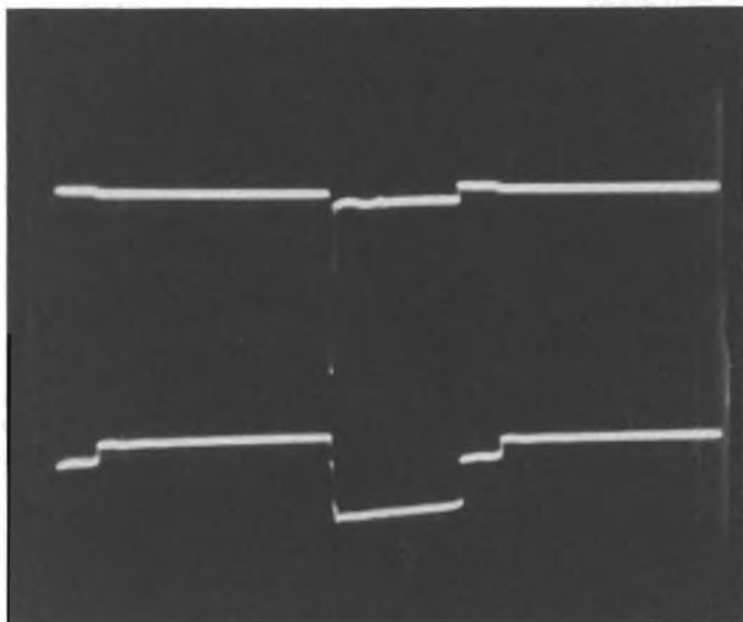
Fig. 11 - Andamento dell'impulso di comando di base del transistore finale di riga BU189. (in alto): corrente di base 200 mA/div. (in basso) tensione di base 5 V/div. Scala dei tempi 10 \mu s/div.
