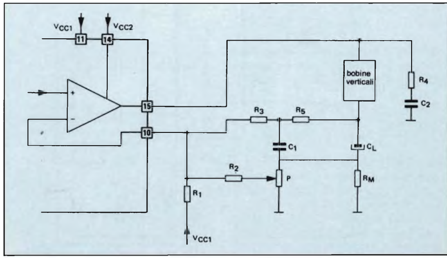
Fig. 7 - Oscillatore e stadio finale di quadro.
