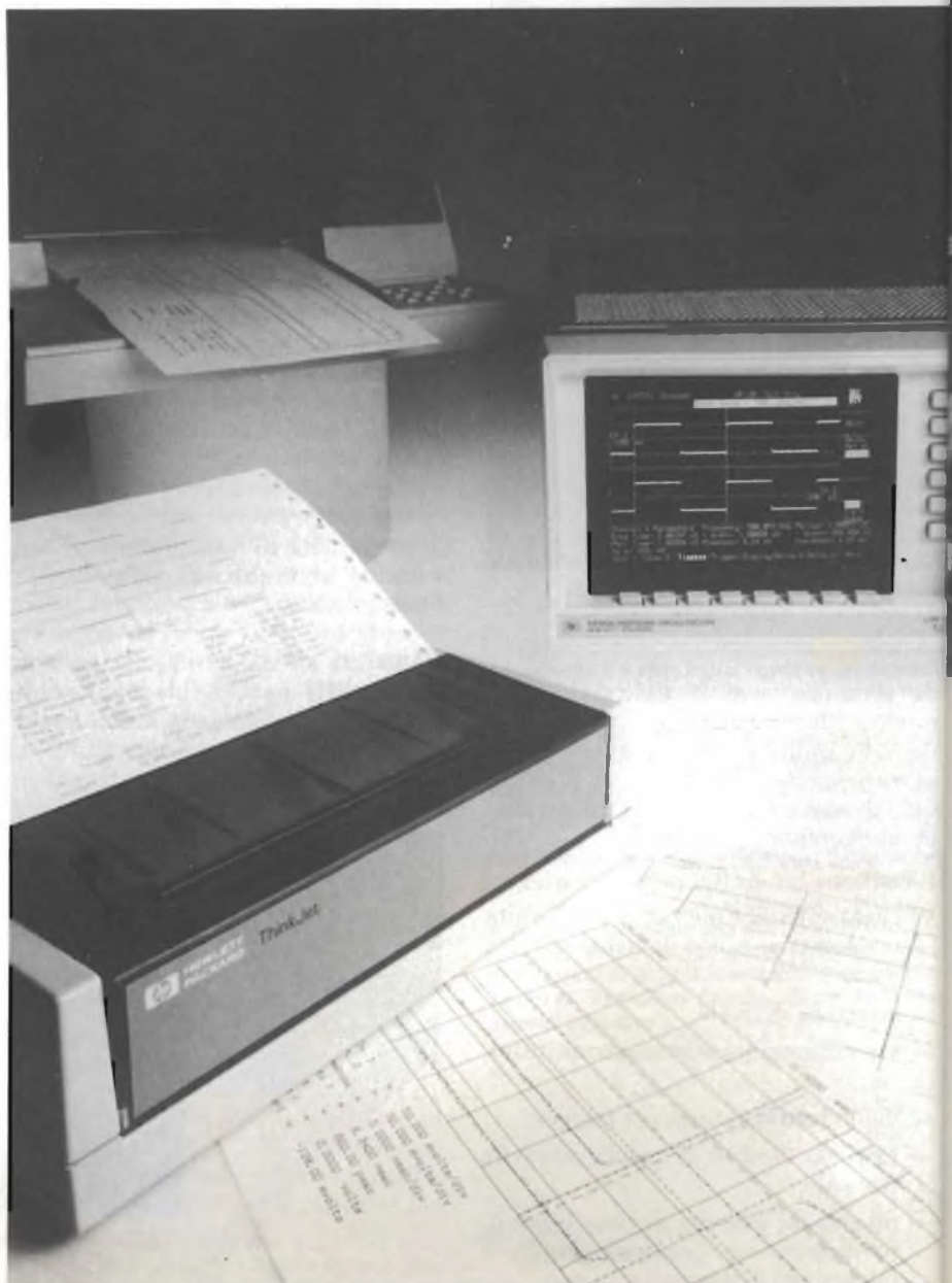
Fig. 2 - Con l'accoppiata HP 54100 A/D e il doppio multiplexer HP 54300A è possibile incrementare la versatilità del sistema. È possibile infatti collegare contemporaneamente allo stesso circuito che si sta esaminando, fino a 16 sonde, e esaminarne la risposta una alla volta.
