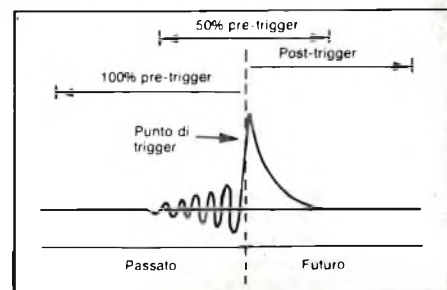
Fig. 4 - La percentuale di pre-trigger può essere impostata a qualsiasi valore compreso fra 0 (post-trigger) e 100%. Nella figura sono esemplificati i valori 50 e 100% di pre-trigger.
