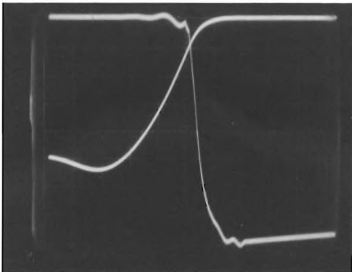
Fig. 13 - Tempo di bloccaggio (turn-off) del transistor di potenza BU 189. Scala dei tempi: 0,5 \mu s/div.
