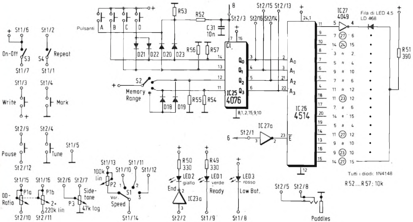
Fig. 9 - La scheda frontale contiene i comandi e gli indicatori.
