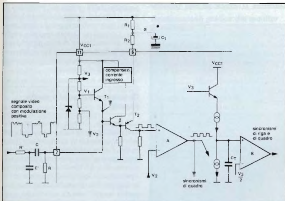
Fig. 2 - Circuiti che effettuano la separazione dei segnali di sincronismo e rispettivamente di riga e di quadro dal segnale video composto positivo.
