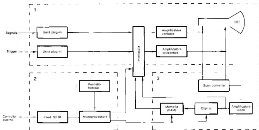
Fig. 5a - Schema a blocchi del modello ibrido della Iwatsu, TS-8123. Il blocco 1 racchiude i circuiti convenzionali, il blocco 2 i circuiti di controllo mentre il blocco 3 contiene i circuiti di memorizzazione.
