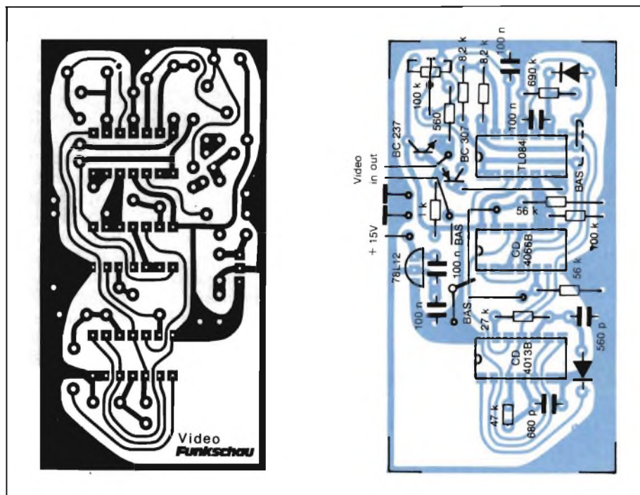
Fig. 4 - Circuito stampato dell'invertitore visto dalla parte del rame, e dalla parte dei componenti. Il circuito deve essere alimentato con una tensione stabilizzata da 12 V (ottenuta, per esempio, dal regolatore di tensione 78L12).
