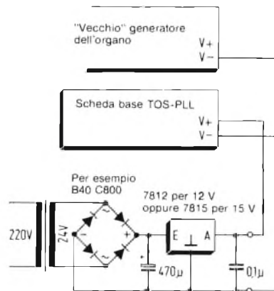
Fig. 14 - Alimentatore supplementare, che dovrà essere utilizzato nel caso l'alimentatore interno si riveli insufficiente.
