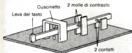
Fig. 2 - Un "wabblers", il cui nome deriva dal fatto che la leva deve essere mossa lateralmente.
