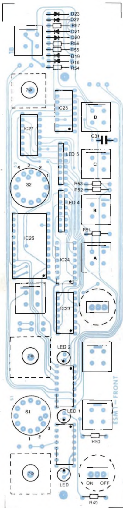
Fig. 13 - Disposizione dei componenti sul circuito stampato frontale, con tutti gli elementi di comando e gli indicatori.
