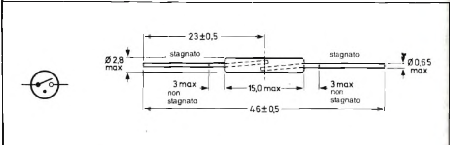
Fig. 1 - Struttura di principio di un microinterruttore reed e relativo simbolo (il puntino nero indica presenza di gas all'interno del bulbo di vetro).
