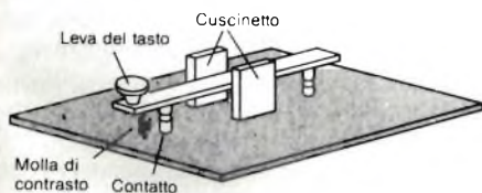
Fig. 1 - Modello originale del tasto Morse classico.
