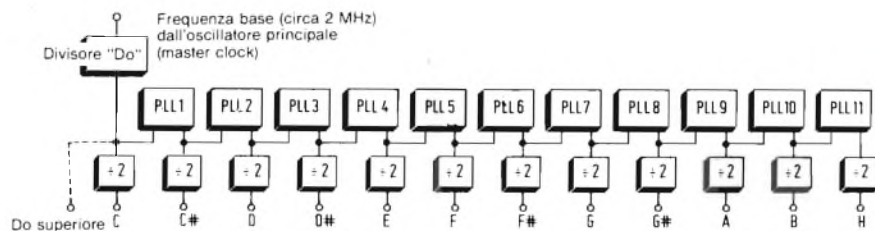
Fig. 6 - Schema a blocchi completo del sintetizzatore di ottava superiore a PLL.
