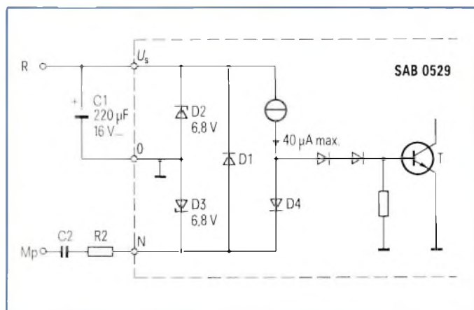
Fig. 3 - Circuito interno del SAB 0529 in corrispondenza dell'ingresso N.
