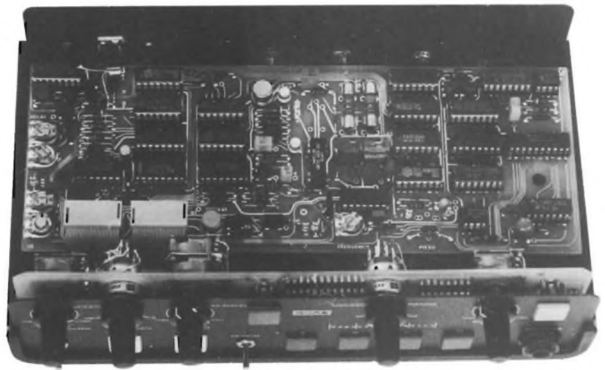
Fig. 14 - Fotografia del prototipo, che mostra la costruzione compatta: le saldature dovranno essere effettuate con molta attenzione, usando un saldatore a punta fine.
