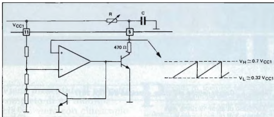
Fig. 4 - Circuito dell'oscillatore di riga.
