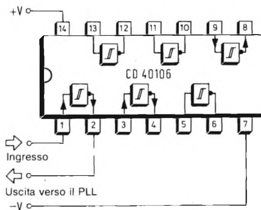
Fig. 13 - Circuito di trigger: se necessario, questo circuito dovrà essere costruito con il componente integrato CMOS 40106.
