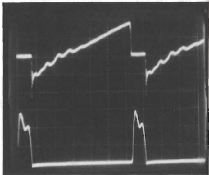
Fig. 12 - Andamento delle correnti (in alto) e delle tensioni (in basso) nel transistore finale di riga BU189. 2 A/div. — 100 V, div. scala dei tempi: 1 \mu s/div.
