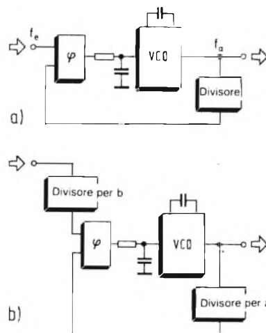
Fig. 1 - Schemi di principio di un moltiplicatore di frequenza (a) e del circuito adatto a rappresentare un rapporto a/b qualsiasi.
