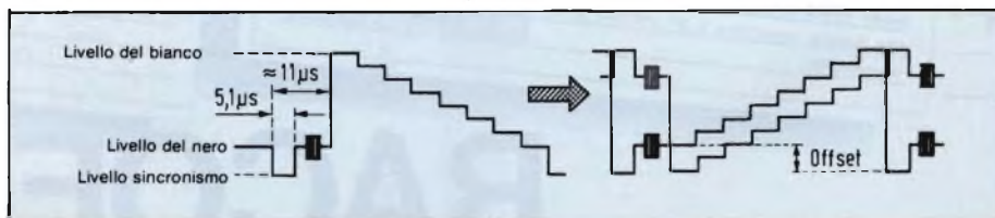
Fig. 1 - Inversione del segnale video richiesta per riprodurre sullo schermo di un monitor testi bianchi su fondo nero. Il segnale video (a sinistra) dopo essere stato invertito, corrisponderebbe a quello (a destra), che presenta un errore di livello (offset). L'inversione però deve riguardare solo il segnale video e non il livello del sincronismo e del nero.
