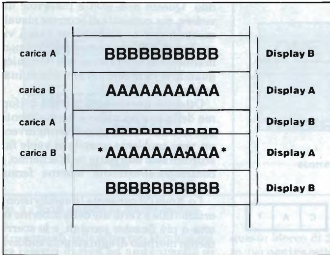
Fig. 7 - Scroll morbido su finestre multiple: normali CRTC con 2 buffer di riga.
