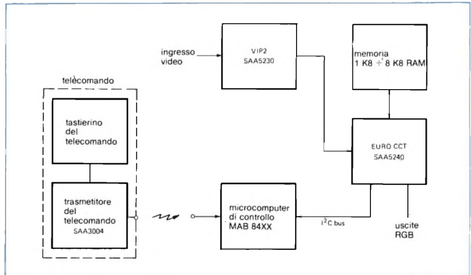
Fig. 4 - Schema a blocchi di decodificatore basato sull'integrato EURO-CCT SAA5240.
