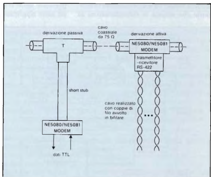
Fig. 2 - Derivazioni attive e passive sul cavo coassiale. Le prese attive utilizzano un trasmettitore e un ricevitore RS-422 per comunicare con le periferiche distanti dal cavo.
