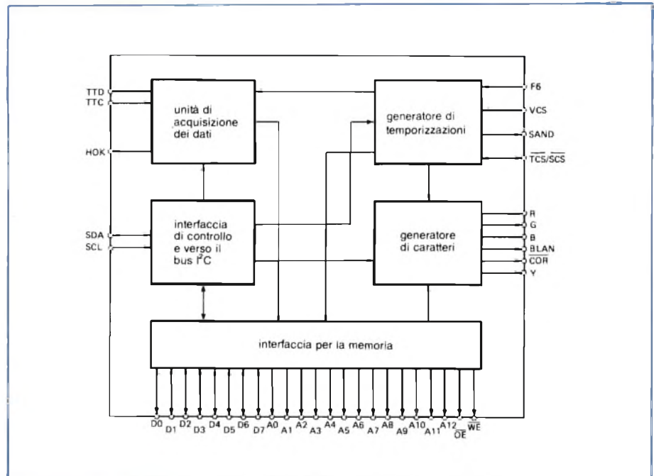
Fig. 6 - Schema a blocchi dell'EURO-CCT SAA5240.
