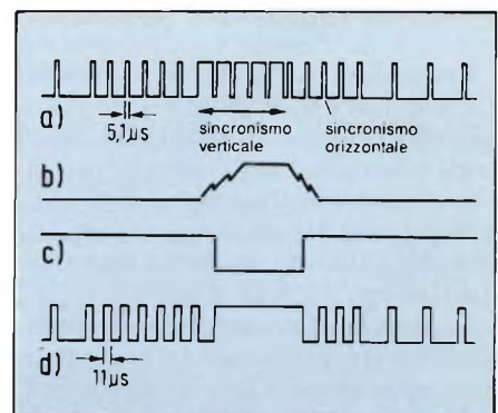
Fig. 3 - Formazione dei segnali destinati al comando dei due interruttori analogici. I segnali di comando sono i segnali c) e d), derivati dai normali impulsi di sincronismo.
