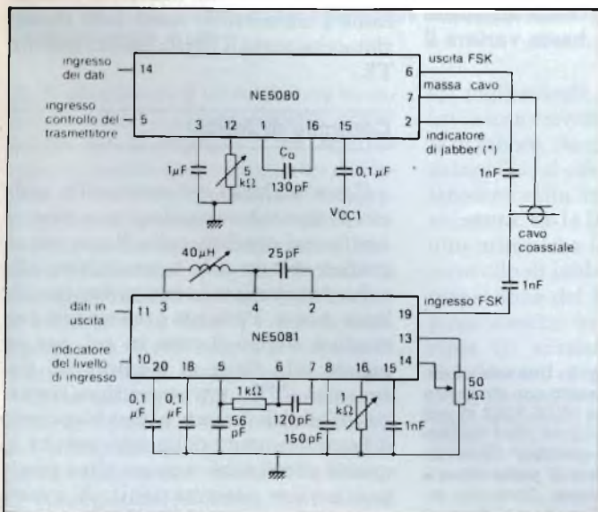
Fig. 1 - Esempio di utilizzazione dell'NE5080 e dell'NE5081 come modem FSK in semi-duplex. Con i componenti esterni indicati il modem lavora a una frequenza portante di 5 MHz e con dati fino a 2 Mbit/s.
