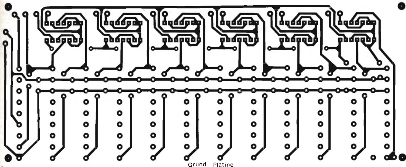
Fig. 9 - Scheda base, sulla quale sono inseriti i divisori, il divisore "do" innestabile ed i moduli PLL.
