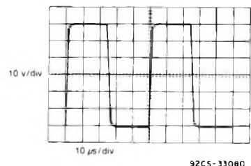
Fig. 2 - Risposta dell'amplificatore ad una forma d'onda rettangolare con frequenza di 20 kHz.
