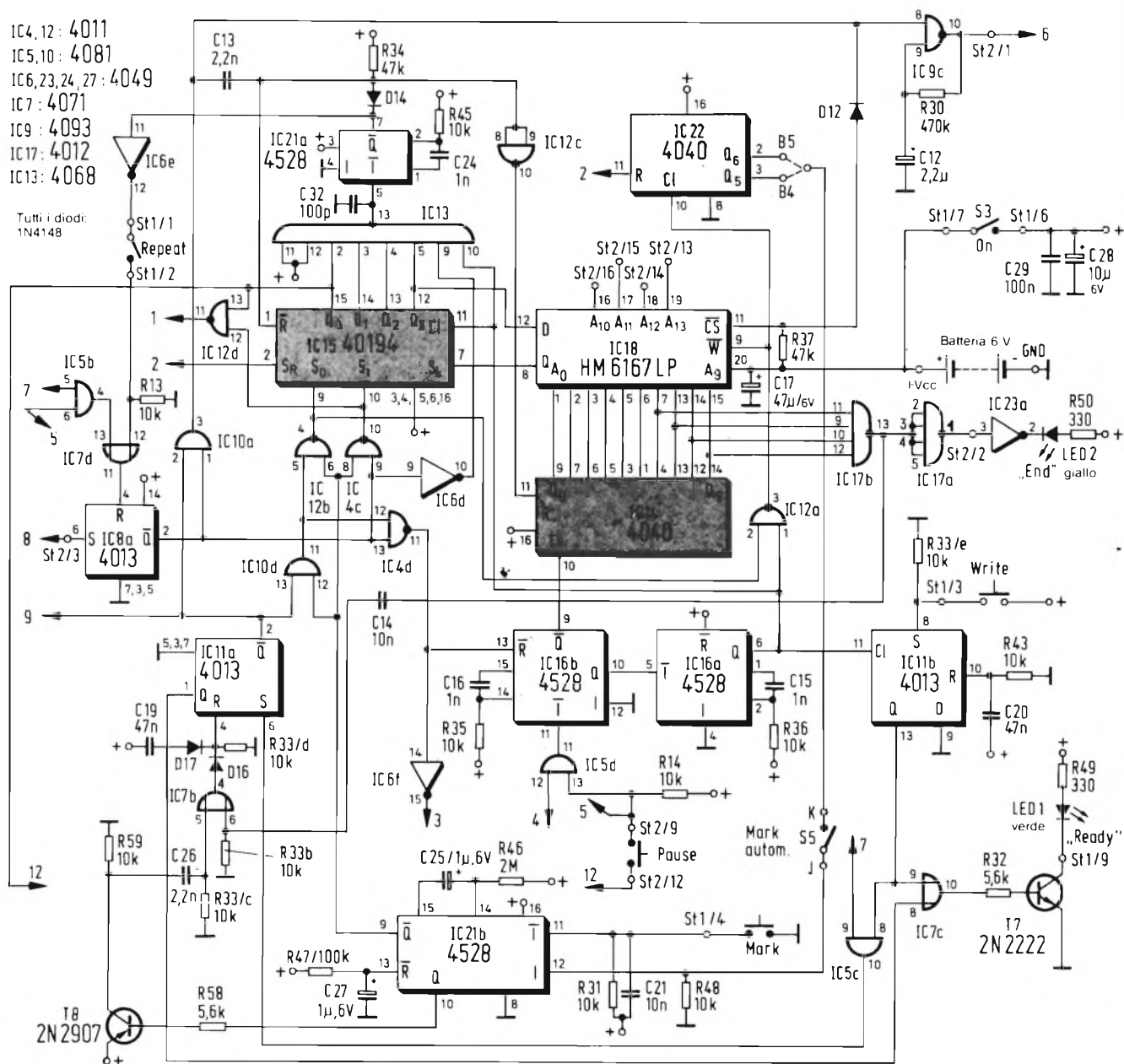
Fig. 8 - Il circuito elettronico della memoria è il nucleo di questo apparecchio: nelle 16 sezioni di memoria potranno essere inseriti testi standard qualsiasi.
