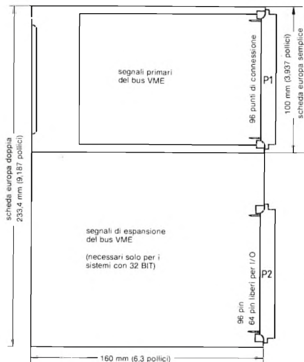
Fig. 1 - Bus VME su scheda europea semplice e doppia.
