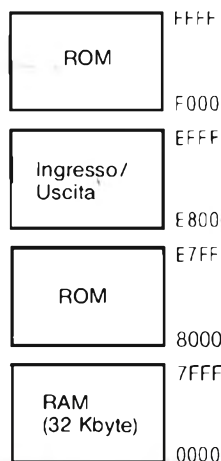
Fig. 1 - Configurazione dello spazio di memoria del computer CBM-4032.
