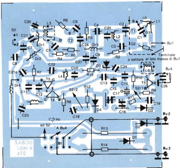
Fig. 3 - Disposizione dei componenti sul circuito stampato del convertitore: attenzione alle necessarie schermature interne. Questo circuito dovrà essere inoltre inserito in un astuccio metallico di schermo.
