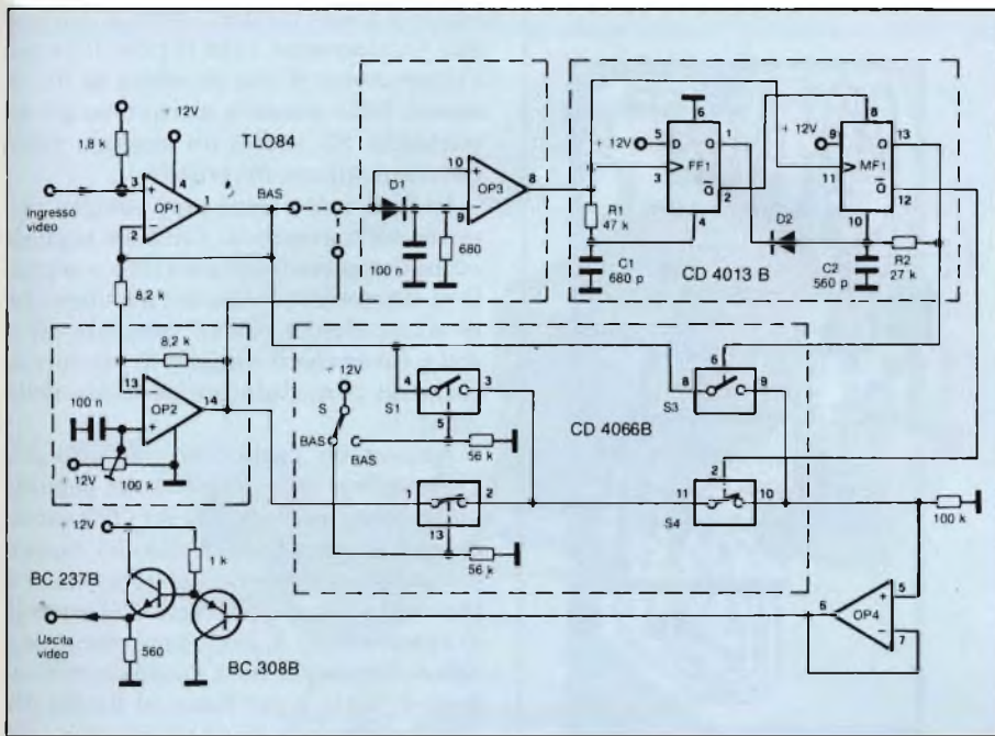
Fig. 2 - Circuito che effettua l'inversione del solo segnale video e mantiene inalterata la polarità del livello del nero e dei sincronismi. Trattandosi di una elaborazione di natura analogica, il circuito può invertire segnali video provenienti dalle sorgenti più disparate come computer, telecamere e videoregistratori a colori senza soppressione dei grigi. Venendo attenuata la portante del colore, i colori riprodotti risultano un po' scialbi.
