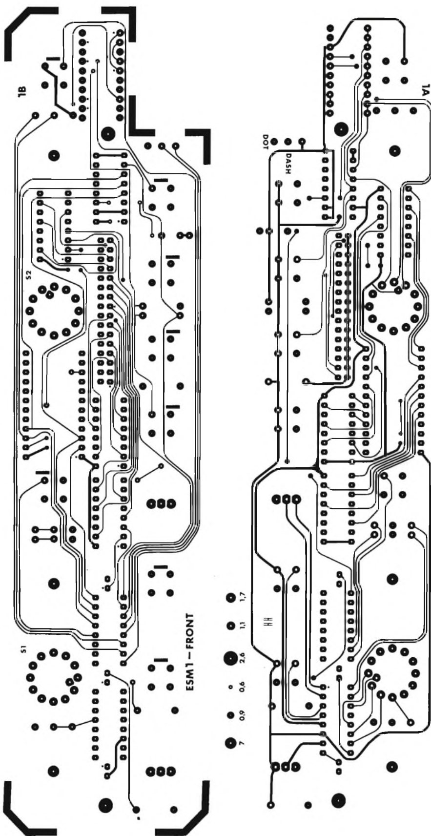
Fig. 10 - Circuito stampato principale in grandezza naturale. Per garantire la sicurezza del funzionamento, è necessario impiegare un circuito stampato a doppia faccia incisa, con fori metallizzati (vedi elenco dei componenti).
