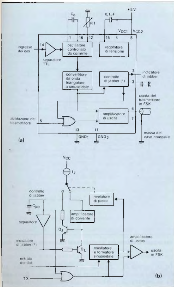
Fig. 4 - (a) Schema a blocchi del trasmettitore NE5080; (b) buffer di uscita e controllo di jabber.
