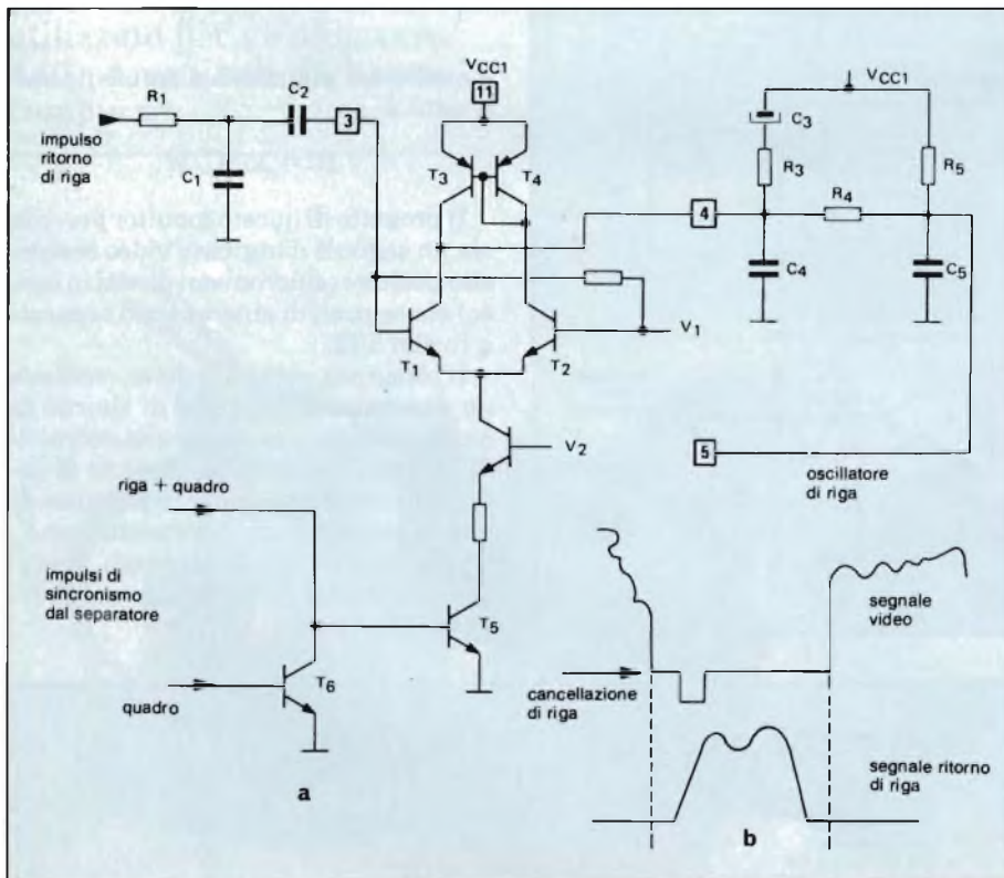
Fig. 5-a) Circuito del comparatore di fase; b) segnali presenti sul comparatore di fase.
