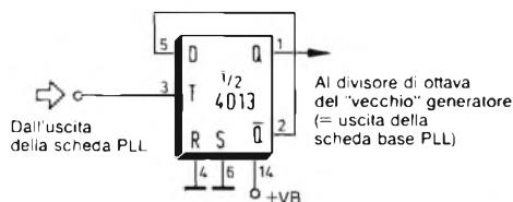
Fig. 10 - Divisore per due della frequenza: le frequenze dei segnali d'uscita delle schede PLL devono essere ancora dimezzate.
