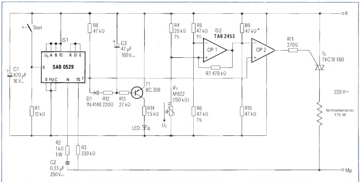
Fig. 9 - Schema di un sistema di regolazione di temperatura temporizzato nel quale un LED indica le condizioni di funzionamento del circuito.
