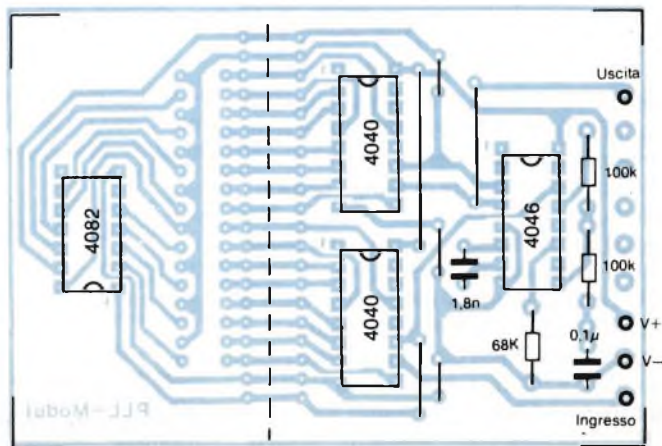
Fig. 4 - Disposizione dei componenti sul modulo PLL. Il circuito stampato può essere diviso in corrispondenza alla linea tratteggiata, montando poi una spina ed una presa lineare per la connessione, in modo da non dover sostituire l'intera scheda in caso si voglia modificare la programmazione.
