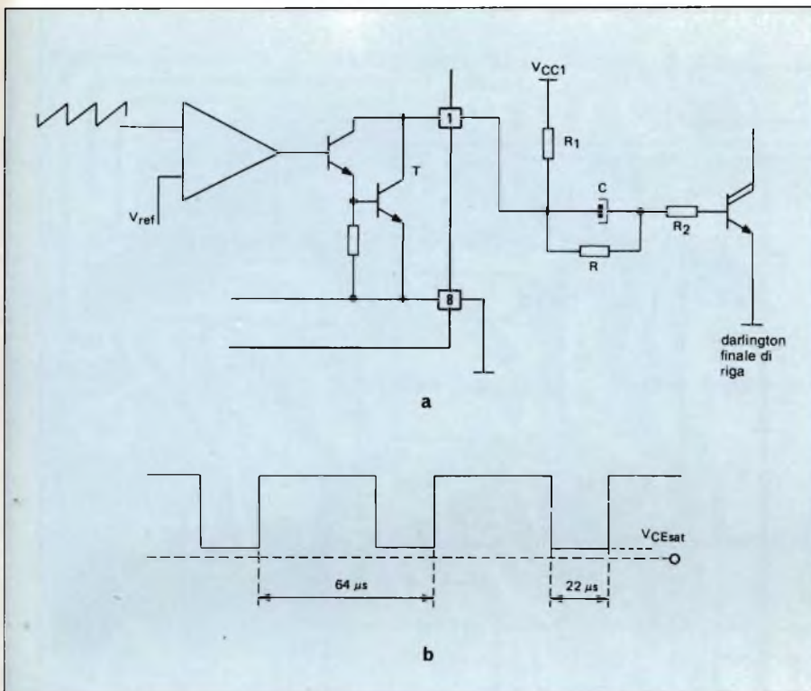
Fig. 6-a) Generatore d'impulsi e stadio d'uscita orizzontale. b) segnale d'uscita al terminale 2.
