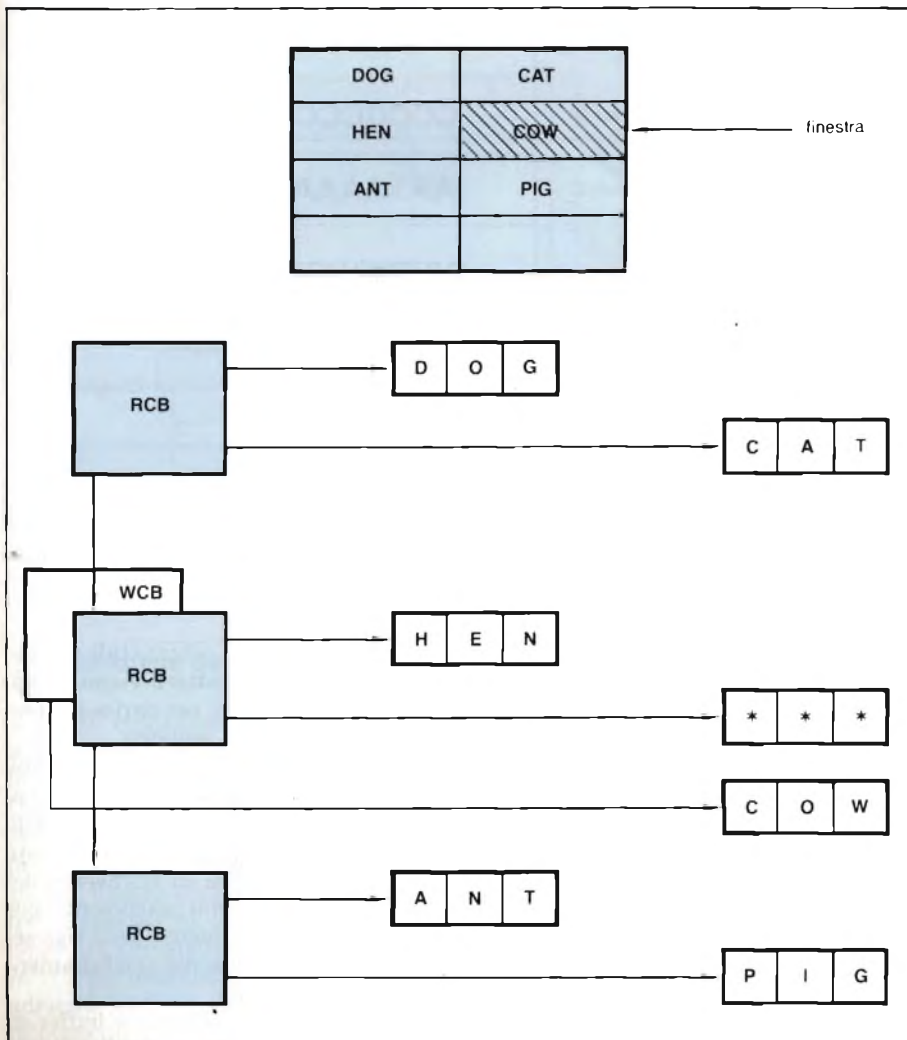
Fig. 6 - Esempio di finestra video. WCB = Window Control Block, equivalente per le finestre video dell'RCB (vedi testo).
