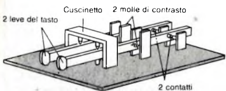
Fig. 3 - Un tasto "squeeze" ha due levette (paddle) che necessitano di un minimo movimento delle mani durante la manipolazione.
