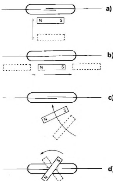
Fig. 5 - Vari sistemi di apertura/chiusura di un microinterruttore reed realizzabili nel caso in cui il campo magnetico sia prodotto da un magnete permanente.
