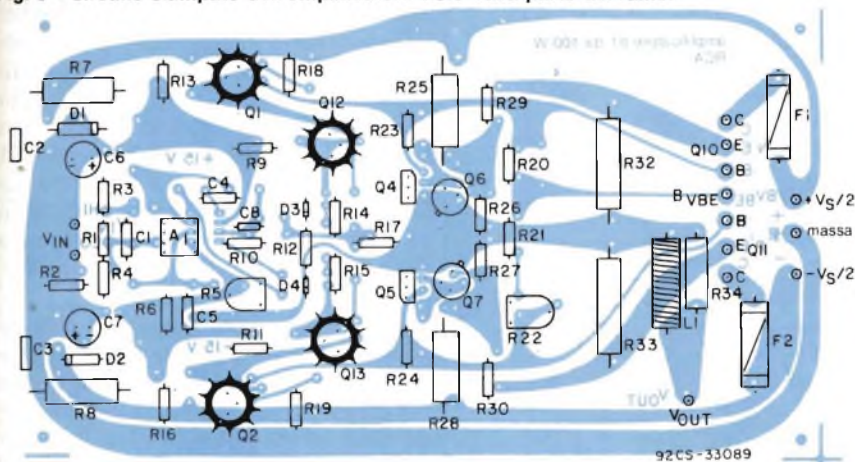
Fig. 3 - Circuito stampato dell'amplificatore visto dalla parte del rame.
