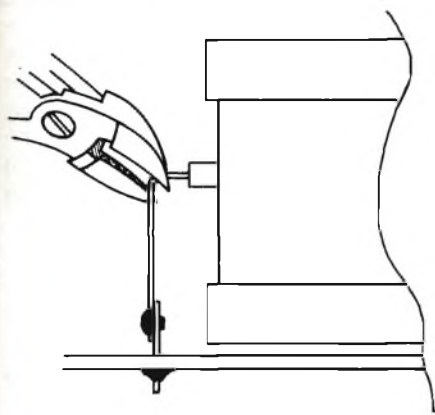
Fig. 15 - Troncatura dei conduttori di uscita del "vecchio" TOS, necessaria in alcuni tipi di organo.
