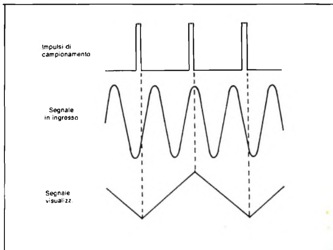
Fig. 3 - La figura mostra come, se i punti di campionatura sono insufficienti, un segnale sinusoidale venga visualizzato come un'onda triangolare avente differente periodo.
