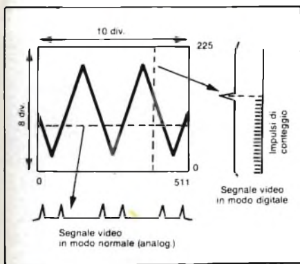
Fig. 6 - Sono illustrati i due diversi modi di prelievo del segnale video, durante il funzionamento normale (analogico) e digitale dell'oscilloscopio ibrido della Iwatsu.
