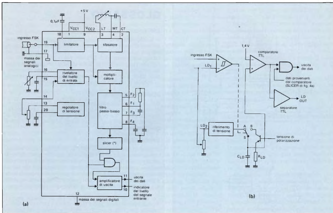
Fig. 5 - (a) Schema a blocchi del ricevitore NE5081; (b) rivelatore del livello del segnale in entrata per la reiezione del rumore e la selezione della gamma dinamica.
