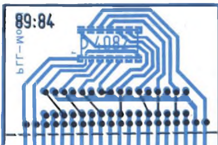
Fig. 5 - Programmazione mediante ponticelli dei diversi rapporti di divisione del modulo PLL.
