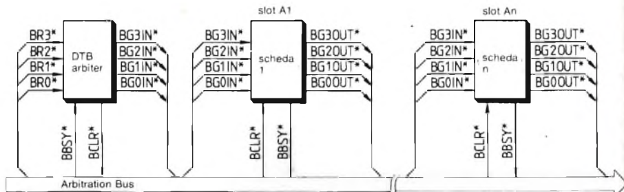
Fig. 7 - Diagramma funzionale relativo all'arbitrazione del DTB.
