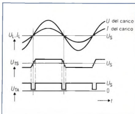
Fig. 5 - Segnali relativi al modo di funzionamento "sincronizzazione in tensione".
