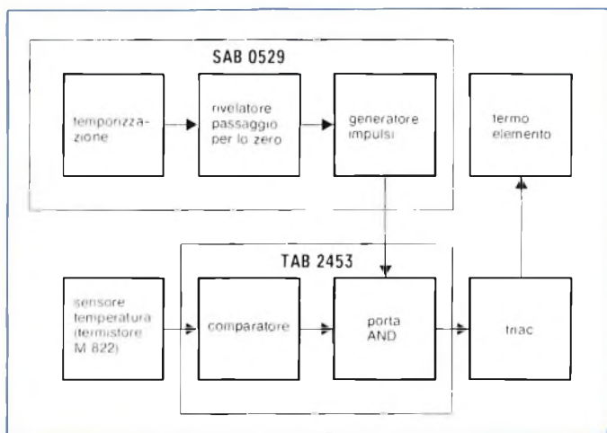
Fig. 1 - Schema a blocchi di un sistema di temporizzazione di un dato valore di temperatura.
