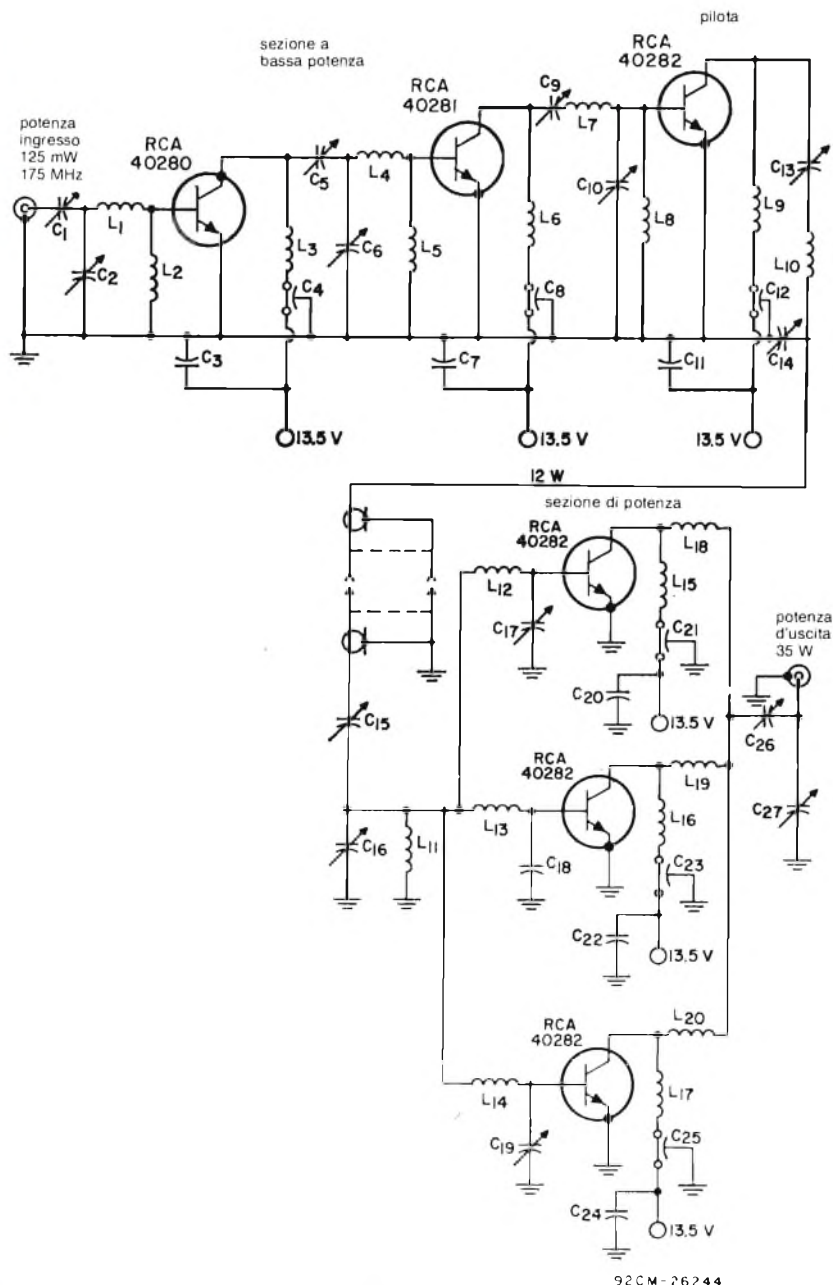
Fig. 1 - Schema elettrico dell'amplificatore da 175 MHz e potenza d'uscita di 35 W.
