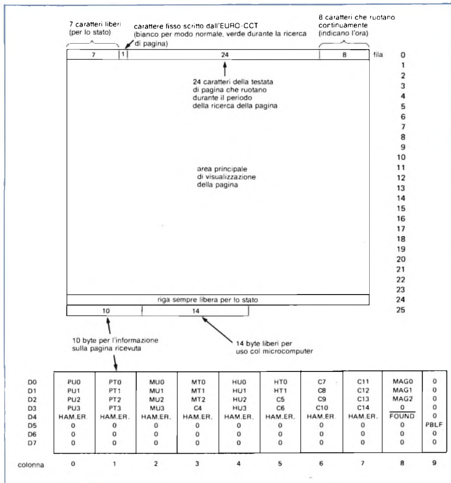
Fig. 7 - Organizzazione della memoria video nel decodificatore EURO-CCT.
