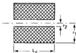
Fig. 4 - Struttura di principio della bobina di eccitazione di un microinterruttore reed.
