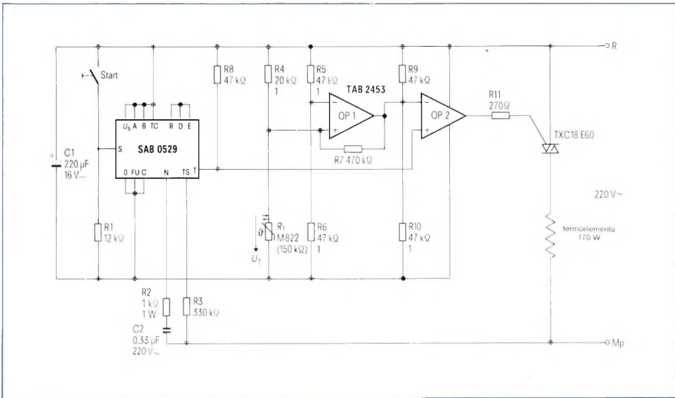
Fig. 2 - Schema del circuito utilizzato per mantenere un dato processo ad una data temperatura e per un tempo determinato (in questo caso, 30 minuti a 70 °C).
