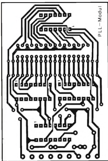
Fig. 3 - Circuito stampato di un modulo PLL, che contiene il circuito di figura 2.
