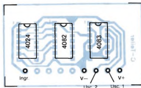
Fig. 12 - Disposizione dei componenti sul divisore per due della frequenza.
