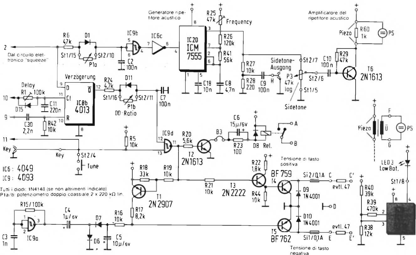
Fig. 7 - Schema del circuito elettronico del tasto, che adatta i segnali provenienti dal tasto "squeeze" al pilotaggio del radiotrasmittitore.
