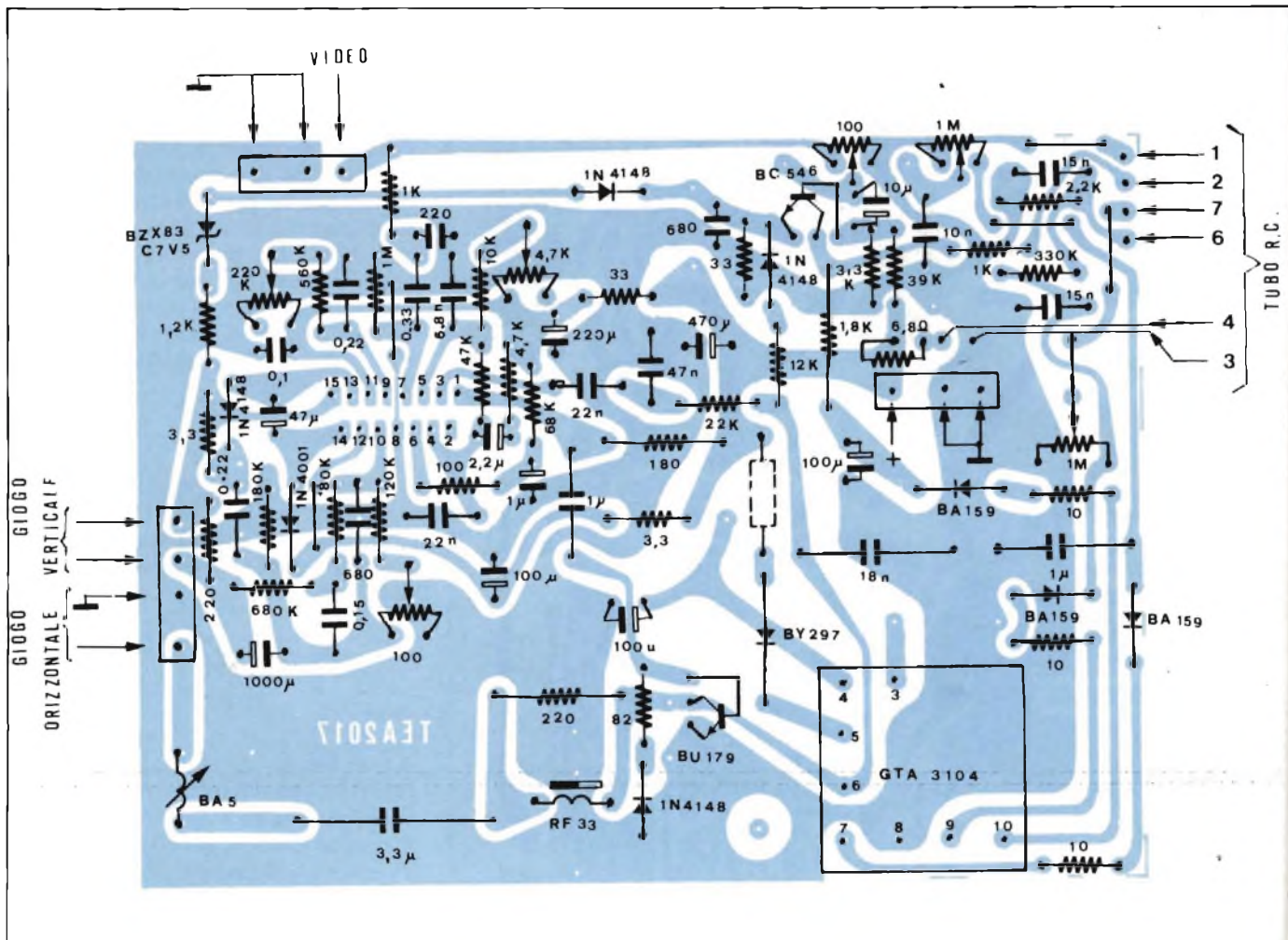
Fig. 10 - Circuito stampato del monitor visto dalla parte dove sono montati i componenti.
