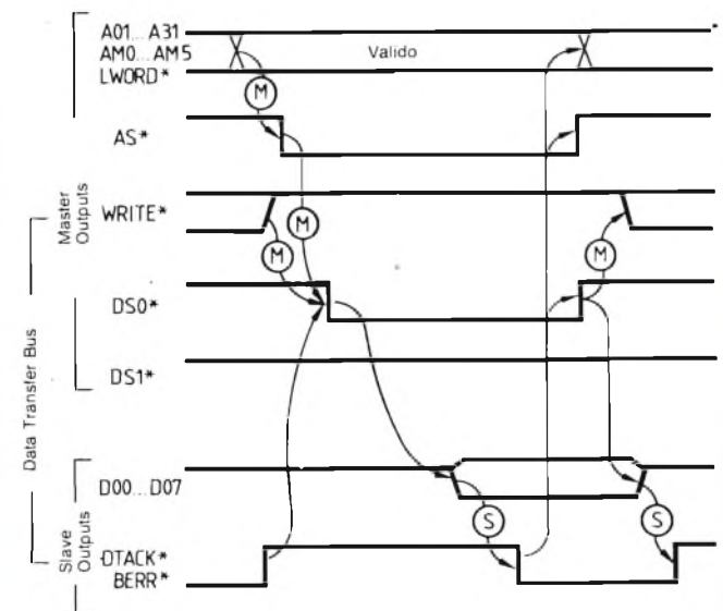
Fig. 5 - Lettura di un byte sul DTB. Il segno * dopo il nome di un segnale significa che questo è attivo al livello basso. Le frecce con il segno M indicano relazioni di tempo garantite dalla temporizzazione interna del MASTER; le frecce con il segno S indicano relazioni di tempo garantite dalla temporizzazione interna dello SLAVE.
