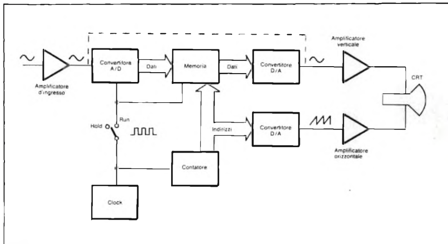
Fig. 2 - Schema a blocchi di un oscilloscopio digitale. La linea tratteggiata mostra il percorso del segnale nel caso si escluda la memorizzazione.
