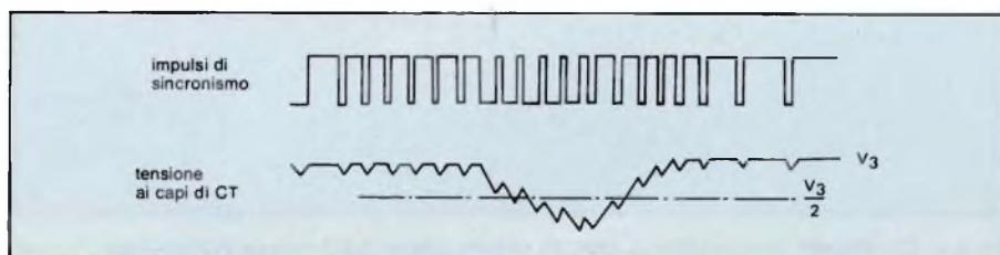
Fig. 3 - Segnali di sincronismo di riga e di quadro separati e corrispondenti tensioni a capi del condensatore C_T .
