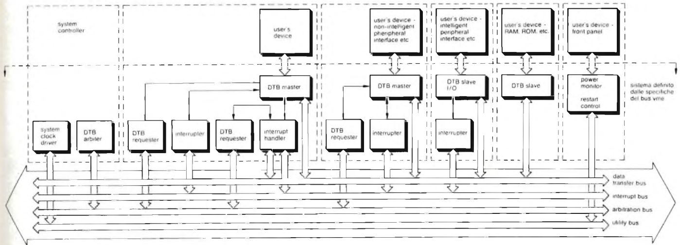
Fig. 3 - Suddivisione funzionale di un sistema secondo il bus VME.
