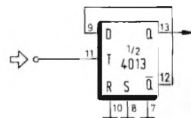
Fig. 10 - Divisore per due della frequenza: le frequenze dei segnali d'uscita delle schede PLL devono essere ancora dimezzate.
