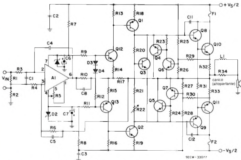
Fig. 1 - Schema elettrico dell'amplificatore audio con potenza d'uscita di 100 W. L'elenco completo dei componenti è riportato nella tabella 3.
