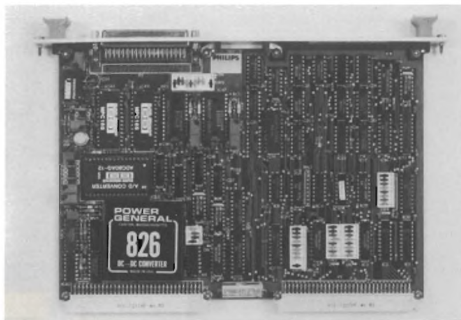
Una delle molte schede VMEbus prodotte dalla Philips/Signetics (modulo I/O analogico programmabile PG 3652). Questa società ha diviso le sue schede VMEbus in 7 categorie, e precisamente: 6 schede per l'elaborazione centrale dei dati; 2 schede di memoria; 2 schede per il controllo del sistema; 1 scheda per il controllo delle periferiche; 2 schede comunicazione dati; 3 schede I/O; schede sottosistemi industriali I/O; sistemi di assemblaggio. Il numero delle schede di ciascuna categoria è in continuo aumento allo scopo di soddisfare le esigenze di qualsiasi sistema di elaborazione e controllo industriale
