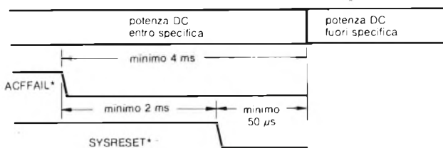
Fig. 11 - Temporizzazione relativa alla caduta della tensione di rete.
