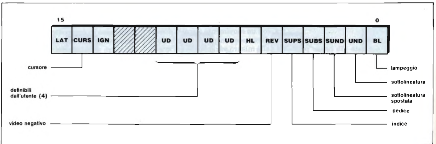
Fig. 9 - Organizzazione delle parole di attributi video.
