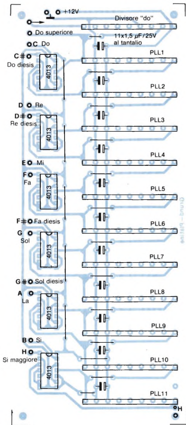
Fig. 11 - Disposizione dei componenti sulla scheda base, comprese tutte le schede inseribili.
