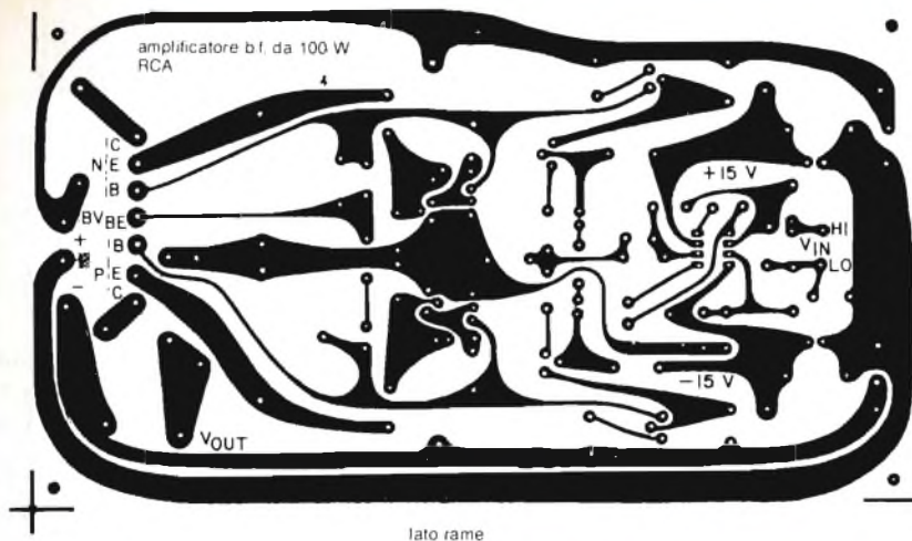
Fig. 3 - Circuito stampato dell'amplificatore visto dalla parte del rame.
