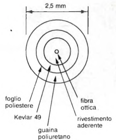
Fig. 11 - Tipico cavo in fibra ottica per trasmissione dati. Da notare il tipo di rivestimento "aderente" ed il ridotto diametro esterno.
