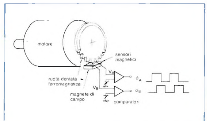
Fig. 2 - Encoder a riluttanza.
