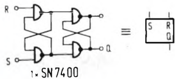
Fig. 5 - Schema elettrico del circuito eventualmente necessario per eliminare i rimbalzi dei contatti.
