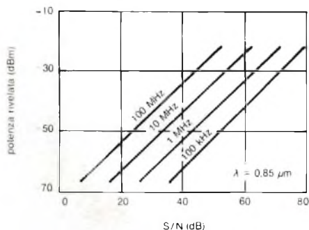
Fig. 7 - Grafico che mostra la relazione fra la sensibilità, il rapporto segnale/disturbo e la banda passante di un rivelatore ottico, relativamente alla lunghezza d'onda di 0,85 \mu\text{m} .
