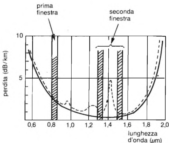
Fig. 4 - Diagramma di attenuazione delle fibre ottiche, in funzione della lunghezza d'onda impiegata. Si notino i tre picchi di assorbimento dovuti allo ione OH (linea tratteggiata). La linea continua indica l'andamento teorico.
