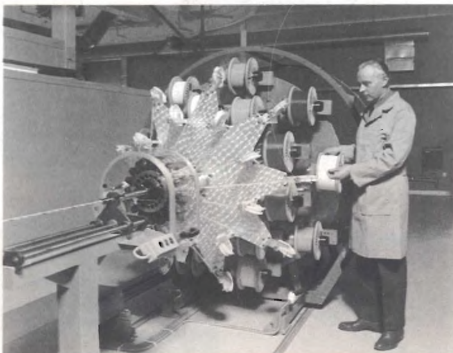
Produzione di un cavo in fibra ottica alla Ericsson, rappresentata in Italia dalla RACOEL.
