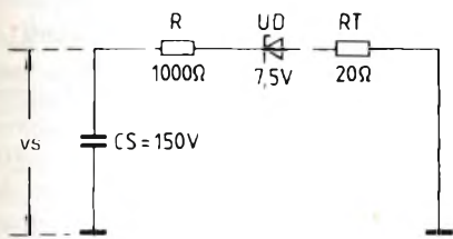
Fig. 3 - Circuito equivalente di una scarica elettrostatica in un transistor NPN.
