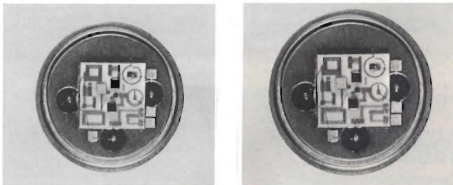
Fig. 1 - Moduli oscillatori TO 5502 in contenitore TO-8 e F 57529 accordabili mediante varactor. Le frequenze di accordo possono andare da 2100 a 2600 MHz. Sono destinati principalmente alle applicazioni in banda E.
