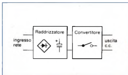
Fig. 2 - Il convertitore fraziona una tensione continua ottenuta previo raddrizzamento della tensione della rete.
