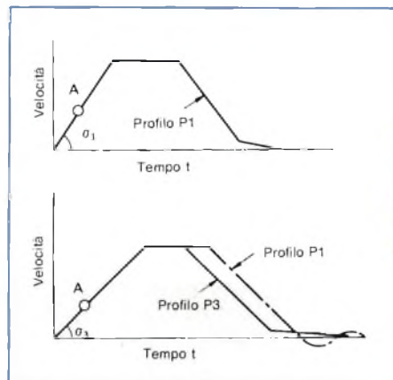
Fig. 7 - Adattamento della decelerazione al carico applicato.
