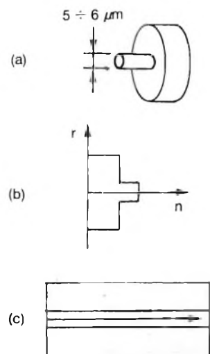
Fig. 9 - Fibra ottica monomodo. Il nucleo di questa fibra ha un diametro molto piccolo, comparabile con la lunghezza d'onda della luce impiegata (a). L'indice di rifrazione del nucleo è costante (b), mentre in (c) viene evidenziato il modo di procedere dei raggi all'interno della fibra.
