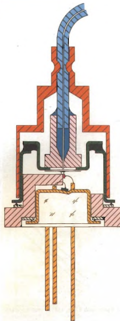
Diodo laser Ga-Al-As tipo 375 CQY accoppiato a fibra ottica (50/125 \mu\text{m} ) prodotto dalla Philips. Può lavorare su lunghezze d'onda da 780 a 880 nm. Si presenta in un contenitore TO-5 modificato. Strutturalmente è identico al tipo 502 CQF. Anch'esso possiede "pig-tail".
