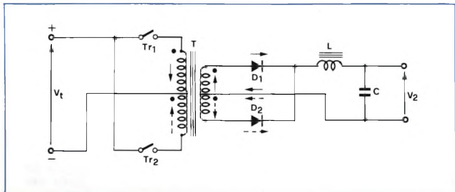
Fig. 5 - Schema di principio di un alimentatore push-pull.
