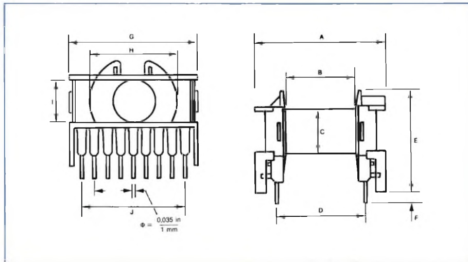
Fig. 9 - Carcassa a corredo dei nuclei ETD. Le dimensioni sono riportate nella tabella 3.
