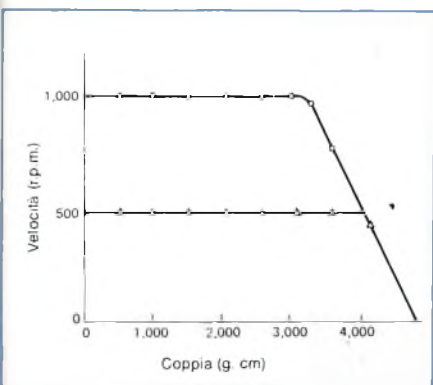
Fig. 6 - Caratteristica velocità/coppia.
