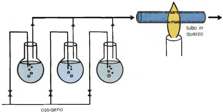
Fig. 8 - Processo schematico CVD (Chemical Vapor Deposition) usato per produrre fibre del tipo "graded index". Le ampolle contengono i vari elementi chimici per ottenere strati di vetro con diverso indice di rifrazione (per cortesia RIFA-RACOEL).
