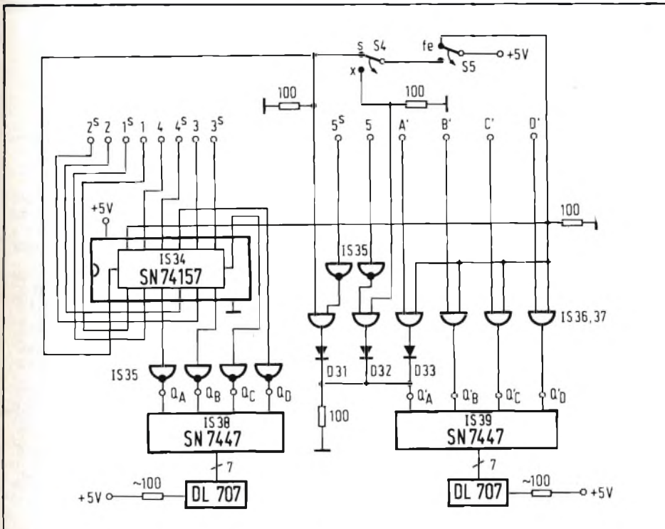
Fig. 9 - Schema dell'unità di visualizzazione
