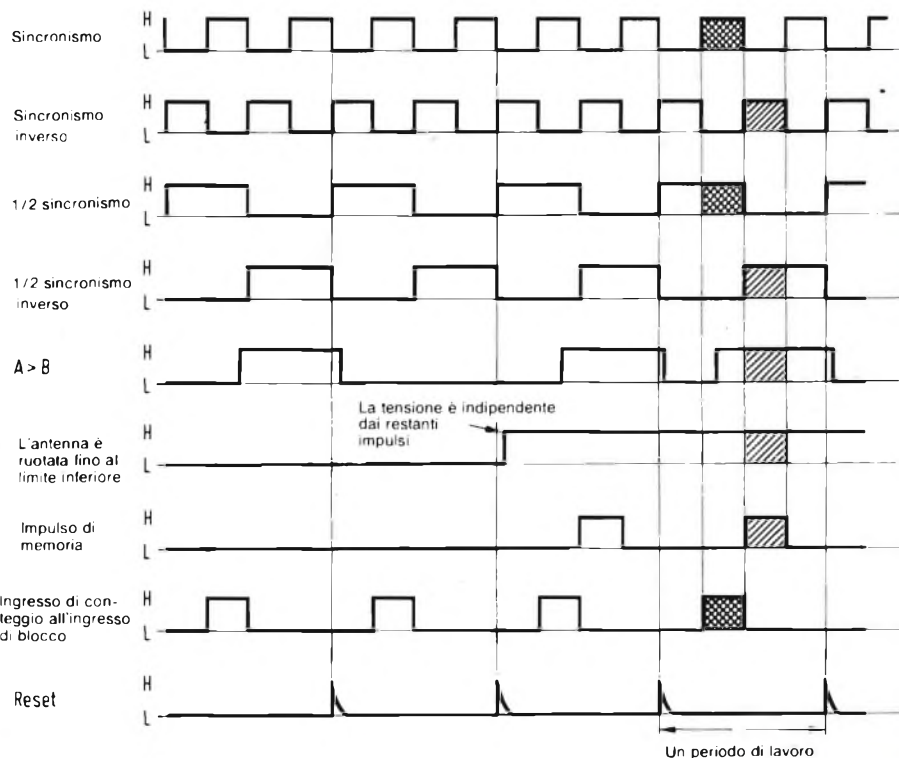
Fig. 3 - Diagramma degli impulsi.
