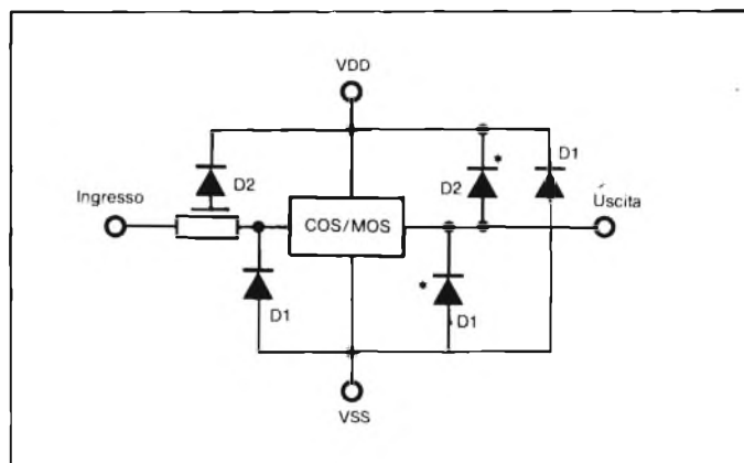
Fig. 1 - Rete di protezione standard incorporata in tutti i CMOS RCA (COS/MOS) serie A e B. I diodi contrassegnati con asterisco vengono formati in fase di produzione del dispositivo. La tensione di rottura di D1 è circa 25 V, quella di D2, circa 50 V.
