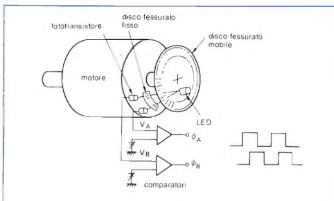
Fig. 1 - Encoder ottico.
