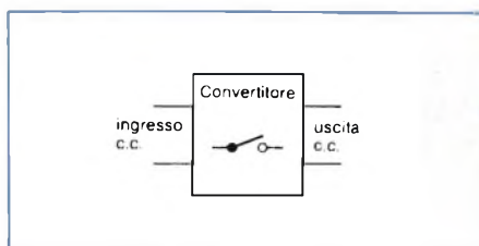
Fig. 1 - Il convertitore fraziona una tensione continua (batteria).
