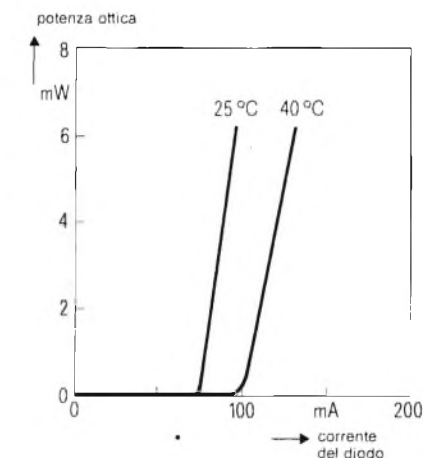
Fig. 6 - Caratteristiche potenza/corrente diretta di un diodo laser In-Ga-As-P, per due differenti temperature (a). Lo spettro, a 25 °C, è molto stretto (b).
