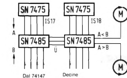
Fig. 14. Questa modifica permette di far ritornare automaticamente l'antenna nella posizione originaria, in caso di spostamenti dovuti al vento.
