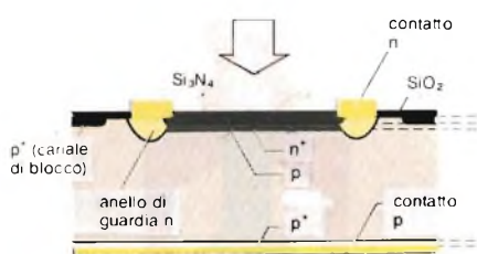
Fig. 9 - Tipica struttura di un fotodiolo ad effetto valanga (APD) al silicio. Lo strato di \text{Si}_3\text{N}_4 costituisce una copertura antiriflessa.
