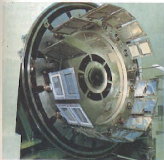
Fig. 10 - Due fasi del processo di produzione e di test dei pannelli elettroluminescenti: a) test di durata di vita; b) la disposizione dei sottili strati degli elettrodi X-Y e dello strato luminescente sul substrato di vetro avviene in camere a vuoto spinto e ad elevata temperatura.
