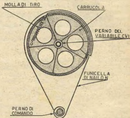
Fig. 4. — Come viene installata la funicella di nylon sulla carrucola della demoltiplicazione.
