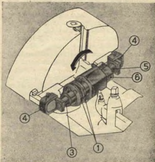
Fig. 4. — Ecco come viene fissato sul tornio l'attrezzo.
