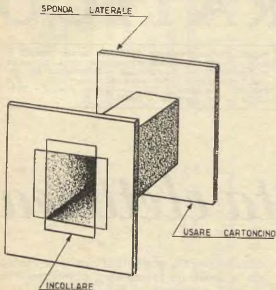
Fig. 2. — Il cartoccio del trasformatore, dovrà essere costruito con del cartoncino sottile e allo stesso tempo robusto. Il cartone presspahn è da ritenersi tra i più indicati.
