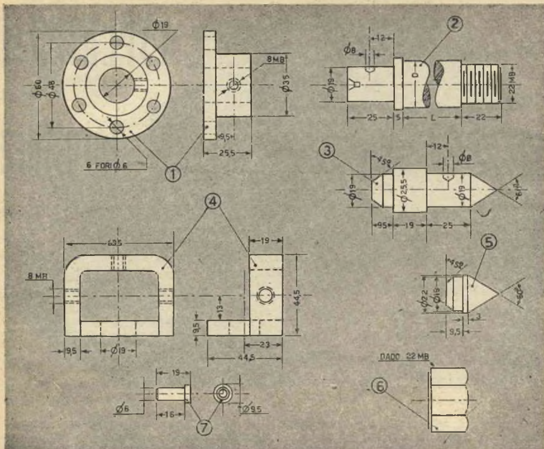
Fig. 2. — In questo disegno sono rappresentati tutti i particolari necessari al complesso. Notare che dei particolari 1 e 4 ne vanno costruiti due esemplari.
