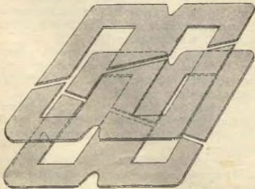
Fig. 3. — I lamierini, per non avere perdite nel trasformatore, vanno incrociati tra di loro.
