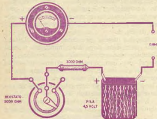
Fig. 7. - Per usare lo strumento come ohmetro si inseriranno così la pila e un potenziometro. Con i valori inseriti è possibile misurare resistenze da 100 a 100.000 ohm.
