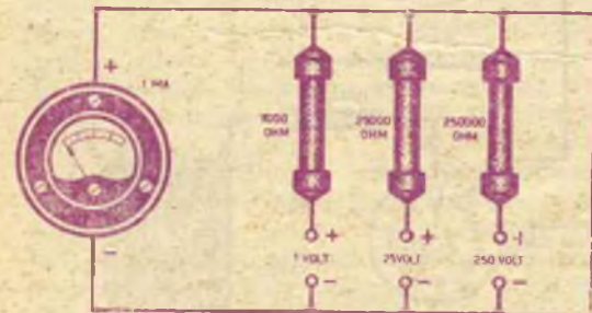
Fig. 4. - Ecco come si presenta un semplice strumento per misurare tutte le tensioni, da 1 a 250 volt, a tre portate.
