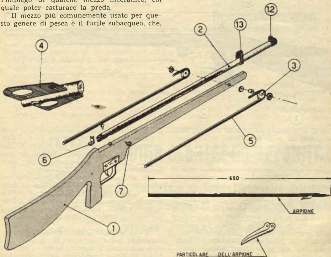
1. Supporto — 2. Canna — 3. Carrucola — 4. Percussore — 5. Elastico — 6. Mirino — 7. Occhiello — 8. Grilletto — 9. Molla a lamina — 10. Perno d'arresto — 11. Boccola — 12. Mirino — 13. Fascetta.
