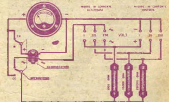
Fig. 6. - Così si presenta uno strumento per il controllo della tensione a corrente continua (C. C.) e a corrente alternata (C. A.). Un semplice interruttore include o esclude il raddrizzatore a seconda che si voglia la corrente continua o alternata.
