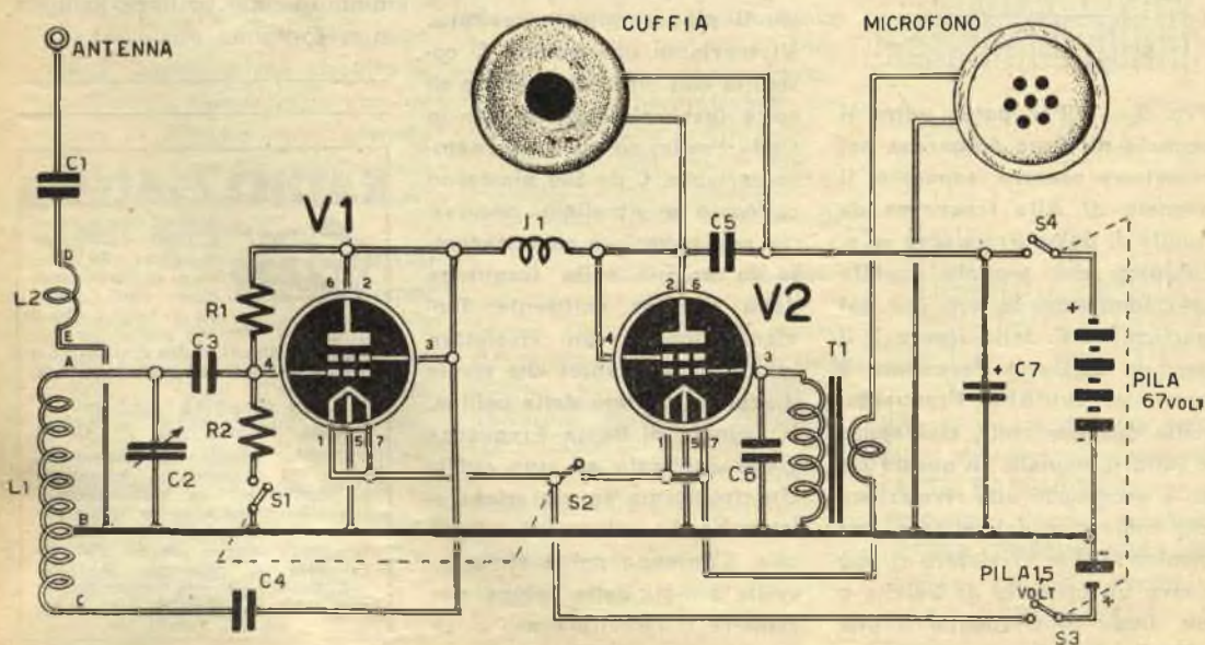
Schema elettrico.
