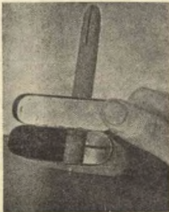
Fig. 3. - Al fine di mantenere dritto l'attrezzo e lavorare così a nostro agio, lo fisseremo ad una piccola scatola seguendo il sistema chiaramente illustrato nella figura.
