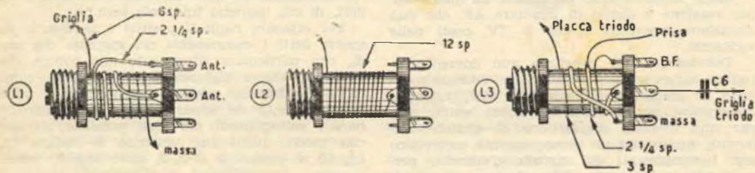
Fig. 3. — Le bobine del ricevitore sono avvolte in piccoli supporti per bobine Microdin. In figura sono visibili a grandezza naturale tali bobine ed il relativo avvolgimento.
