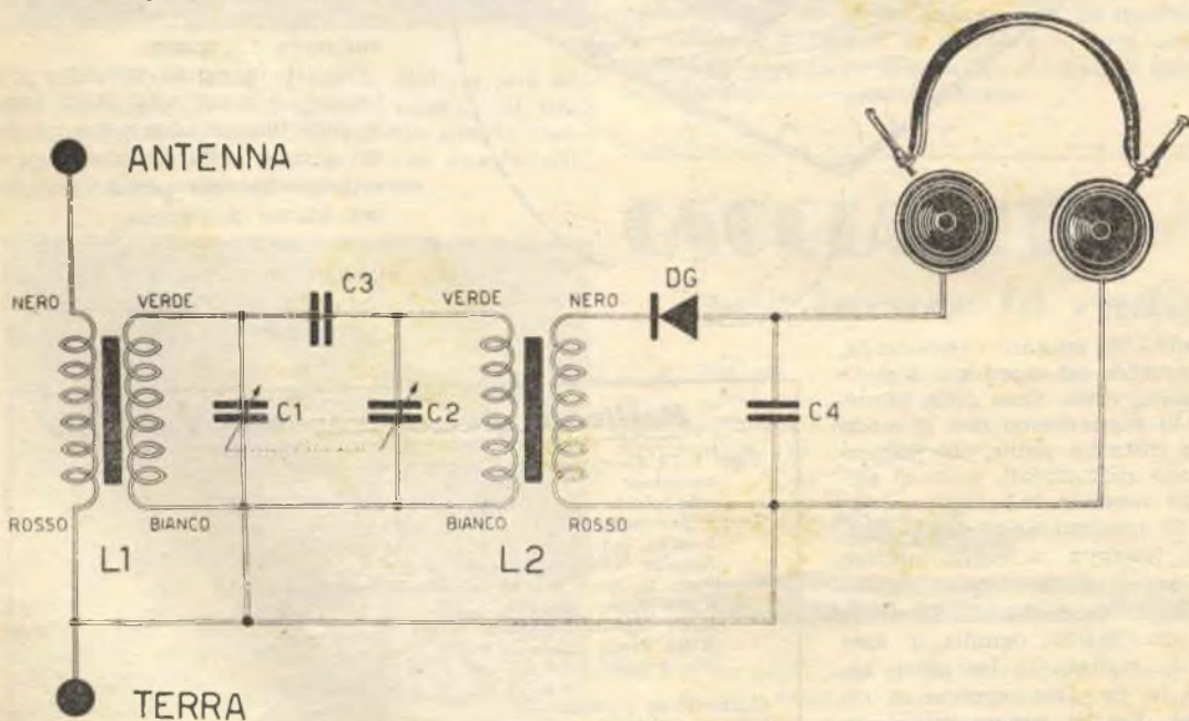
Fig. 1. — Schema elettrico del ricevitore.
