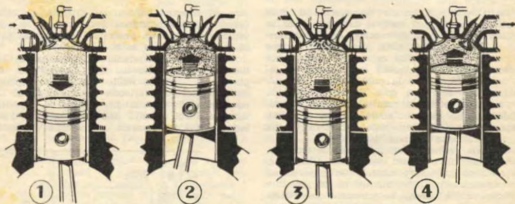
Fig. 3. — In queste quattro figurine, sono rappresentate le fasi di un motore a quattro tempi. Aspirazione, Compressione, Scoppio-Espansione e Scarico.
