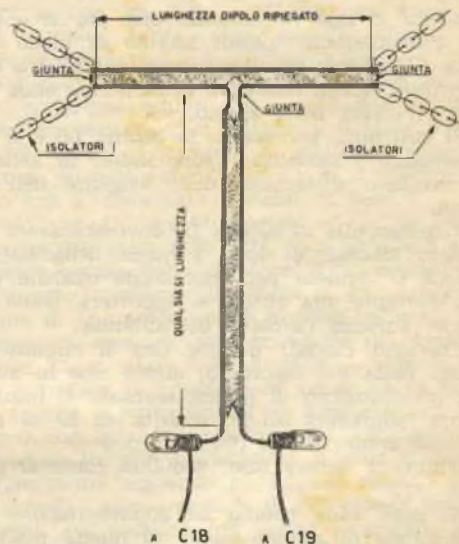
Fig. 13. — Soltanto la piattina bifilare da 300 ohm, si presta alla costruzione dell'antenna a dipolo ripiegato che qui vedete.
