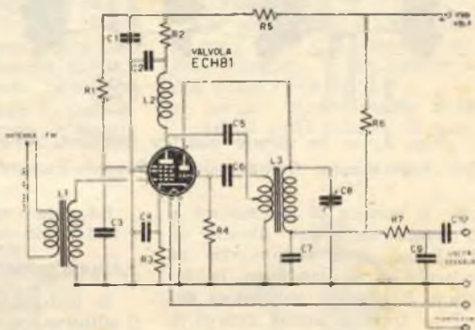
Fig. 1. — COMPONENTI.
