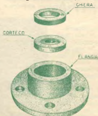
Fig. 3. — Per fissare il corteco alla vasca, ci si servirà di una flangia e di una ghiera entro i quali si serrerà il corteco stesso.
