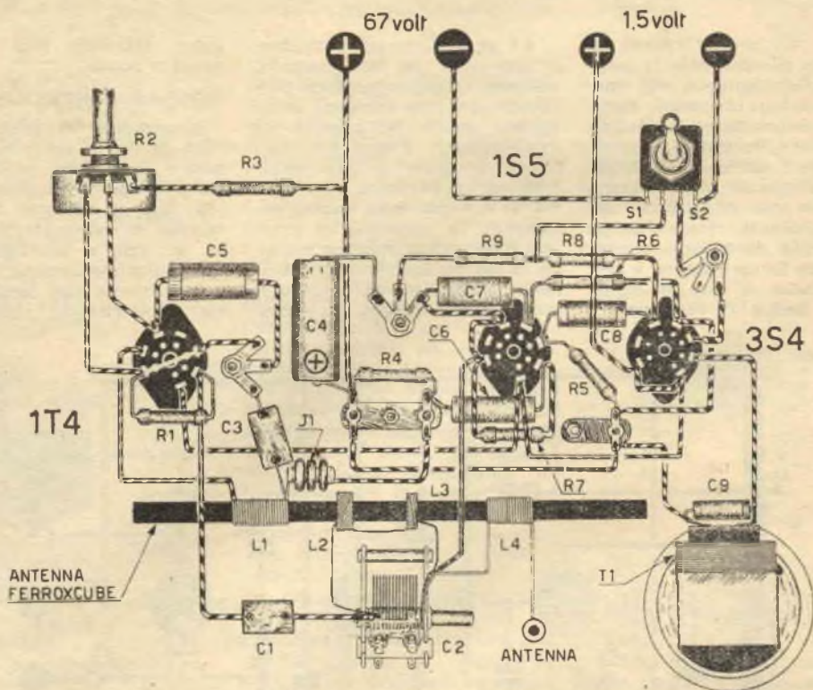
Fig. 2. — Schema pratico.
