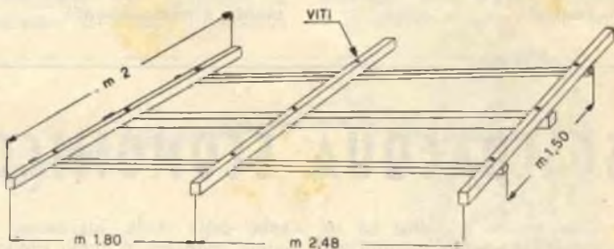
Fig. 8. — La culla di sostegno per gli elementi d'antenna, che normalmente si costruisce con tubo ANTICORODAL, può essere costruita anche in legno. Ecco le dimensioni relative alla culla di un'antenna per la gamma dei 20 metri.
