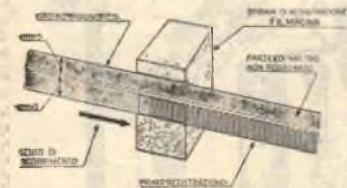
Fig. 3 — In un Registratore a doppia traccia il nastro viene registrato solamente su una sola metà della larghezza totale.
