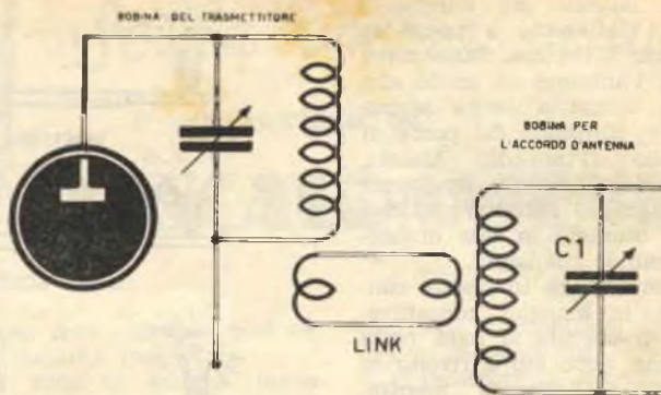
Fig. 7. — L'accordo in parallelo delle due bobine è necessario quando con l'accordo in serie l'antenna non assorbe la energia AF irradiata dal trasmettitore. In questo caso la capacità del condensatore variabile C1 sarà di 50 pF al massimo; riguardo alle spire della bobina per l'accordo d'antenna, vedere fig. 6.
