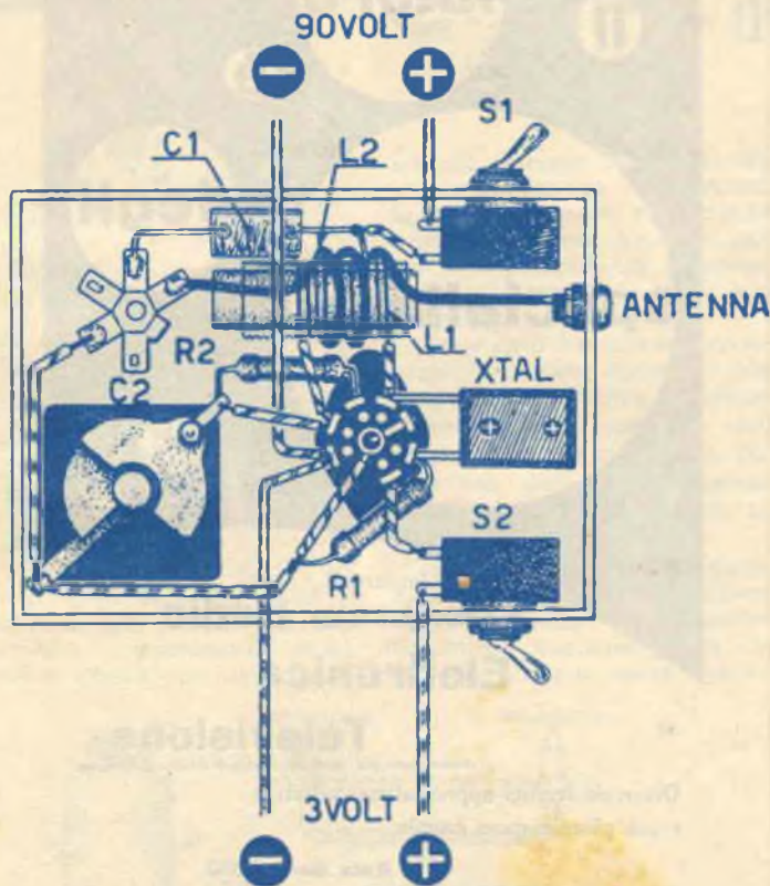
Fig. 2. — Schema pratico del radiocomando descritto nell'articolo.
