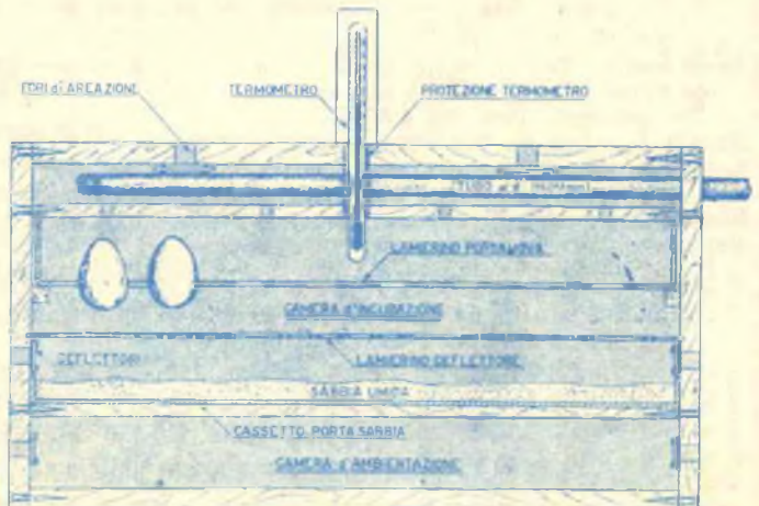
Fig. 1. — Ecco come si presenta lo spaccato dell'incubatrice.
