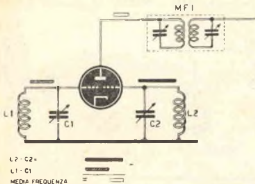
Fig. 3. - Qui sopra è sintetizzato un circuito cambia-frequenza, in cui C1 e L1 rappresentano il circuito di sintonia, C2 e L2 quello oscillatore, e MF1 la Media Frequenza.
