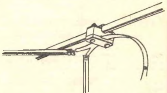
Fig. 6. — Utilizzando per la discesa piattaforma bifilare da 300 ohm, i due capi verranno collegati ai due esterni dell'elemento a Delta. La piattaforma dovrà essere tenuta fissata al tubo di supporto a mezzo di un apposito isolatore distanziatore visibile in fig. 8.
