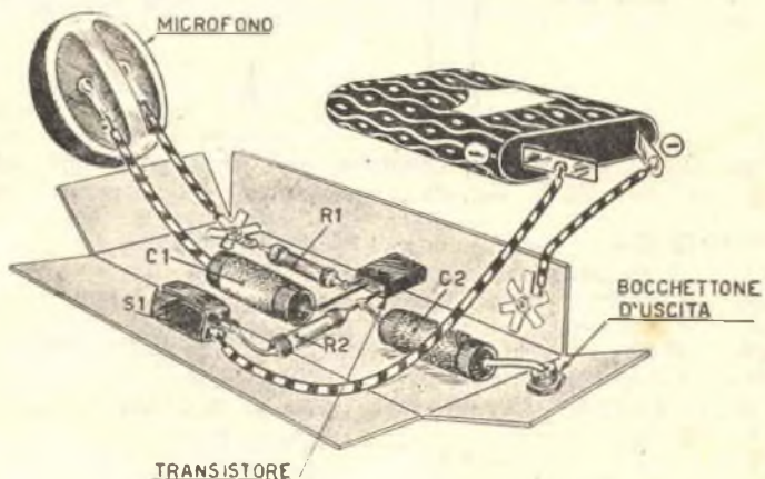
Fig. 7. - Schema pratico del preamplificatore a transistori.
