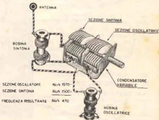
Fig. 2. - La differenza di frequenza dei due circuiti, è sempre uguale al valore della Media Frequenza, qualunque posizione assumano le lamelle del variabile.
