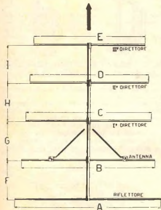
Fig. 1. — Il piano costruttivo dell'antenna. Le dimensioni A - B - C - D - E - F - G - H - I si potranno ricavare dalle tabelle N. 1, N. 2 e N. 3.
