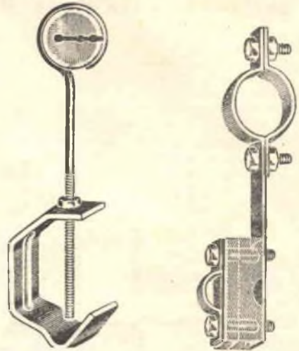
Fig. 5. — Ecco due tipi di isolatori-distanziatori da utilizzare per la piattaforma di discesa.
