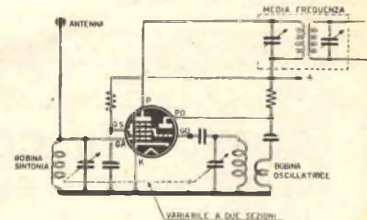
Fig. 4. - In pratica per la conversione di frequenza non si fa uso di una valvola come quella della fig. precedente, bensì di una valvola versione di frequenza mediante un triodo-esodo, molto più complessa. Qui è rappresentata la con-
