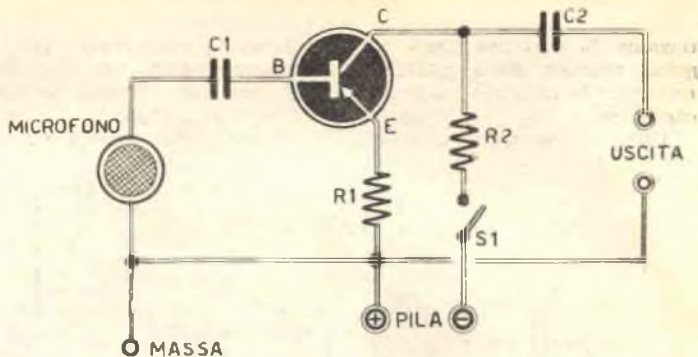
Fig. 6. - Lo schema elettrico del preamplificatore a transistori.
