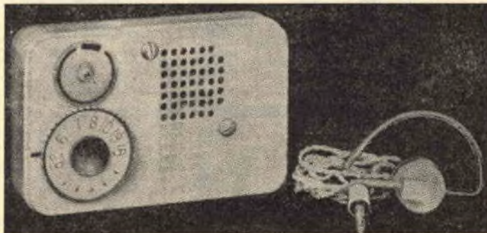
Fig. 3. — Come si presenta il Reflex ad 1 transistor realizzato in sede di elaborazione
