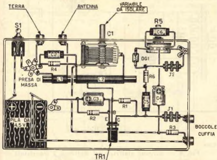
Fig. 2. — Schema pratico del Reflex a 1 transistor
