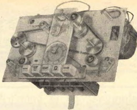
Fig. 2. — Piastra di montaggio completo.
