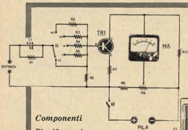
Fig. 3 - Schema elettrico del voltmetro a transistor.
