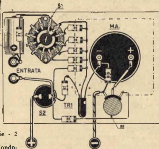
Fig. 4 - Schema pratico del voltmetro a transistor.
