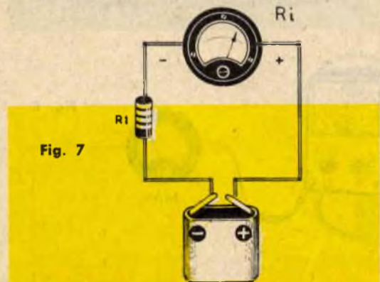
Fig. 7 - Non possedendo un milliamperometro si può ugualmente determinare la sensibilità di uno strumentino realizzando il circuito di figura: tutto sta nell'individuare una resistenza di valore noto che faccia deviare l'indice a fondo-scala e nell'applicare la formula riportata nell'articolo.
