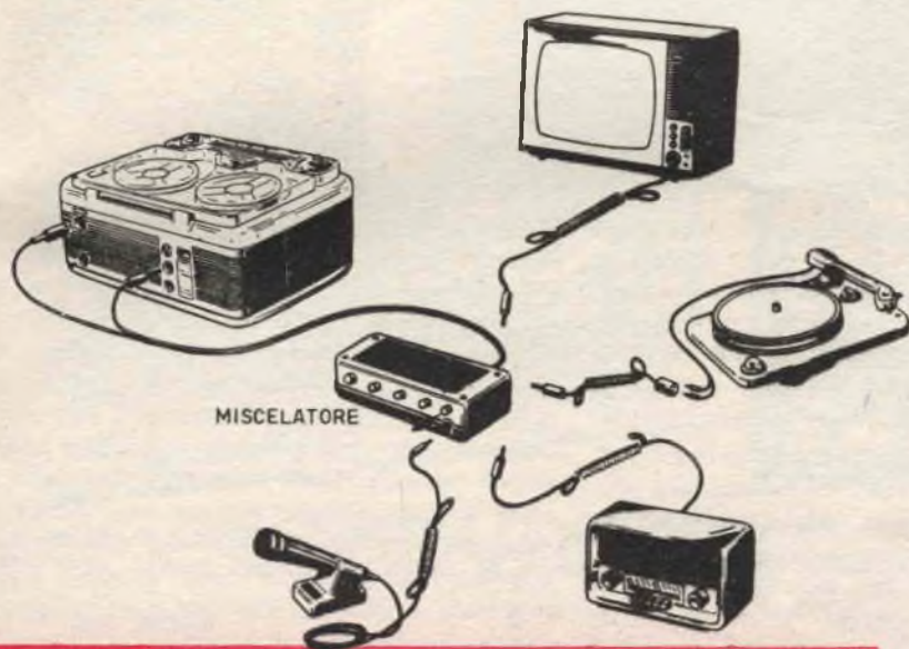
Fig. 7. Per la sovrapposizione dei suoni è indispensabile utilizzare un miscelatore di segnale. Con questo elemento è possibile sovrapporre nella proporzione desiderata, i suoni provenienti da più fonti.
