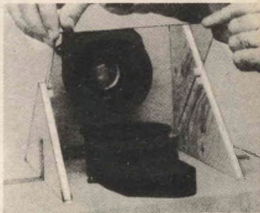
Fig. 3 Per dirigere l'immagine verso il muro dovrete applicare sopra l'obiettivo uno specchio di alta qualità, inclinato di 45^\circ .
