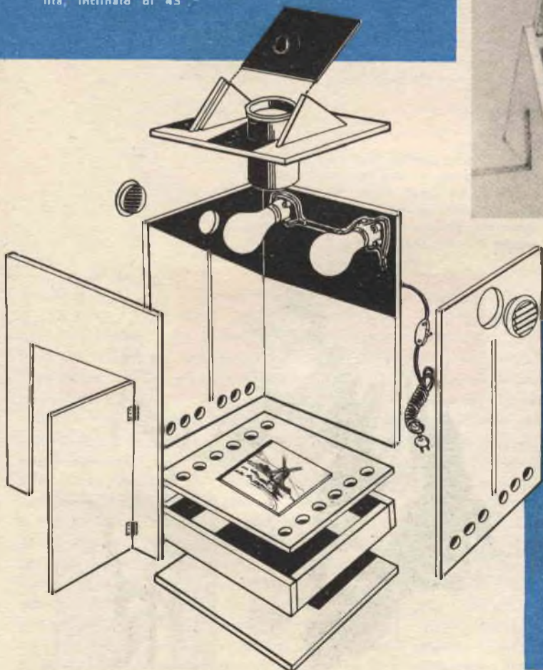
Fig. 3 Per dirigere l'immagine verso il muro dovrete applicare sopra l'obiettivo uno specchio di alta qualità, inclinato di 45^\circ .
