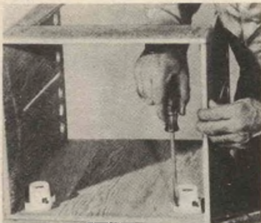
Fig. 1. Le dimensioni della cassetta, per questo proiettore, sono facoltative; in linea di massima, si potranno considerare cm. 30 x 25 di base e cm. 35 di altezza. Al margine superiore si fisseranno i due portalampade, disponendoli in modo da poter avvitarle agevolmente le lampadine. Per aumentare la luminosità, si potranno fissare superiormente degli specchi in modo che la luce sia riflessa sul piano su cui appoggia l'immagine da proiettare.
