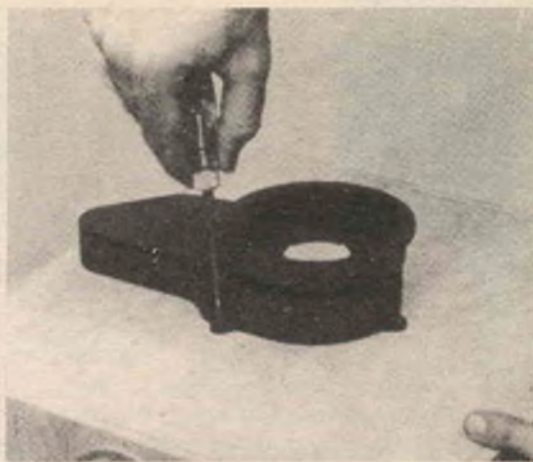
Fig. 2. Il componente più importante del proiettore è l'obiettivo. Cercate presso qualche negozio di ottica delle vecchie macchine a soffietto e tagliate loro l'obiettivo; scegliete quello le cui lenti abbiano il massimo diametro, poiché maggiore è il diametro, maggiore luminosità avrà l'immagine. L'obiettivo verrà fissato al centro del piano superiore con qualche vite e, se necessario, con un collare.
