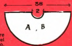
Fig. 5. Elementi costituenti la vasca semicilindrica in plexiglass: a,b) semicerchi; c) foglio di fissare ai semicerchi mediante l'apposito mastice.
