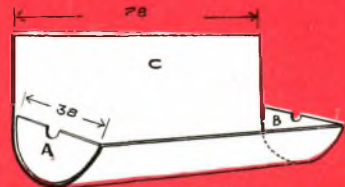
Fig. 5. Elementi costituenti la vasca semicilindrica in plexiglass: a,b) semicerchi; c) foglio di fissare ai semicerchi mediante l'apposito mastice.
