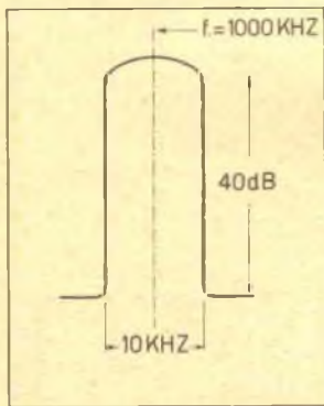
Curva approssimativa della selettività a 1MHz
