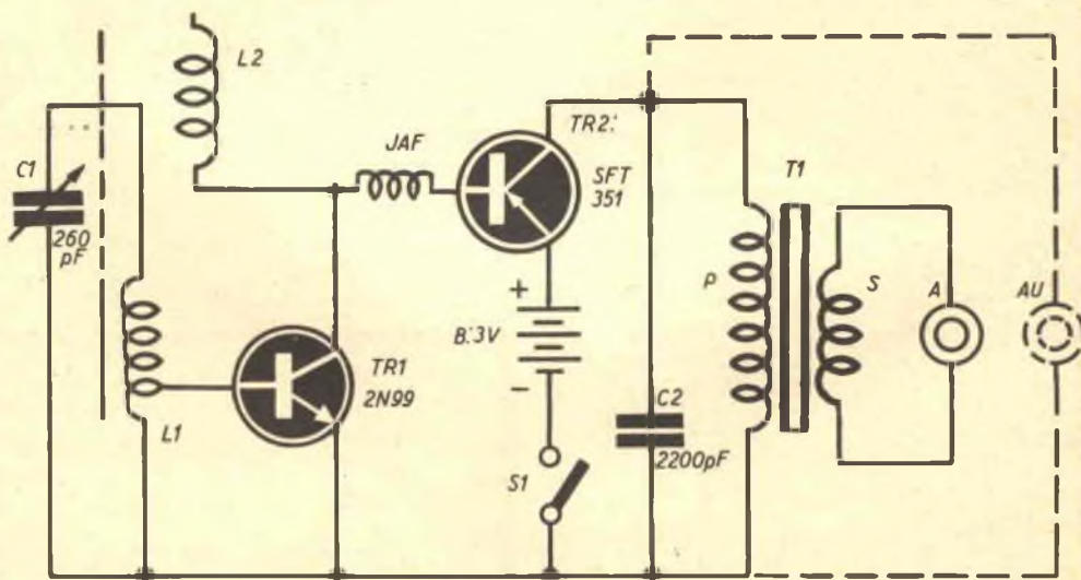
FIG. 1: SCHEMA ELETTRICO
