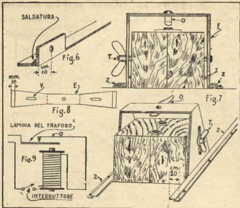
ARCHETTO ELETRICO DA TRAFORO - Segue da pag. 195
