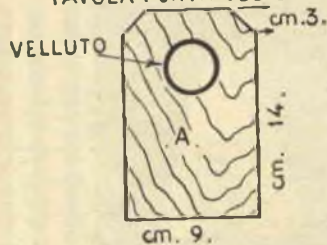
TAVOLA PORTA OBBIETTIVO
