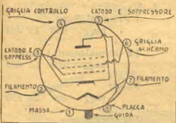
Zoccolo della valvola 717A - Serie Octal
