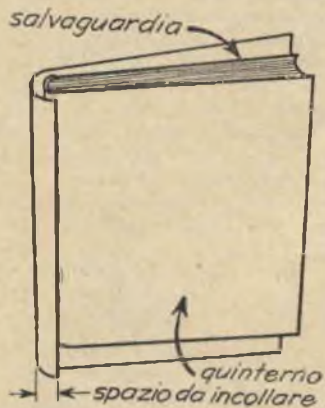
FIG. 15 - Modo di posare le salvanguardie
