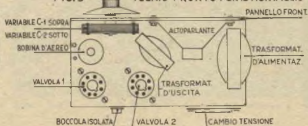
FIG.5 TELAIO PRONTO PER IL MONTAGGIO
