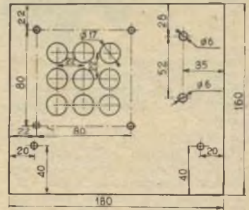
FIG.7 PANNELLO FRONTALE
