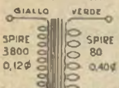
FIG.2 SCHEMA DEL TRASFORM.D'USCITA
