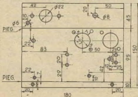
FIG. 6 TELAIO DI ALLUMINIO
