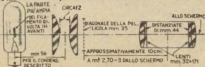
LAMPADA A CONTATTO UNICO PER PROIEZIONE 100 WATT
