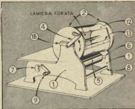
FIG. 12 TELA INCHIOSTRATRICE
