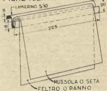
FIG. 12 TELA INCHIOSTRATRICE
