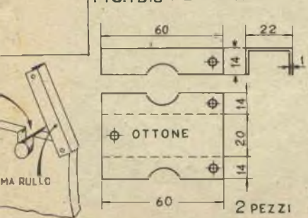
FIG. 1 Bis FERMARULLO
