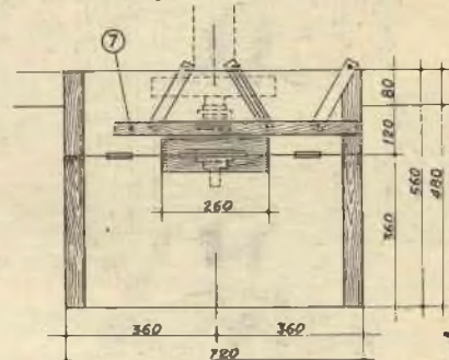
FIG. 5c PIANTA
