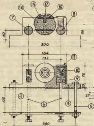
FIG. 1c FIANCO SEZIONATO
