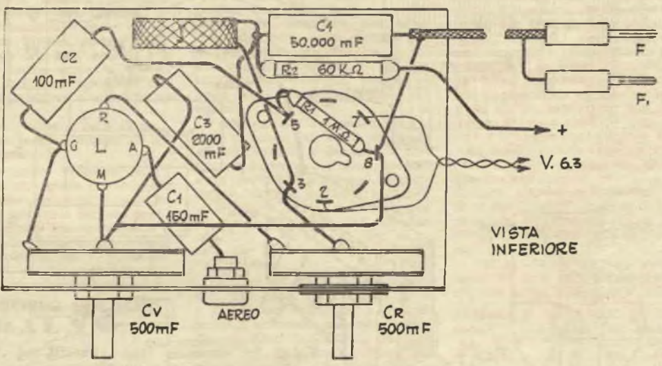
Fig. 4 SCHEMA COSTRUTTIVO
