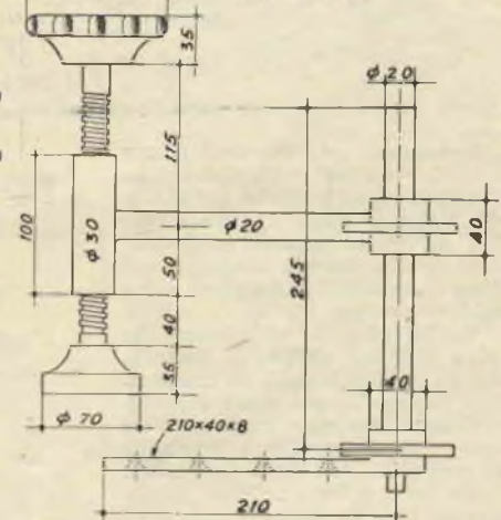
FIG. 4 p VITE DI BLOCCAGGIO PARTIC. 12
