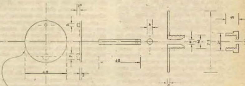
PIATTINA D'INNESTO PER LA CHIAVETTA DELLA CINEPRESSA PAILLARD "L8"
