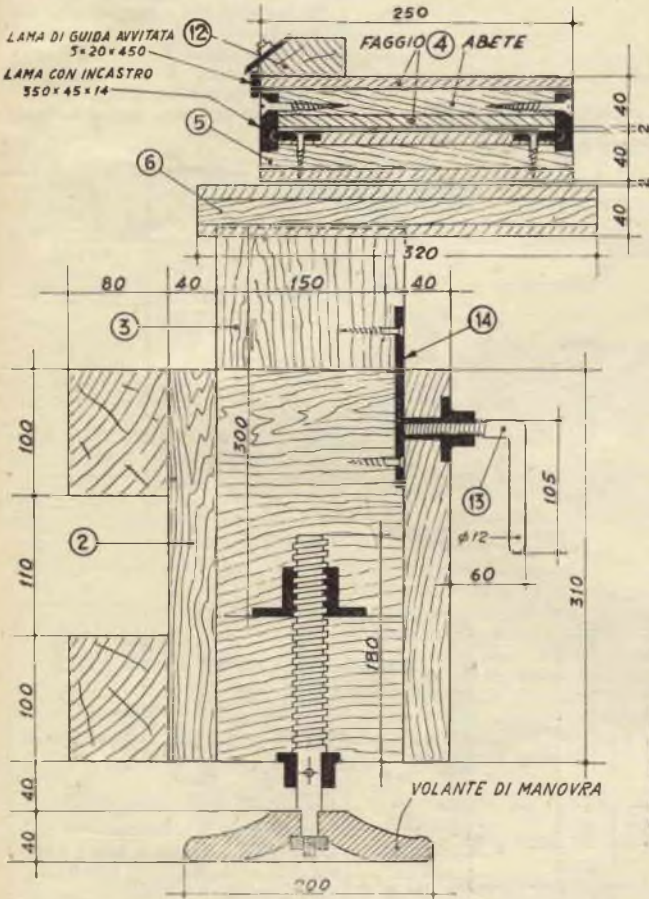
FIG. 4e CONGEGNO SOLLEVAMENTO PARTIC.
