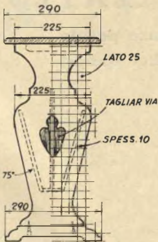
VEDUTA LATERALE
