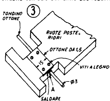
FISSARE RUOTE E PULEGGIA SUL TONDINO UNGERE CON OLIO L'INTERNO DEL TUBETTO "A."
