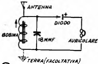
④ SCHEMA ELETRICO
