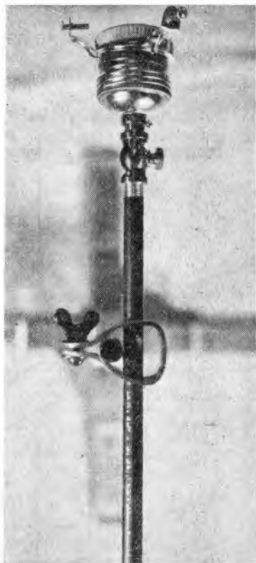
Il braccio porta lampada (in realtà esso deve stare in posizione orizzontale; qui è raffigurato verticalmente per comodità di impaginazione) completo di fermo scorrevole, raccordo a snodo e portalampada.
