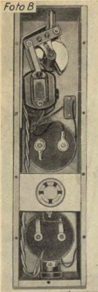
Foto B - Veduta posteriore dello strumento montato. Notate il pannello di alluminio che sorregge lo zoccolo a 5 terminali. Il coperchio è fatto di plastica trasparente
