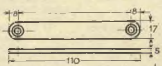
2 FLANGIE (Legno) A = 2 PEZZI B = 1 PEZZO LISCIO B' = 1 PEZZO CON GOLA
