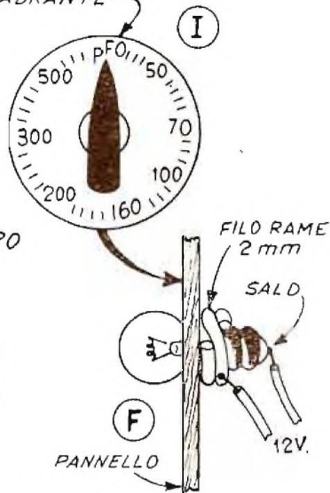
ESEMPIO DI QUADRANTE
