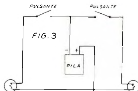
SCHEMA ELETTRICO
