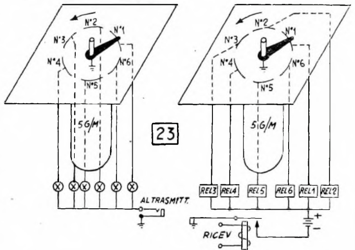
Fig. 23. - Due commutatori sincronizzati, uno alla stazione trasmittente ed uno alla ricevente permettono un buon sistema di comando a distanza.
