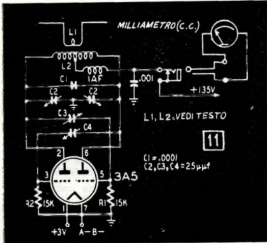
Fig. 11. - Semplicissimo trasmettitore, da usare con i ricevitori monovalvolari precedentemente descritti.
