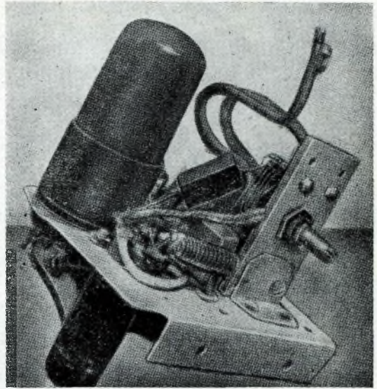
Fig. 13. - Il trasmettitore completamente montato permette di vedere le bobine in tubo di rame da 6 mm.
