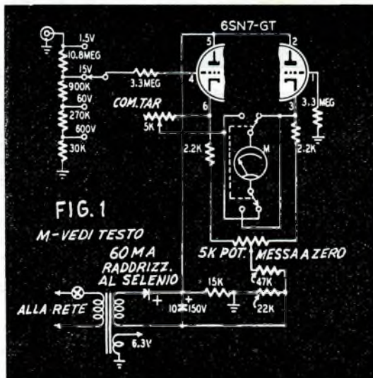
Questo circuito semplicissimo permette la realizzazione di uno strumento più che sufficiente ad un dilettante per quanto non adatto ad un professionista
