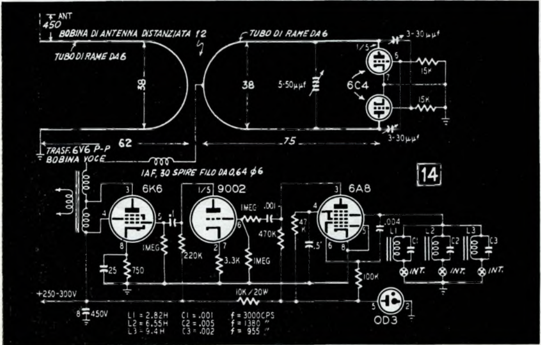
Fig. 14. - Trasmittitore con due 6C4 in push-pull, di potenza assai superiore ai tipi precedenti, richiede una sorgente di energia capace di assicurare circa 300 volt.
