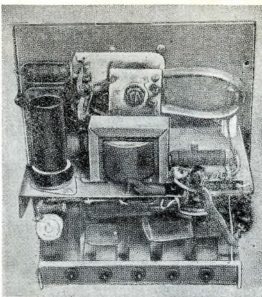
Fig. 15. - Il trasmettitore di figura 14 completamente montato. Se ben allineato questo apparecchio è capace di dare risultati eccellenti.
