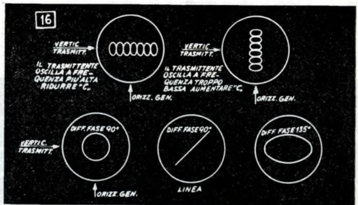
Fig. 16. - Controllo delle frequenze di trasmissione dell'apparecchio di figura 14.
