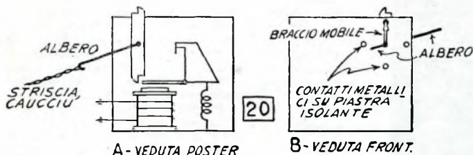
Fig. 20 (a e b) - Un semplicissimo stepper è costituito da un relay e da un braccio ruotante (a). Sul retro (b) la spazzolina ed i contatti.
