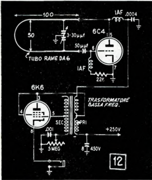
Fig. 12. - A fianco lo schema elettrico di un trasmettitore includente uno stadio modulatore.
