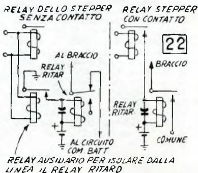
Fig. 22 - Un relay a ritardo fa sì che durante il suo movimento il braccio mobile non innesterà alcun circuito.
