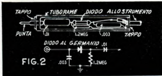
Schema costruttivo ed elettrico della punta esploratrice
