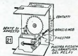
Fig. 21 - Una ruota dentata ed un dente di arresto permettono alla spazzola di agire su di un maggior numero di contatti.
