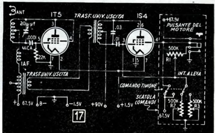
Fig. 17. - Trasmettitore particolarmente adatto per un decodificatore ad aste vibranti.
