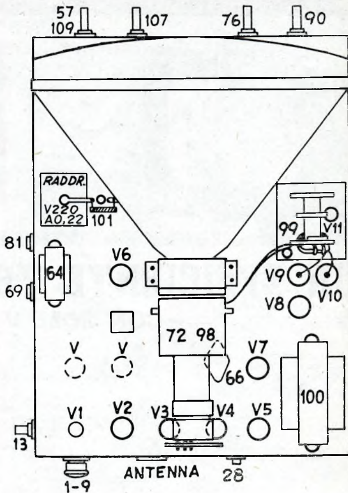
DISPOSIZIONI PARTI SULLO CHASSIS DEL T/11
