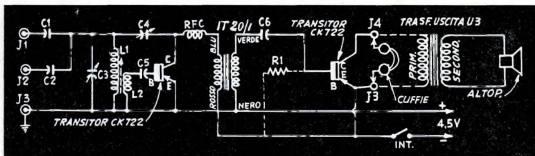
Schema elettrico del ricevitore a reazione a due transistor. Il circuito di principio è quello dell'emettitore a massa.
