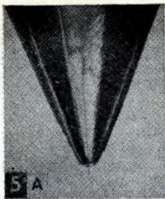
(A) Come appare al microscopio una puntina per microscolco nuova. (B) come appare, sempre al microscopio, una puntina per dischi a 78 giri, nuova. (C) Dopo una cinquantina di ore di uso, la punta di uno stiletto di zaffiro comincerà a perdere la sua rotondità e ad assumere, invece un profilo simile a quello di uno scalpello. (D) Dopo 100 ore di uso, la punta sarà stata sostituita da un filo piatto, molto tagliente, che oltre a produrre degli indesiderabili rumori ed a diminuire la resa, specie delle frequenze alte, danneggerà irrimediabilmente i dischi.
