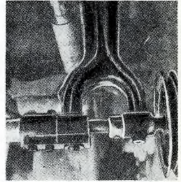
Veduta ravvicinata del supporto di banco modificato: è possibile notare che l'adattatore è unito al supporto stesso per mezzo delle sue staffe (superiore ed inferiore).
