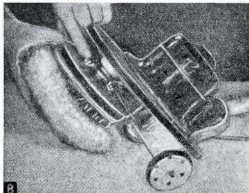
L'insieme formato dal disco di gomma e dal tampone di lana di agnello viene trattenuto contro la superficie inferiore della spazzola grazie a due lunghe viti strette, al di sopra della spazzola, da due galletti.
