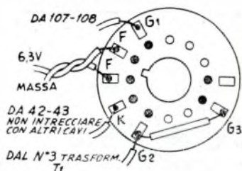
Collegamento allo zoccolo del cinescopio.
