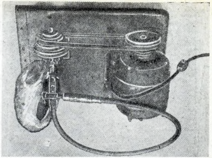
Veduta del complesso motore accessorio ed albero flessibile, montati su di un supporto di legno. Il motore può inclinarsi all'indietro, per mantenere la cinghia di trasmissione nella giusta tensione. Il cambiamento della velocità di rotazione dell'albero flessibile si ottiene passando la cinghia da una coppia di pulegge ad un'altra.
