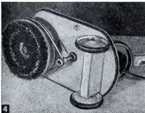
Il sistema delle due pulegge e della cinghia di trasmissione assicura la diminuzione di velocità di rotazione della spazzola; la potenza viene, viceversa, aumentata.
