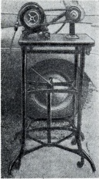
Veduta di fianco del complesso pronto per funzionare: notare l'inclinazione del motore elettrico. Nella foto, il basamento, pure munito delle proprie rotelle è stato poggiato su di una intelaiatura metallica formata da profilato angolare in ferro, in modo che risulti di più agevole manovra.
