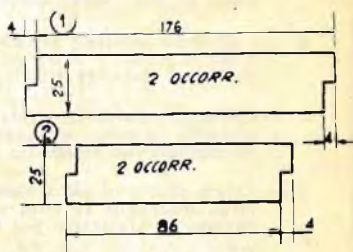
Modelle delle pareti laterali della scatola.
