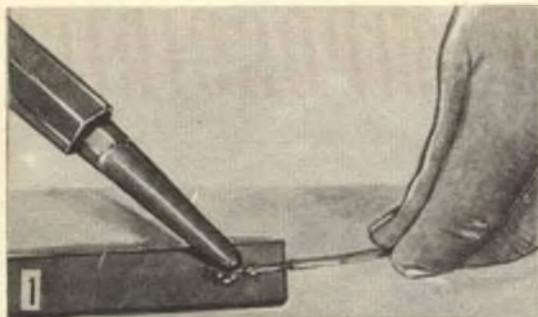
Foto 1 - Semplice saldatura di un filo di rame ad un pezzo di grafite, secondo la nuovissima tecnica, di recente scoperta ed illustrata nel presente articolo. Foto 2 - Prima operazione è quella del riempire di lega per saldare, le porosità della rotella abrasiva, fissata su di un utensile a motore; è bene che la lega sia ad alto tenore di stagno; ossia al 60% Sn ed il 40% Pb.
