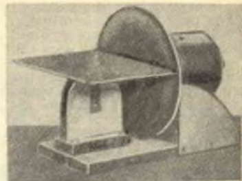
L'utensile multiplo, preparato per funzionare come lisciatrice a piano inclinabile, il disco su cui viene incollata la carta o la tela abrasiva può essere di 15 o di 20 cm.
