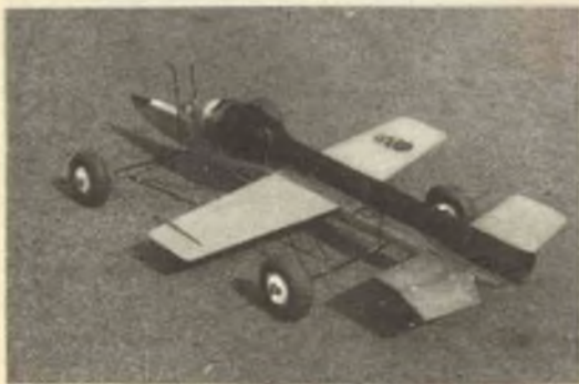
Un altro convenzionale modello da velocità con pulsogetto.
