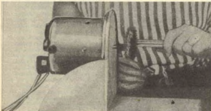
Con questa semplice disposizione il complesso può essere usato come lucidatrice e pulimentatrice ad alta velocità: le spazzole vi possono essere fissate a mezzo di un mandrino conico. Con la stessa disposizione il complesso può essere usato come piccola mola a motore.
