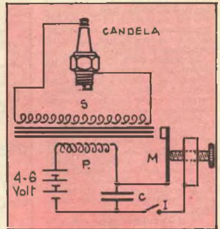
Schema elettrico impianto accensione.
