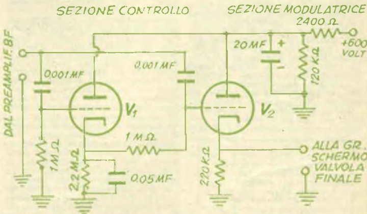
V1 e V2 - LE SEZIONI DI UNA VALVOLA 12 AU 7
