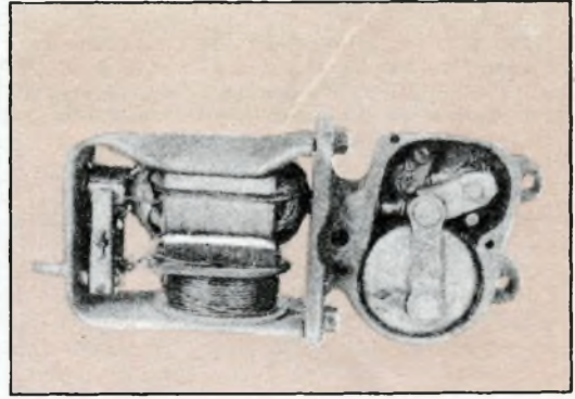
(Foto a sinistra): Altro esempio tipico, da tenere presente se una volta che il motorino sia separato dalla carcassa contenente gli altri meccanismi, alcune delle sue parti, quali il rotore e le spazzole rimangono prive di appoggio. In questo caso, i perni per il rotore sono costituiti da due laminette di ottone o di acciaio, opportunamente montate. - (Foto a destra): Veduta interna di uno dei motori elettrici, con collegato, il meccanismo di trasformazione del movimento: tutta la parte di destra può essere tagliata senz'altro, liberando il motorino di sovrastrutture inutili e mettendo anche allo scoperto il suo asse rotante. Il taglio della struttura di destra, nel suo punto più sottile può anche essere eseguita con un archetto da traforo, munito di lama a metallo
