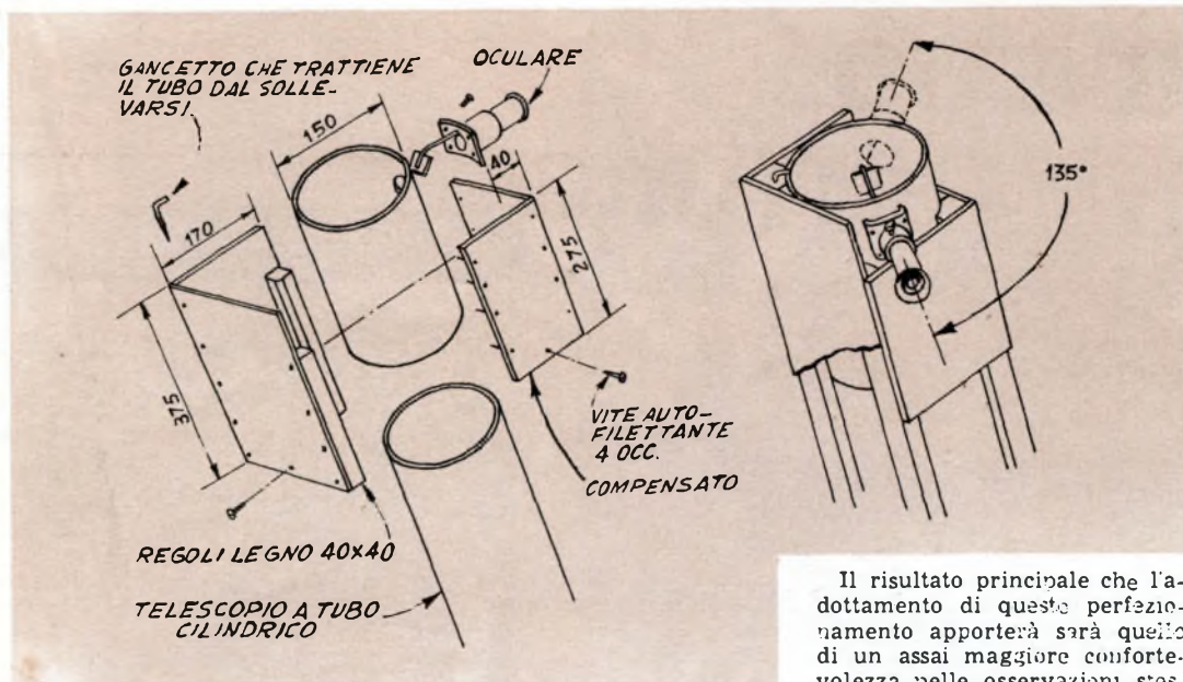
Nella tavola di sinistra, è illustrata la modifica nel caso di un telescopio munito di una struttura cilindrica, mentre nella illustrazione di destra è indicata la modifica da attuare nel caso di un telescopio a struttura parallelepipedica, in ognuno dei casi, la rotazione massima possibile per l'oculare è di circa 135 gradi
