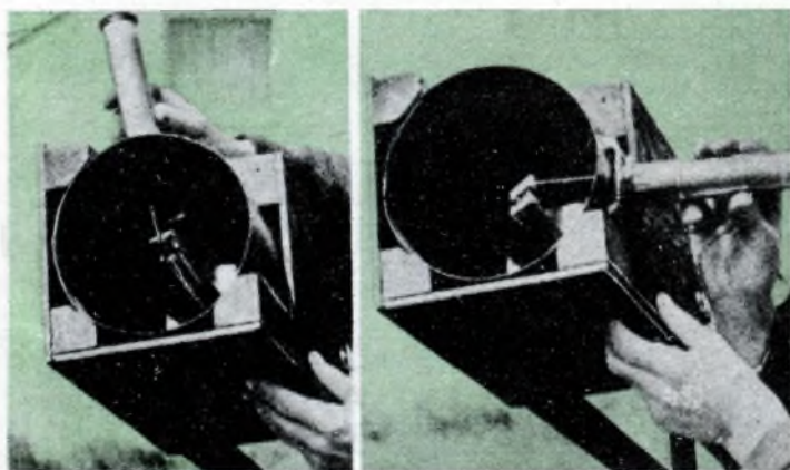
Un esempio pratico dell'impiego dell'oculare orientabile: una volta effettuato il puntamento del telescopio, si ruota l'oculare nella posizione che risulti la più conveniente alla osservazione e la più comoda
