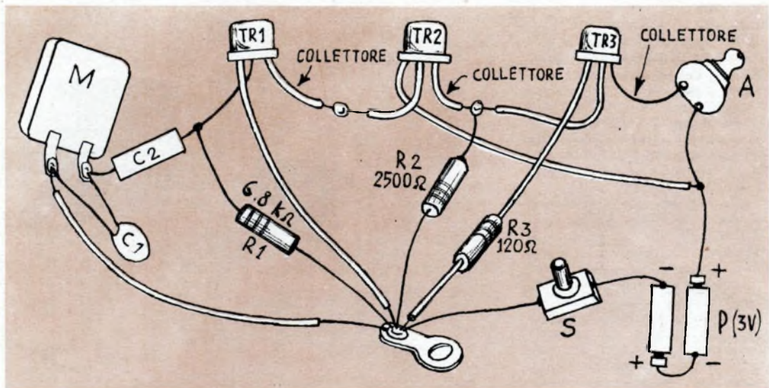
SCHEMA PRATICO. Nota: sostituendo R2 un potenziometro di pari valore si atterrà il controllo di volume. Per il valore di C1 vedi testo
