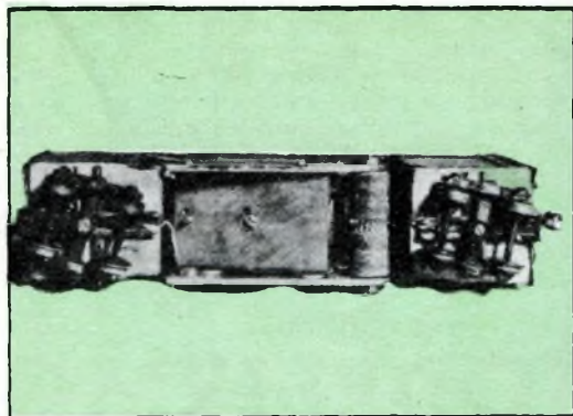
(Foto a sinistra): Veduta, dal di sotto, del complesso per la pulitura automatica delle rotaie: posso assicurare che con un tale dispositivo, è possibile portare a termine in un quarto di ora, un lavoro che se condotto manualmente, richiederebbe non meno di un'ora, a parte le difficoltà secondarie che esso presenterebbe. - (Foto a destra): Il motore con la vite senza fine, pronto per essere installato sullo chassis, su cui si trova già il cilindro rotante abrasivo, con la ruota dentata nel suo centro. Se si tratti di un impianto ad alimentazione sulle due rotaie, occorre usare, come del resto per tutte le vetture dei convogli che si fanno marciare su di esso, un carrello avente le ruote isolate dalla massa del carro stesso, perché non abbia a verificarsi qualche cortocircuito.
