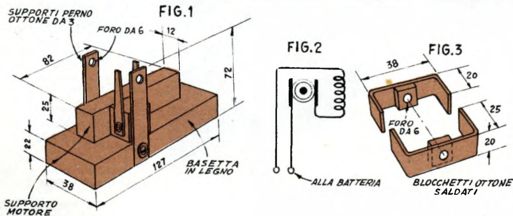
Esempio tipico di montatura, in legno e metallo, particolarmente adatta nel caso di motorini che non abbiano una carcassa unica che sostenga il sistema delle spazzole ed il perno dell'asse del rotore. In fig. 2, i due principali collegamenti tra rotore e statore, le cui caratteristiche sono discusse nel testo
