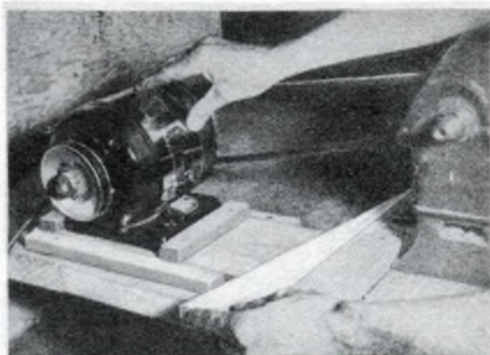
La base del motore viene a poggiare tra i due listellini trasversali, sulla bassetta scorrevole. Nota la forma del listellino posteriore, destinata ad impedire che sotto lo sforzo di rotazione, il motore possa impennarsi sul suo basamento, dato che questo non risulta perfettamente ancorato alla base
