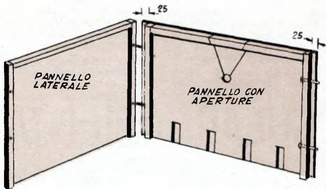
Costruzione dei pannelli laterali, isolanti
