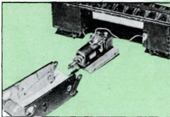
(Foto a sinistra): Veduta, dal di sotto, del complesso per la pulitura automatica delle rotaie: posso assicurare che con un tale dispositivo, è possibile portare a termine in un quarto di ora, un lavoro che se condotto manualmente, richiederebbe non meno di un'ora, a parte le difficoltà secondarie che esso presenterebbe. - (Foto a destra): Il motore con la vite senza fine, pronto per essere installato sullo chassis, su cui si trova già il cilindro rotante abrasivo, con la ruota dentata nel suo centro. Se si tratti di un impianto ad alimentazione sulle due rotaie, occorre usare, come del resto per tutte le vetture dei convogli che si fanno marciare su di esso, un carrello avente le ruote isolate dalla massa del carro stesso, perché non abbia a verificarsi qualche cortocircuito.
