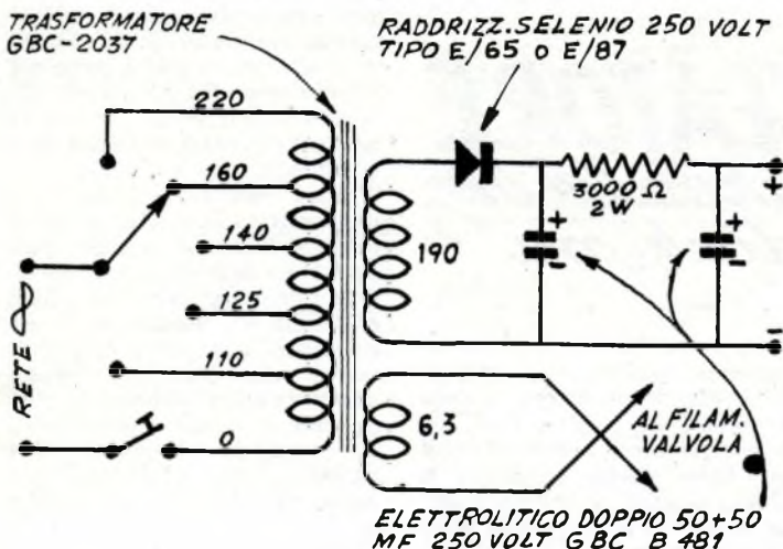
Schema alimentare autonomo
