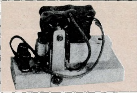
(Foto a sinistra): Altro esempio tipico, da tenere presente se una volta che il motorino sia separato dalla carcassa contenente gli altri meccanismi, alcune delle sue parti, quali il rotore e le spazzole rimangono prive di appoggio. In questo caso, i perni per il rotore sono costituiti da due laminette di ottone o di acciaio, opportunamente montate. - (Foto a destra): Veduta interna di uno dei motori elettrici, con collegato, il meccanismo di trasformazione del movimento: tutta la parte di destra può essere tagliata senz'altro, liberando il motorino di sovrastrutture inutili e mettendo anche allo scoperto il suo asse rotante. Il taglio della struttura di destra, nel suo punto più sottile può anche essere eseguita con un archetto da traforo, munito di lama a metallo
