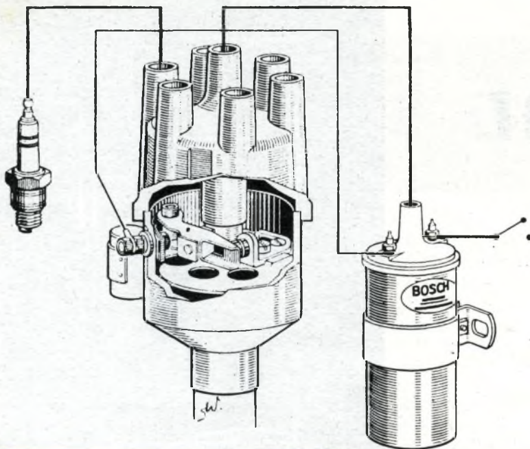
Figura 2a Impianto d'accensione a batteria per motori « a più cilindri », in esecuzione standard.
