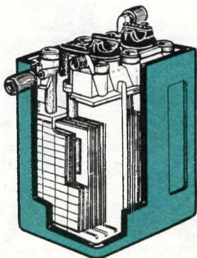
Fig. 2 - Sezione di una batteria classica al piombo, dalla quale appare la disposizione delle placche e dei setti.
