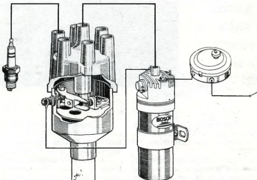
Figura 2b Impianto d'accensione BOSCH a transistor con comando a rottore. In questo sistema d'accensione il rottore meccanico opera con la sola corrente di comando del transistor. Quest'ultimo è alloggiato sull'estremità superiore della bobina, all'interno di una apposita calotta alettata, e comanda la corrente di lavoro in passaggio attraverso la bobina. Nel corpo circolare a destra è sistemata una prerresistenza.
