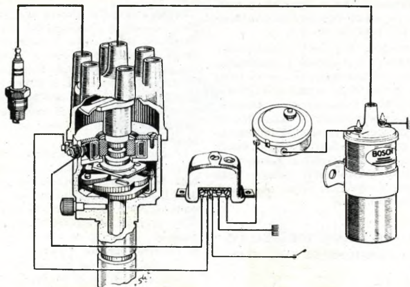
Figura 3 Impianto d'accensione BOSCH a transistor con comando magnetico. Nello spinterogeno, in luogo del rottore, è previsto un generatore di impulsi del tipo a magnete permanente, che assolve le funzioni del rottore meccanico. Questo generatore comanda il transistor dello stadio finale (sulla destra dello spinterogeno) per mezzo di impulsi elettrici, tramite un comando elettronico; il transistor, a sua volta, comanda la corrente di lavoro che passa attraverso la bobina, come per l'impianto con comando a rottore. Nel corpo circolare è sistemata una prerisistenza.
