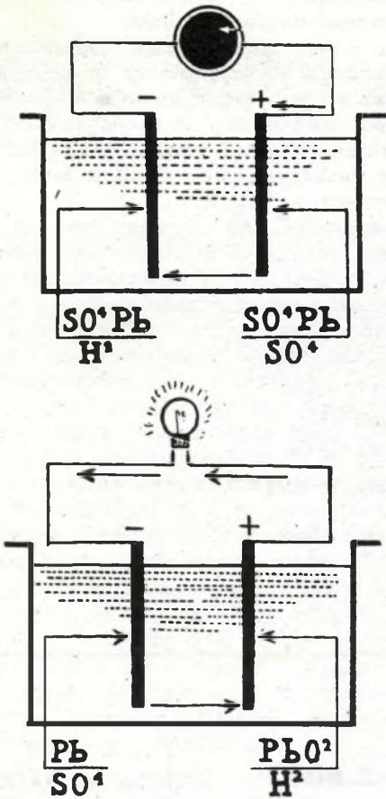
Fig. 1 - Le due fasi delle reazioni chimiche che avvengono in una batteria. In alto, al momento della carica, la corrente va, nella batteria dal + al -. In basso, quando avviene la scarica, il senso della corrente è invertito e la reazione chimica anche.
