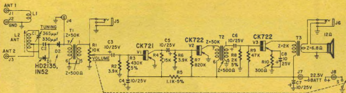
FIG. 1 - SCHEMA ELETTRICO
