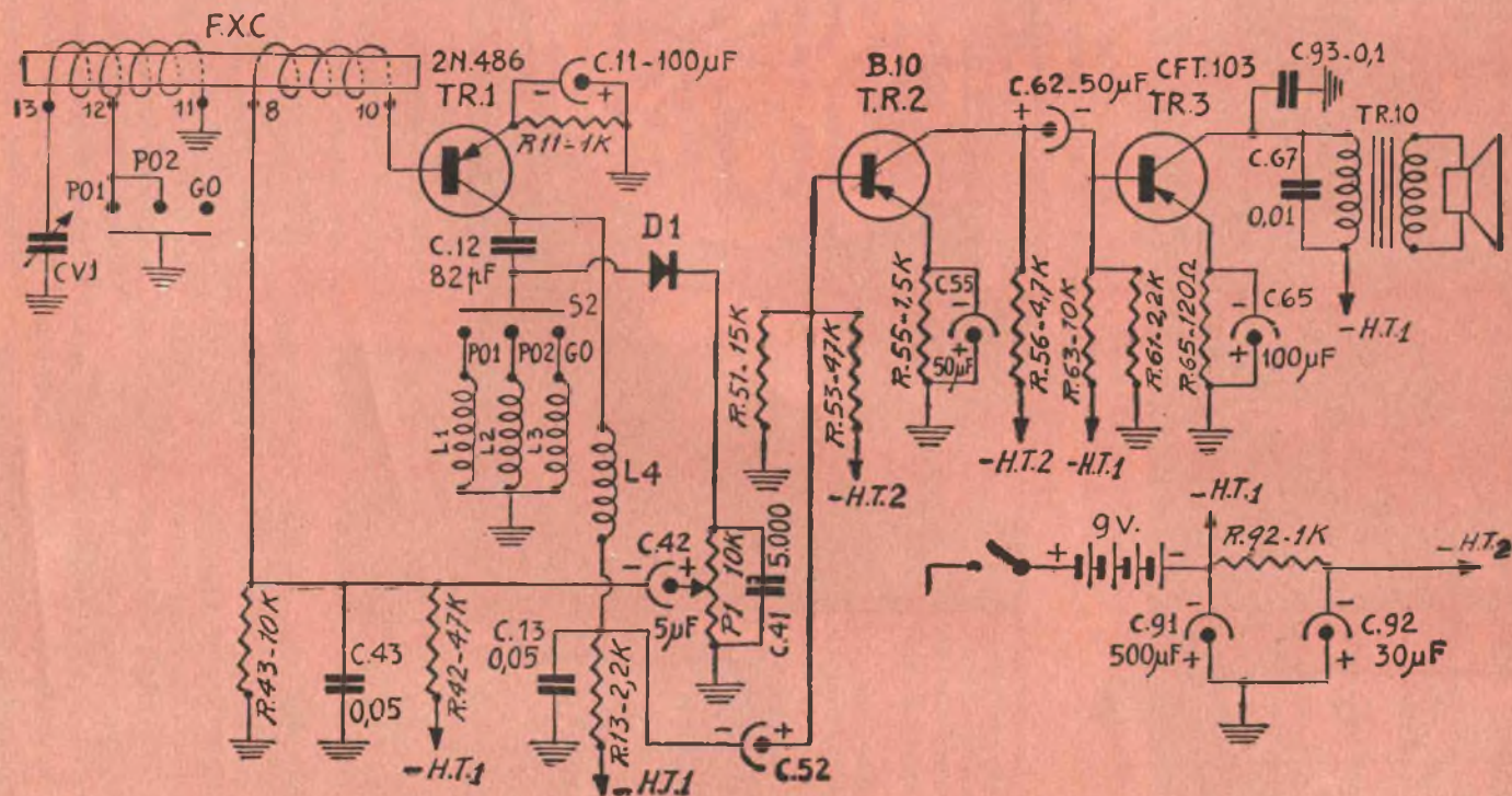
FIG. 2 - Schema elettrico del ricevitore descritto nell'articolo.
