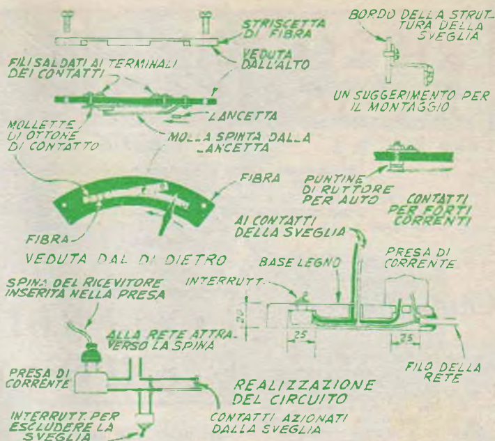
Dettagli costruttivi delle varie parti, è suggerita anche una versione con contatti in grado di dissipare una potenza maggiore
