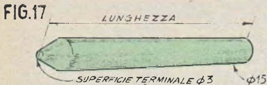
Fig. 17 - Tipo consigliato per punta saldante dritta. Quella inferiore, S deve essere lunga, mm. 100, quella superiore, invece deve essere lunga mm. 150
