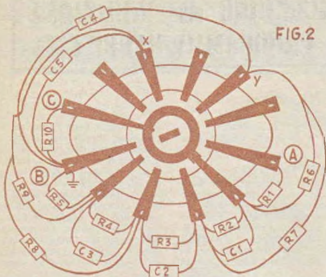
IL COMMUTATORE È VISTO DI SOTTO I TERMINALI X Y SERVONO DI APPOGGIO E SONO DELLA SEZIONE INUTILIZZATA
