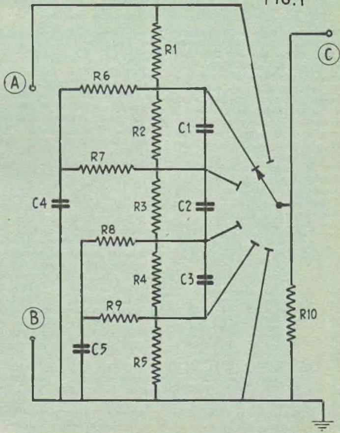
SCHEMA ELETTRICO
