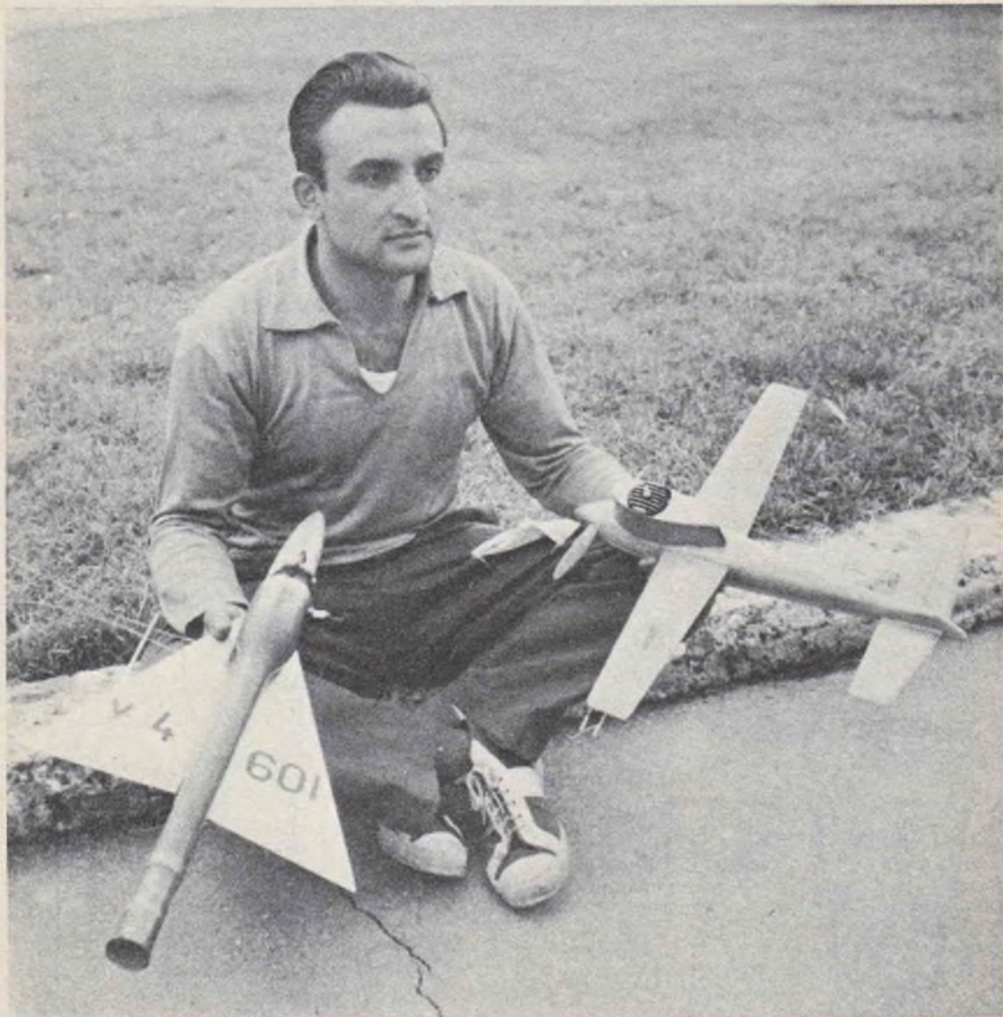
UN MODELLO DA VELOCITA' CON ALA A DELTA E MOTORE A REAZIONE PARAGONATO CON UN MODELLO CON MOTORE A SCOPIO DI TIPO CONVENZIONALE
