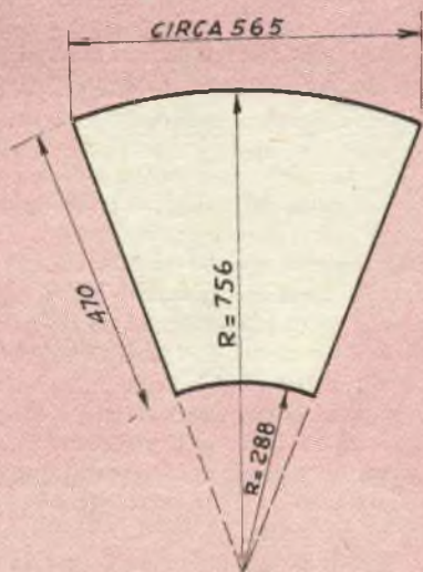
DETTAGLIO TRAPEZOIDALE FORMANTE LA SEZIONE INFERIORE TRONCOCONICA FARNE 4 UGUALI
