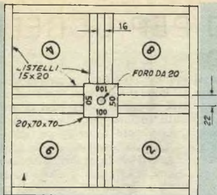
BASE IN COMPENSATO DA 400x400
