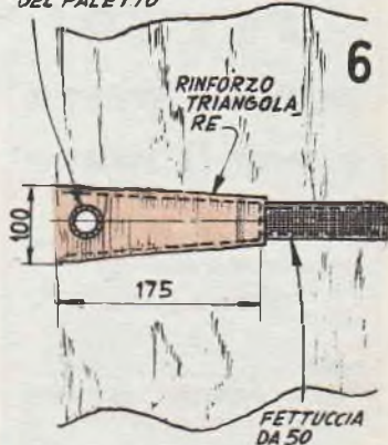
Sistema di rinforzo lungo la linea centrale del tettino e del sopra-tetto, per il foro destinato a fare passare il paletto verticale
