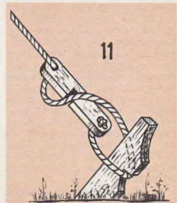
Dettagli del picchetto, del tirantino e del tenditore
