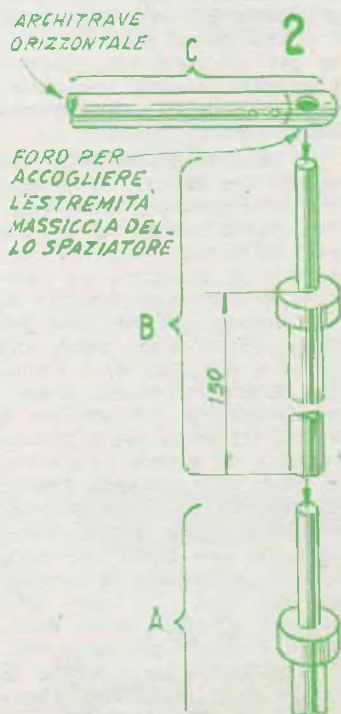
Dettaglio del paletto e dell'architrave orizzontale: A è il paletto; B, lo spaziatore e C è appunto l'architrave
