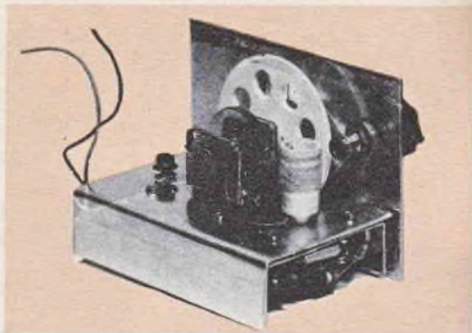
Veduta posteriore dell'oscillatore; per facilitare l'escursione delle gomme, al variabile è stata applicata una demoltiplica
