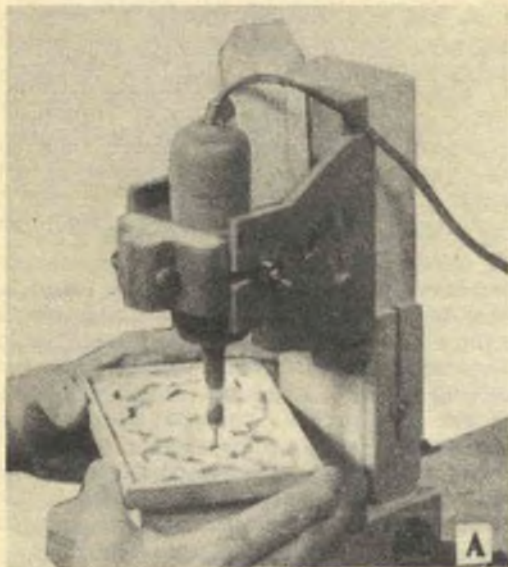
Con il motore montato su di una colonna il lavoro viene spostato comodamente sotto il ferro tagliente, per lavoro di bassorilievo a profondità costante delle incisioni. L'eventuale pulsante dell'interruttore generale dell'apparecchio viene tenuto premuto dalla legatura.
