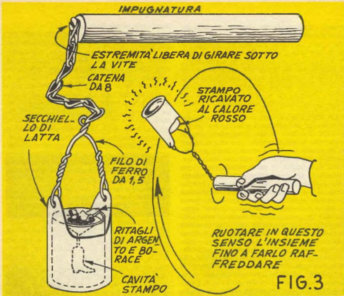
A sinistra ed in alto, il sistema al coperto, pronto per la colata; a destra veduta del complesso durante la rotazione veloce di esso, per costringere il metallo fuso a penetrare nel vano dello stampo per forza centrifuga.
