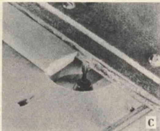
Così possono eseguirsi delle scanalature lungo linee diritte, case per caso, il ferro tagliente più adatto; il lavoro viene fatto scorrere lungo la costola diritta della guida; come si nota il motore viene tenuto in posizione capovolta.
