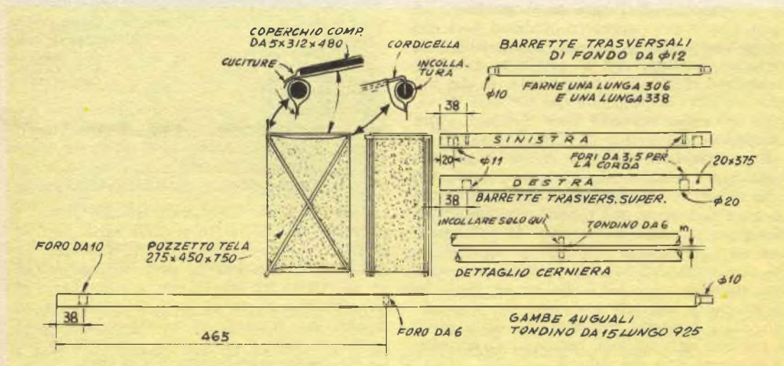
Il portabiancheria nella sua condizione normale, ossia mentre è in uso
