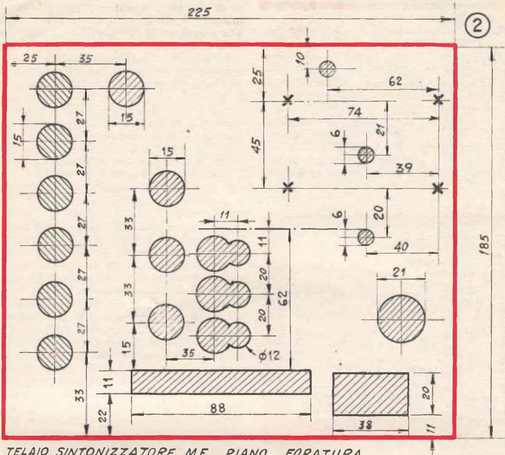
TELAIO SINTONIZZATORE MF. PIANO FORATURA
