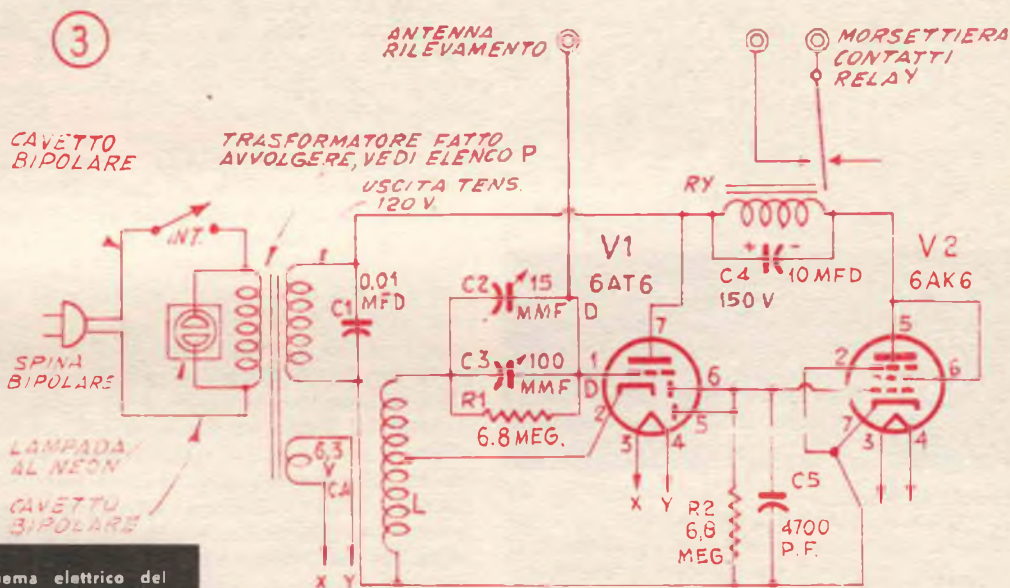
Schema elettrico del complesso
