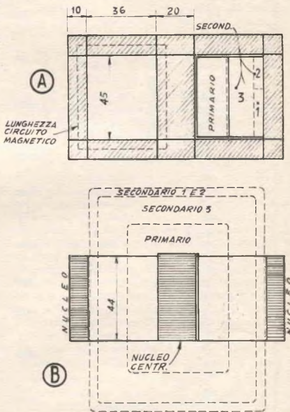
Nel tratteggio, la forma del circuito magnetico di un convenzionale trasformatore di alimentazione; in «A», veduta dall'alto; in «B», veduta della sezione orizzontale, in entrambe indicazione della posizione dei vari avvolgimenti
