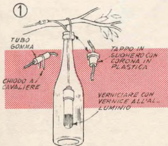
LANTERNA DA UNA BOTTIGLIA COMUNE
