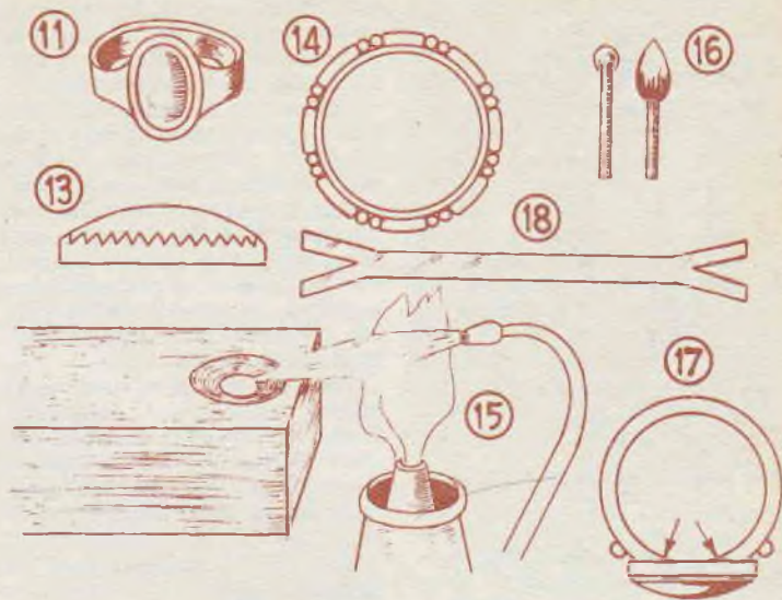
(11) Dettagli basilari dell'anello. (12) Montatura della pietra con sistema di griffa dentellata. (13) Montatura decorata con un cerchietto di filo a sezione non uniforme. (14) Sistema da adottare per preparare dei globetti di argento, la massa scura è un blocchetto di carbone vegetale. (15) A sinistra una sferetta saldata in cima ad un pezzetto di filo; a destra, la stessa appiattita ed intagliata. (16) Veduta dall'alto dell'anello. (17) Elemento di partenza per la realizzazione del cerchietto dell'anello
