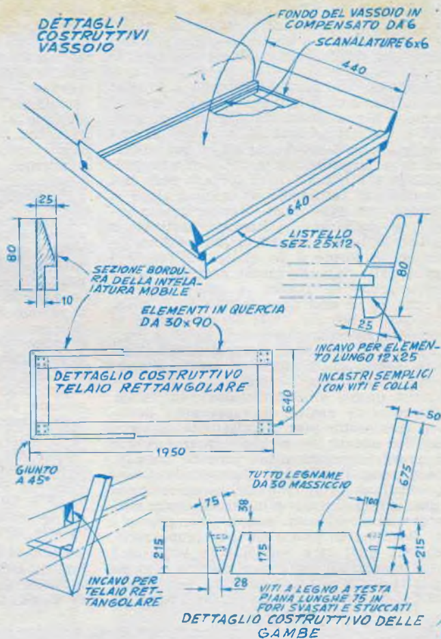
Dettagli costruttivi di molti degli elementi del mobile, ivi compreso il telaio, le zampe, del vassoio, ecc.
