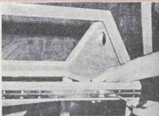
Messa a dimora della cerniera che unisce il coperchio al corpo del terrario; le viti, inossidabili da usare debbono essere di lunghezza sufficiente per fare bene presa nel legno, senza giungere a sporgere dalla parte interna del terrario
