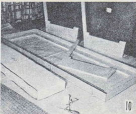
(Foto a sinistra): Qui è illustrata la fase successiva, ossia quella della applicazione dei listelli di bordura: l'insieme viene tenuto stretto, con morsetti apposti, mentre la colla fa presa. — (Foto a destra): Le tre zampe del mobile, formate ciascuna di tre elementi per fare sì che la venatura del legno abbia la direzione migliore per il massimo della resistenza. Tutto è pronto per la unione delle zampe al rettangolo superiore
