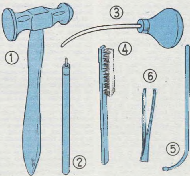
Nell'ordine, un martello con una testa plana ed una tonda; un punteruolo fatto con una puntina da gramofono piantata in cima ad una bacchetta di legno ed un brunitoio; uno spazzolino con setole di ottone; un cannello ferruminatorio, di tipo semplice, un paio di pinzette
