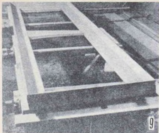
(Foto a sinistra): Qui è illustrata la fase successiva, ossia quella della applicazione dei listelli di bordura: l'insieme viene tenuto stretto, con morsetti apposti, mentre la colla fa presa. — (Foto a destra): Le tre zampe del mobile, formate ciascuna di tre elementi per fare sì che la venatura del legno abbia la direzione migliore per il massimo della resistenza. Tutto è pronto per la unione delle zampe al rettangolo superiore
