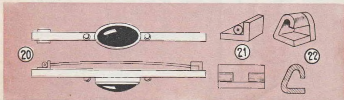
(20) Veduta di fronte e da un lato, di una spilla. (21) Veduta di fianco e dall'alto della cerniera della spilla di fig. 20. (22) Vedute del gancetto di bloccaggio per la spilla della fig. 20.
