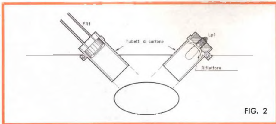
In basso: pista per il robot e schema della disposizione delle parti principali. Sopra: montaggio delle lampadine e delle foto-resistenze.
