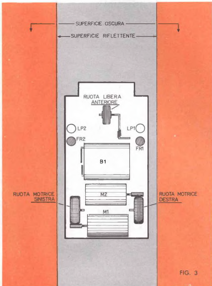
In basso: pista per il robot e schema della disposizione delle parti principali. Sopra: montaggio delle lampadine e delle foto-resistenze.
