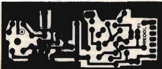
Lato componenti.
