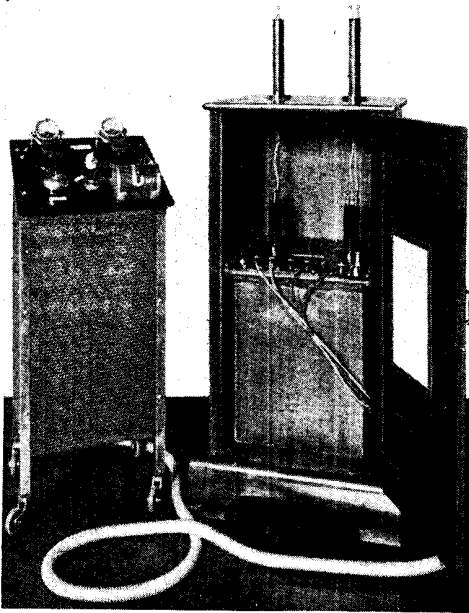
H.T. X-RAY APPARATUS
