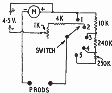
Fig. 3—Circuit for 5 range meter
