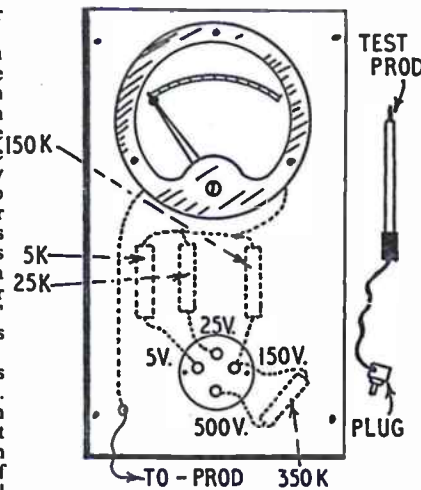
Fig. 4—A 4 range meter
