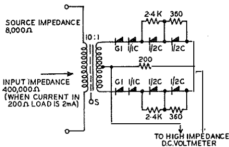
FIG. 5.—RECTIFIER CIRCUIT OF SPEECH ANALYSER.
