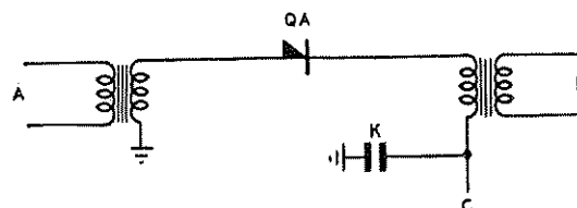
FIG. 7.—ELEMENT SWITCH USING A RECTIFIER.
