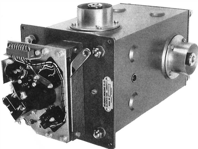
FIG. 2—30 kW COAXIAL SWITCH UNIT
