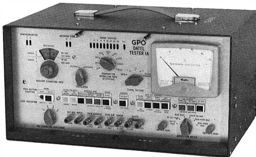
FIG. 2—DATTEL TESTER No. 1A
