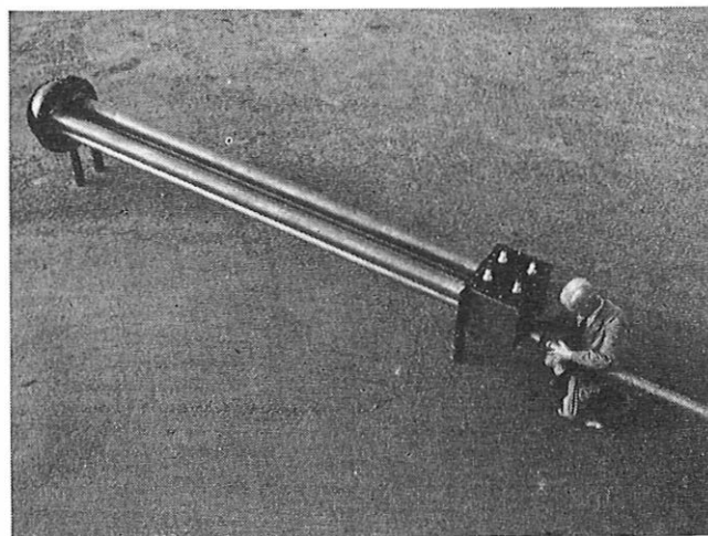
FIG. 8—A 75 kW BALUN
