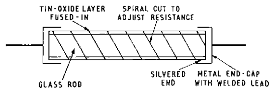
FIG. 2—METAL-OXIDE-FILM RESISTOR
