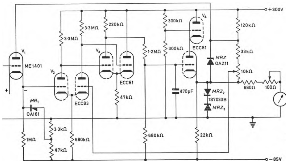
Fig. 4 Memory voltmeter circuit
